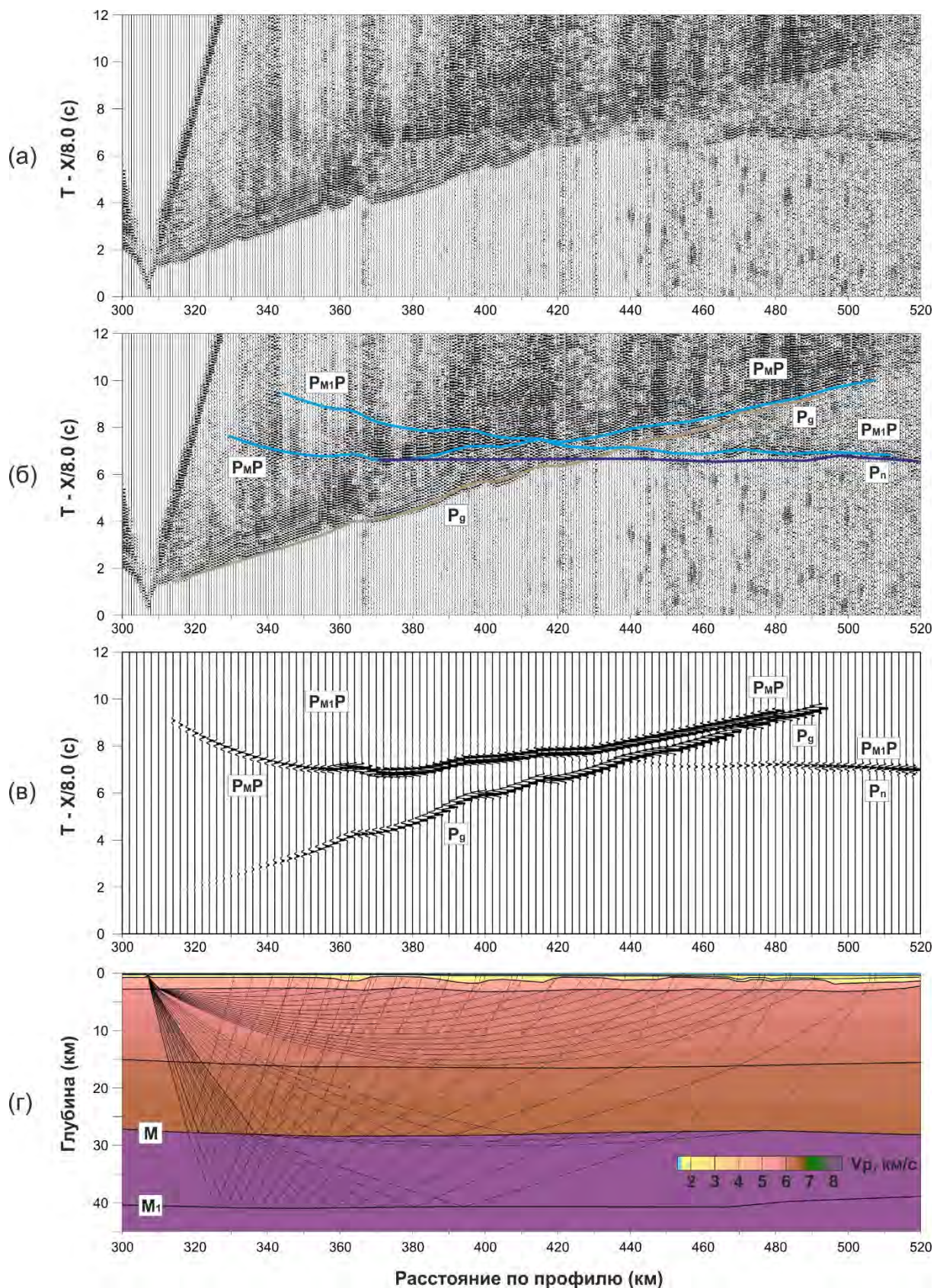
Рис. 3.5. Лучевое кинематическое и динамическое моделирование P-волн от внутри-мантийной границы (границы M_1 )
