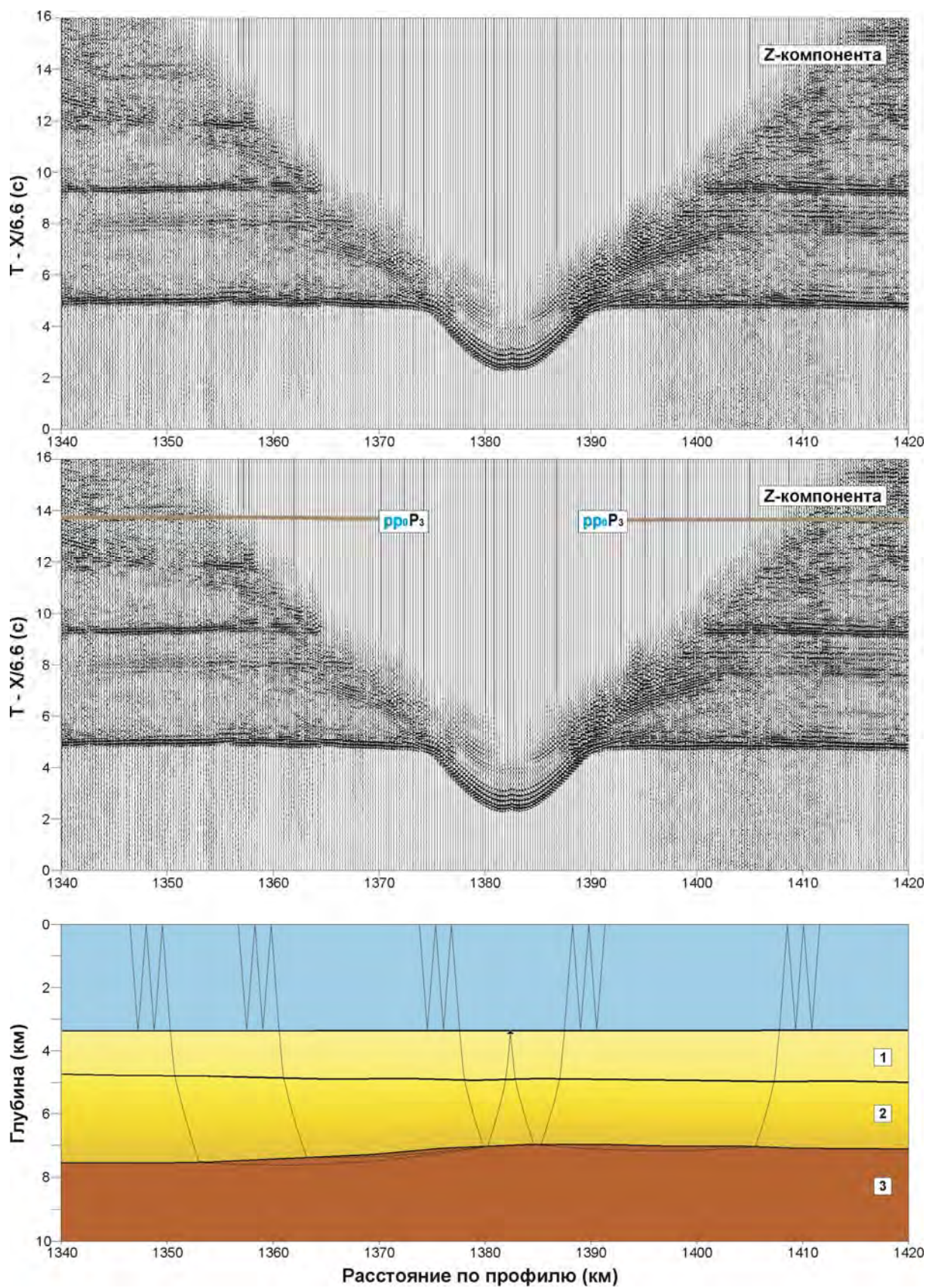
Рис. 9. Лучевое моделирование кратных волн, связанных с водным слоем, pp_0P_3 -волна (ПК 1382, модель_1)
