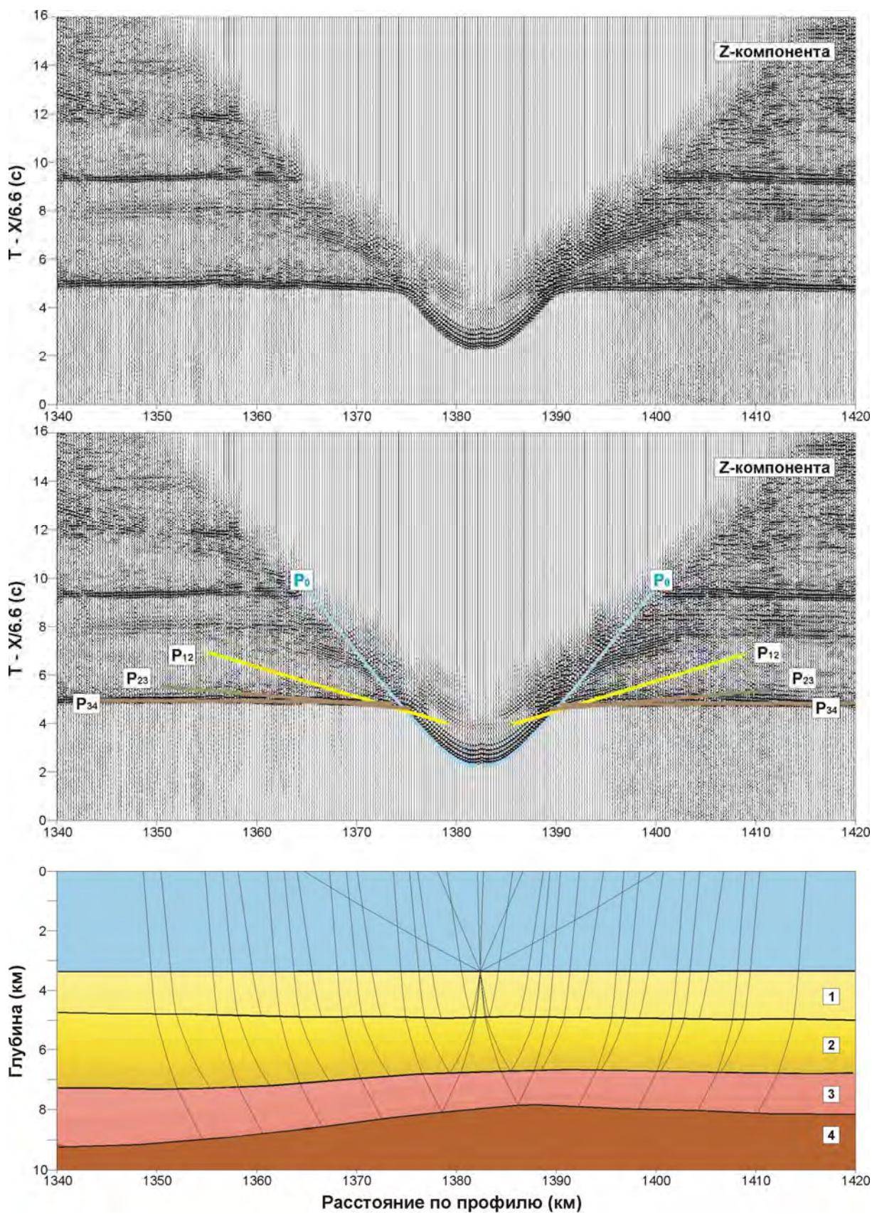
Рис. 6. Лучевое моделирование головных P-волн (ПК 1382, модель_2)
