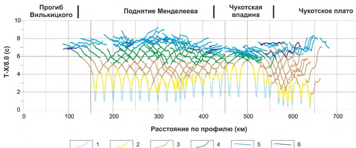
Рис. 3.17. Редуцированные годографы основных продольных волн, зарегистрированные на профиле ГСЗ Арктика-2012, приведенные к середине расстояний источник–приемник
