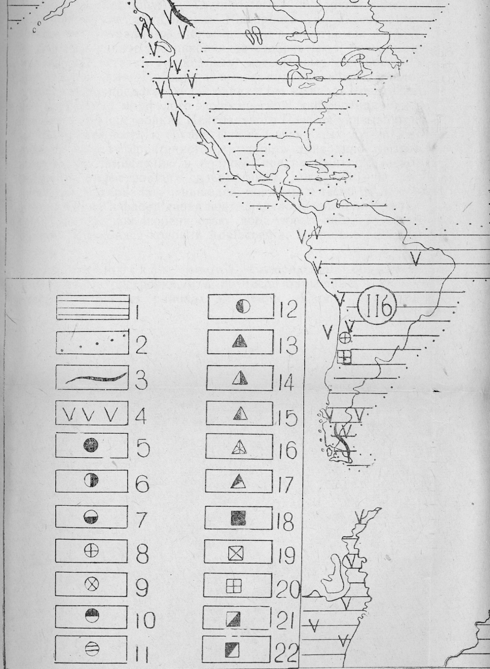
Рис. 3. Географическое распространение некоторых родов склерактиний и схема биогеоценоза. 5— Axosmilopsis , 6— Cyathocoenia , 7— Epismilopsis , 8— Lepidophyllia , 9— Octocoenia , 10— Cyathus , 11— Cyathophyllia , 12— Eliphillum , 13— Thamnasteria , 14— Thecoseris , 15— Gymnastrea , 16— Halysma , 17— Cyathophyllia , 18— Eliphillum , 19— Thamnasteria , 20— Thecoseris , 21— Gymnastrea , 22— Halysma . Гималайская провинция, 1в—Мадагаскарская провинция.
