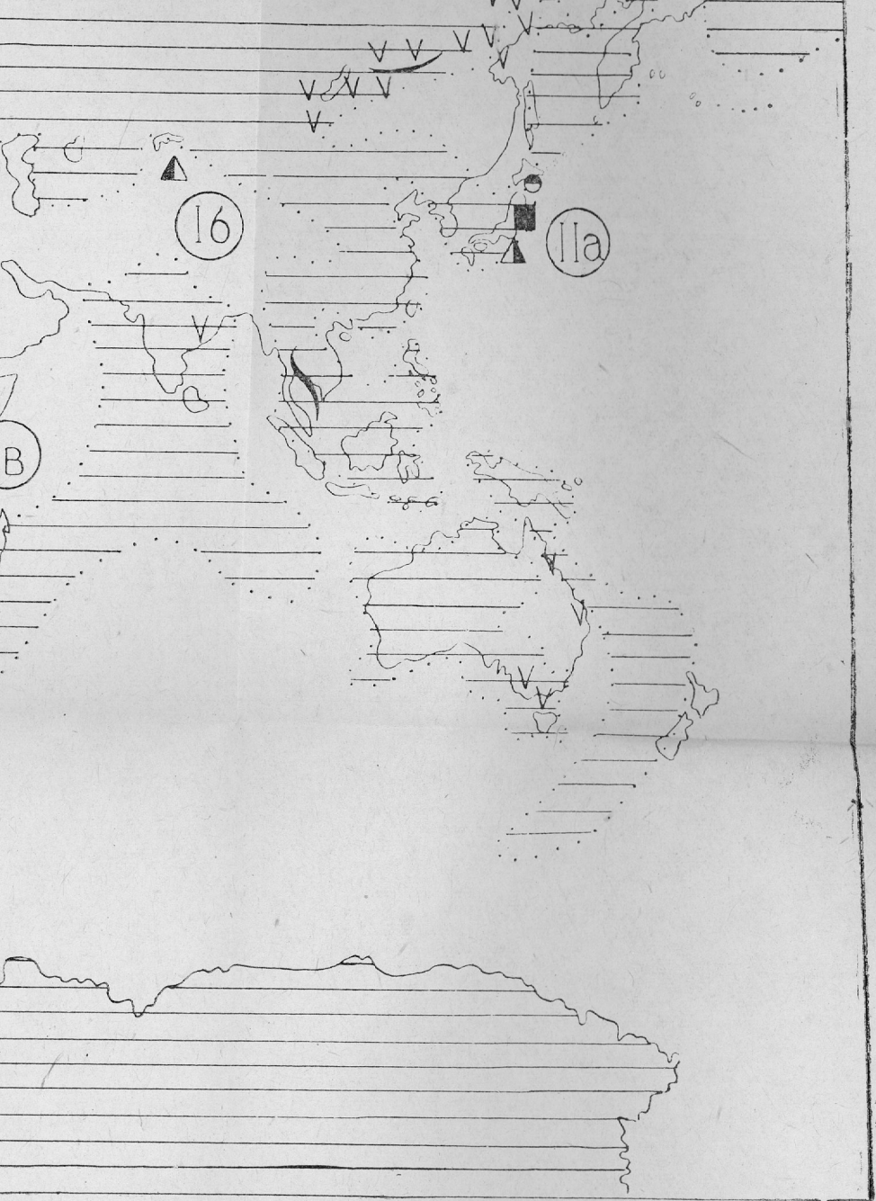
бассейнов. 1 — суша, 2 — морские бассейны, 3 — горы, 4 — действующие вулканы, 12 — Stephanosoenia, 13 — Ellipsoidastraea, 14 — Isastraea, 15 — Montlivaltia, 16 — Theo- ническое районирование: Тетическая область: Ia — Европейская провинция, Ib — Памиро- а провинция, IIb — Южно-Американская провинция.
