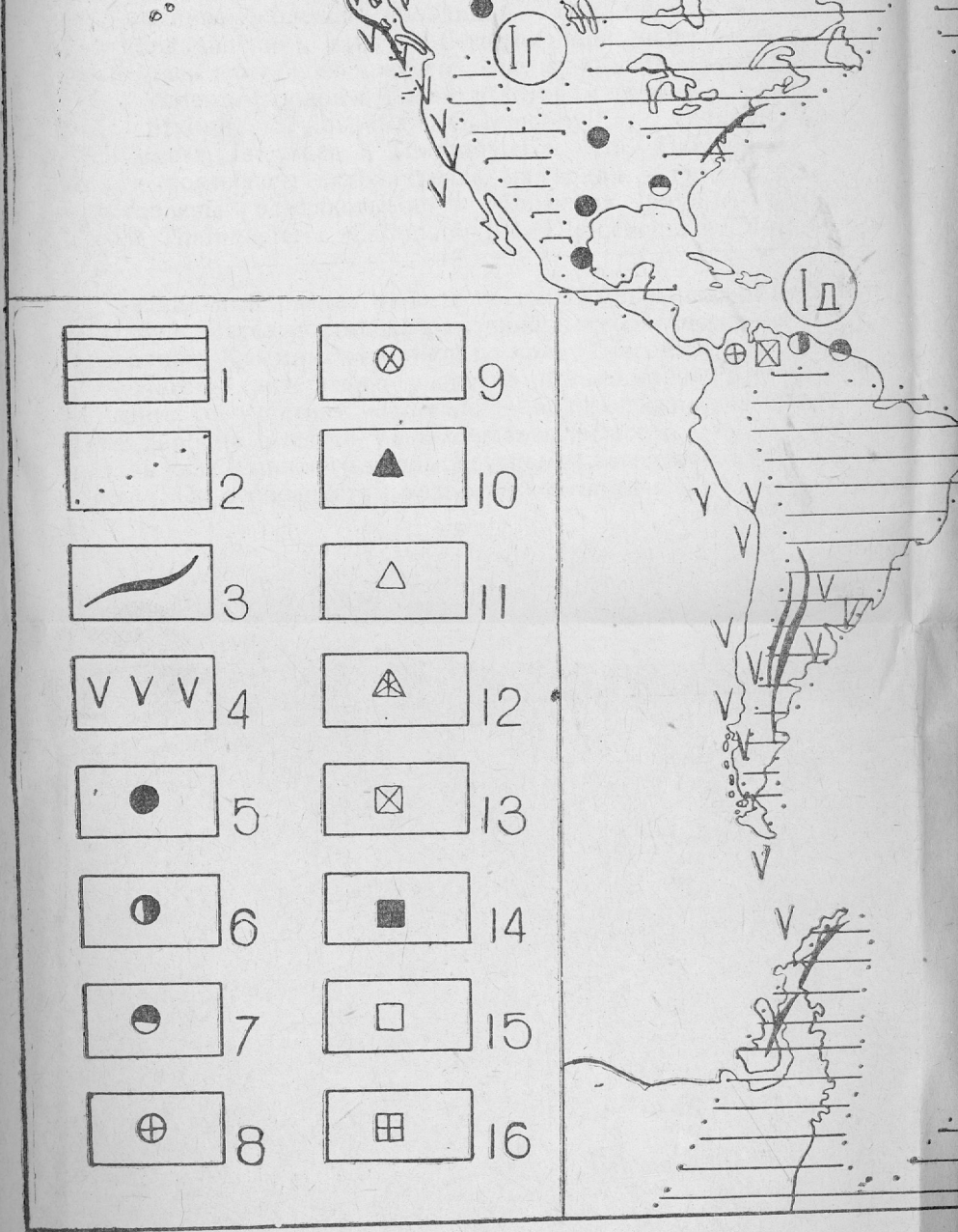
Рис. 4. Географическое распространение некоторых родов склерактиний и схема биогоры, 4 — действующие вулканы, 5 — Actinastraea , 6 — Allocoenia , 7 — Stylina , 8 — Etallonia , 16 — Summigaea . Биогеографическое районирование: Тетическая область ская провинция, Iд — Венесуэло-Колумбийская провинция; II — Тихоокеанская об.
