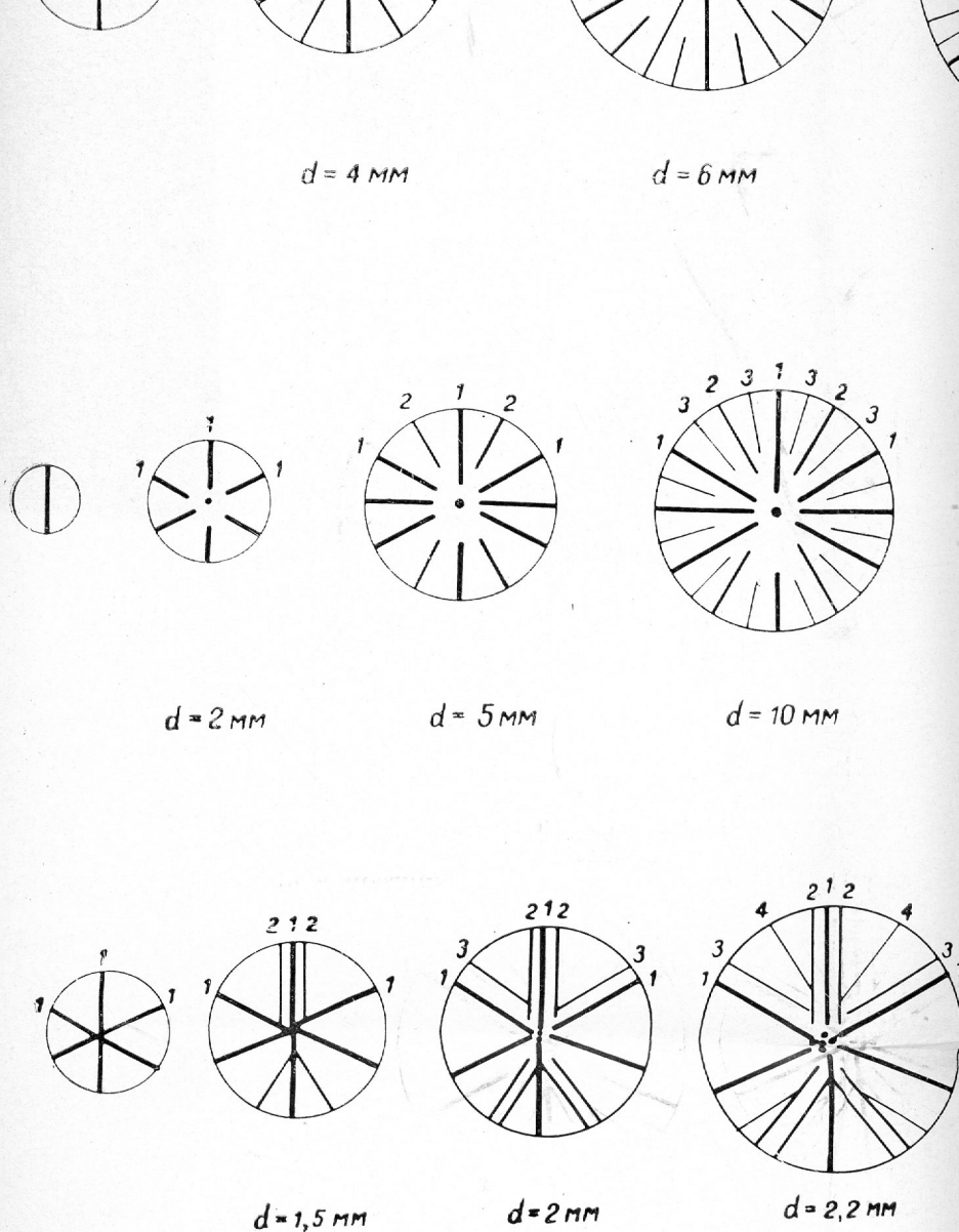
Рис. 1. Схемы онтогенезов септального аппарата у некоторых тонких склерактиний Крыма.
