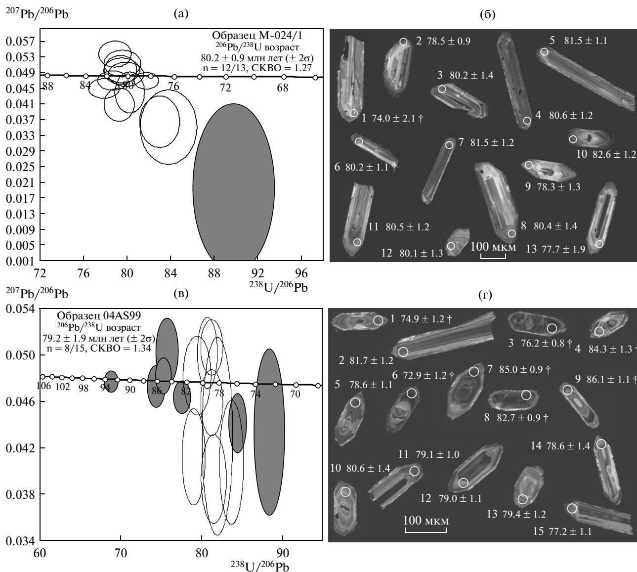
Рис. 4. Диаграммы Тера-Вассербурга (а, в) и катодолуминесцентные изображения цирконов (б, г) для образцов М-024/1 (а, б) и 04AS99 (в, г).
