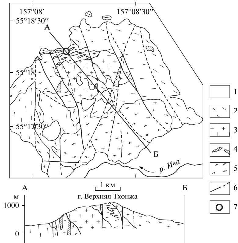
Рис. 3. Геологическая карта массива г. Верхняя Тхонжа (Шаповаленко, 1994), с изменениями.
