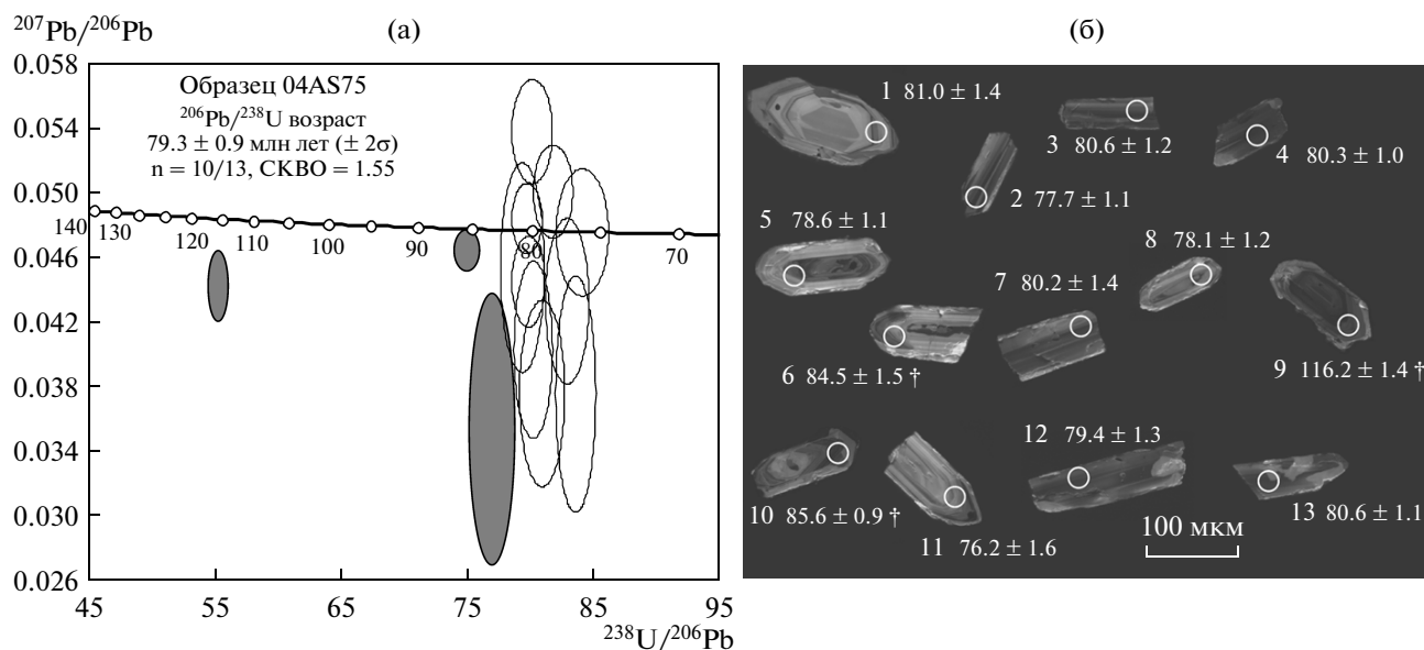
Рис. 5. Диаграмма Тера-Вассербурга (а) и катодоллюминесцентные изображения цирконов (б) для образца 04AS75.
