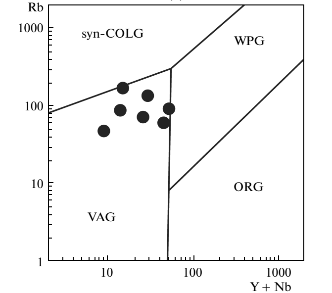
Рис. 10. Диаграммы (а) Zr - 10^4 Ga/Al (Whalen et al., 1987) и (б) Rb - (Y + Nb) (Pearce et al., 1984) для кампанских гранитоидов Малкинского поднятия Срединного хребта. (б): типы гранитов: syn-COLG – синколлизионные, VAG – вулканических дуг, WPG – внутриплитные, ORG – океанических хребтов.
