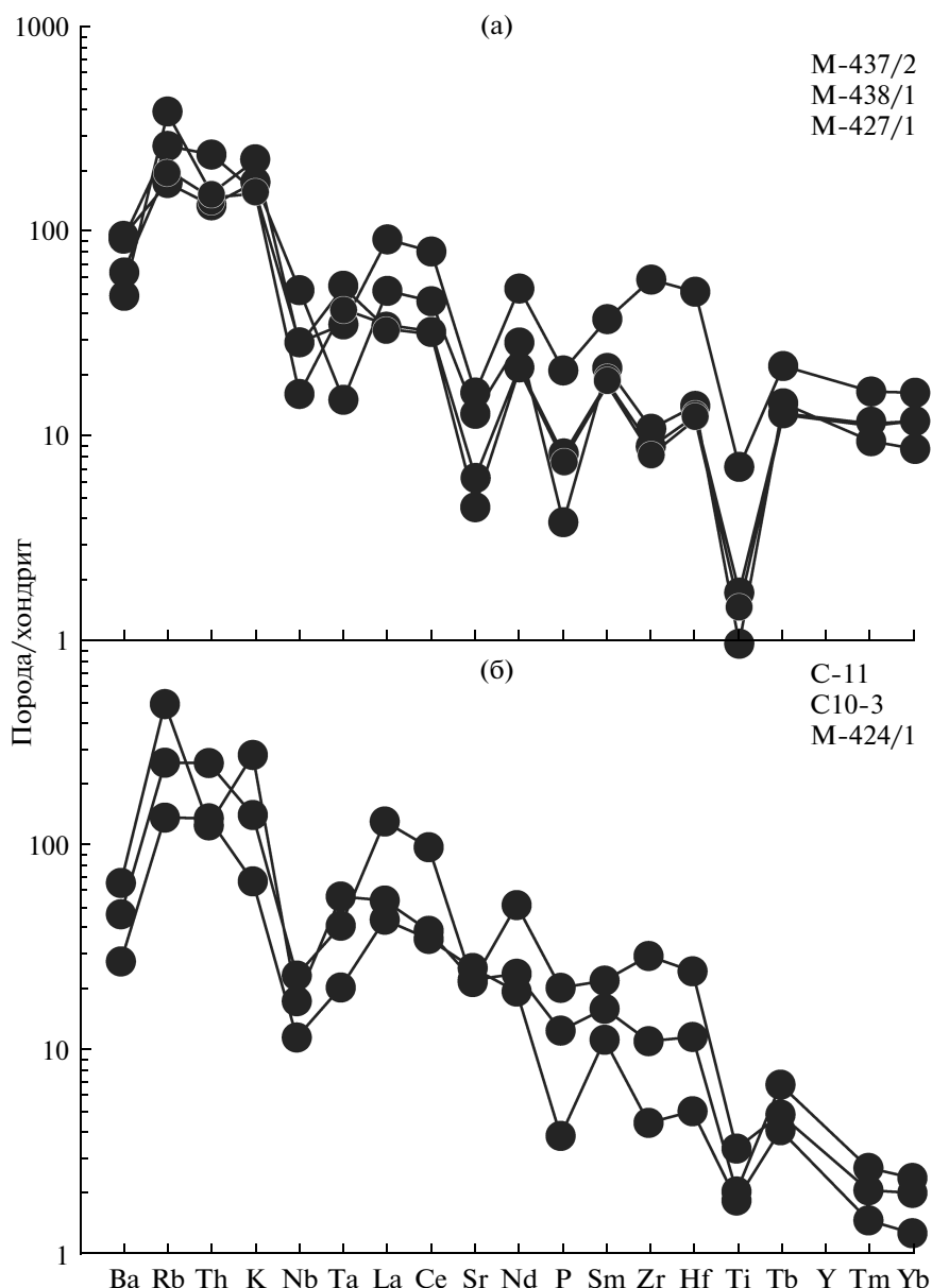
Рис. 12. Спайдер-диаграммы нормированных на состав хондрита (Sun, Donough, 1989) элементов-примесей в камчатских гранитоидах.
