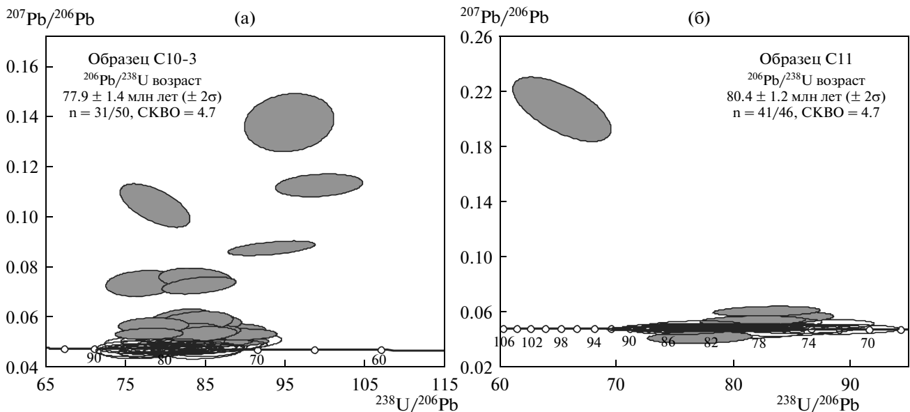
Рис. 6. Диаграммы с конкордией для образцов С10-3 (а) и С-11 (б).
