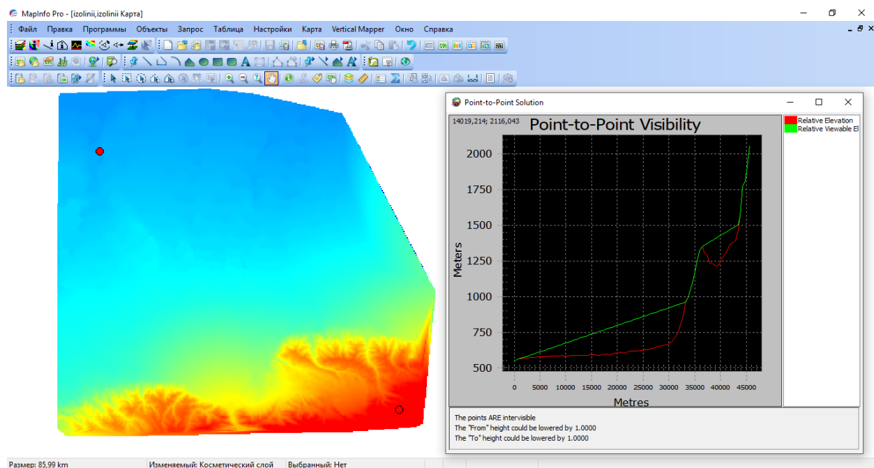
Рисунок 4.24 – 2-D модель рельефа прощадии Талгарского МПВ, профиль рельефа
