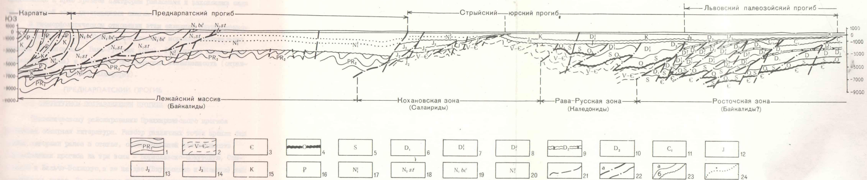
РИС.5. СХЕМАТИЧЕСКИЙ ГЕОЛОГИЧЕСКИЙ ПРОФИЛЬ ЧЕРЕЗ ПРЕДКАРПАТЬЕ И ВОЛЫНЬ
