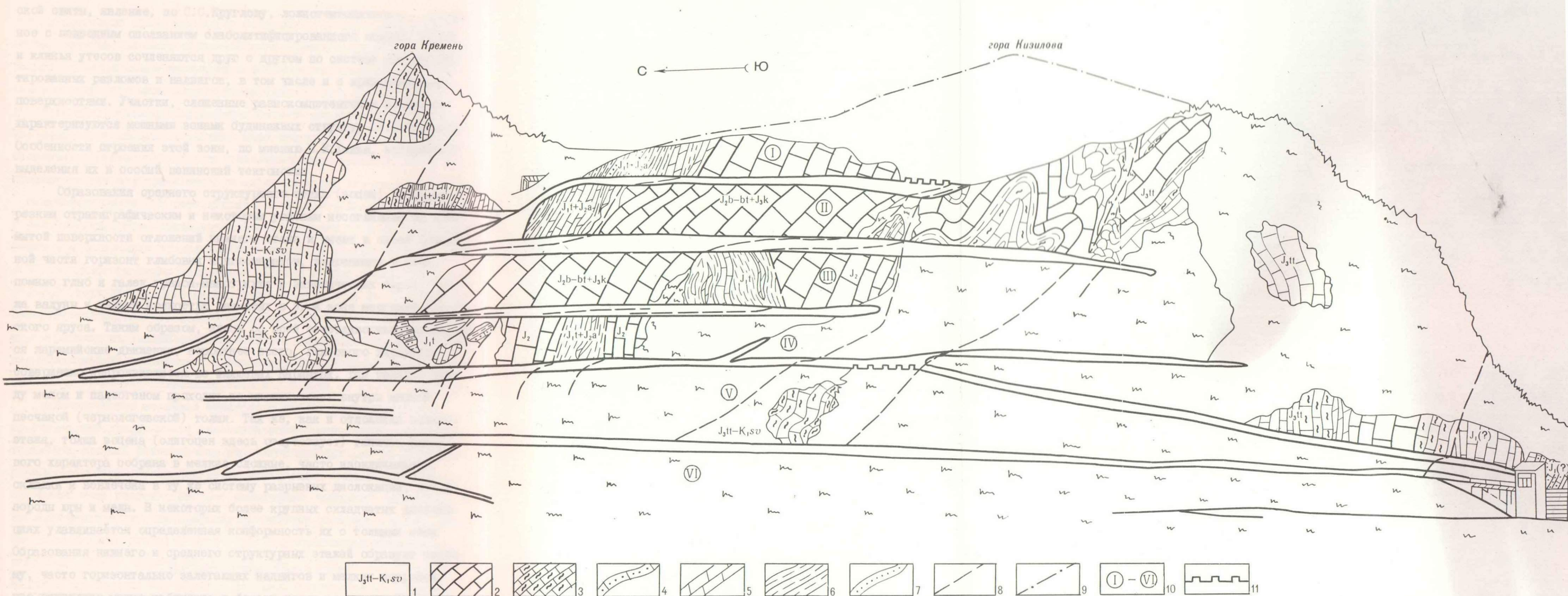
РИС.7. ЗАРИСОВКА КАРЬЕРА С.ПРИБОРЖАВСКОЕ В ЗОНЕ ПЕНИНСКИХ УТЕСОВ (по состоянию работ на 1964 год)
