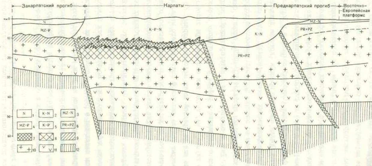
Рис.8. Схема глубинного строения Украинских Карпат
