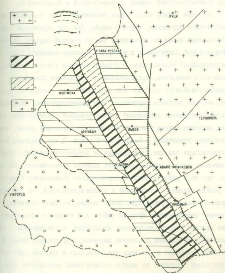
Рис. 4. Тектоническая схема фундамента Предкарпатья.
