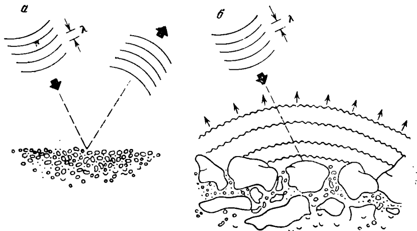
Рис. 37. Отражение радиолокационных сигналов различными поверхностями
