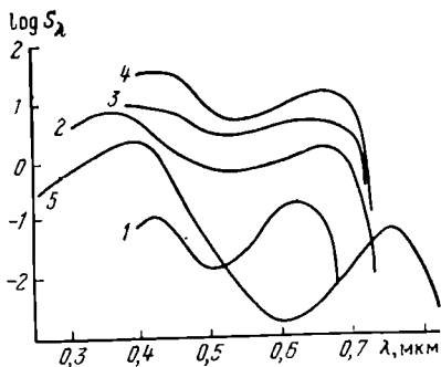
Рис. 14. Кривые спектральной чувствительности основных сортов аэропленок:
