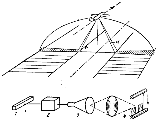
Рис. 36. Принцип действия радиолокационной станции бокового обзора:
