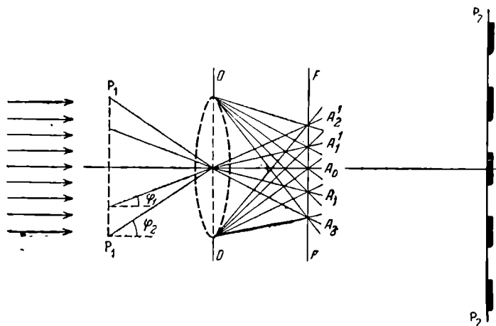
Рис. 32. К дифракционной теории фильтрации
