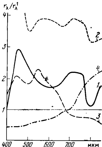
Рис. 5. Кривые отношений спектральных коэффициентов яркостей некоторых сочетаний растительности:
