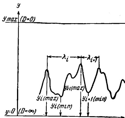
Рис. 28. Элементы регистрограммы
