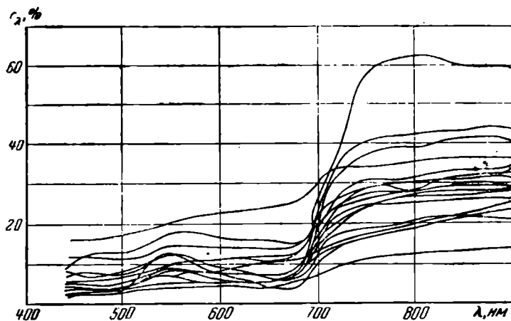
Рис. 11. Кривые СКЯ объектов 2-ой группы
