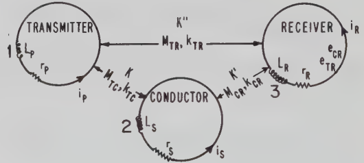
Figure 7.6. Electric-circuit analogy for EM system.
