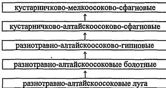
Рисунок 6. Схема сукцессий растительного покрова большинства болот хребта Ергаки.
