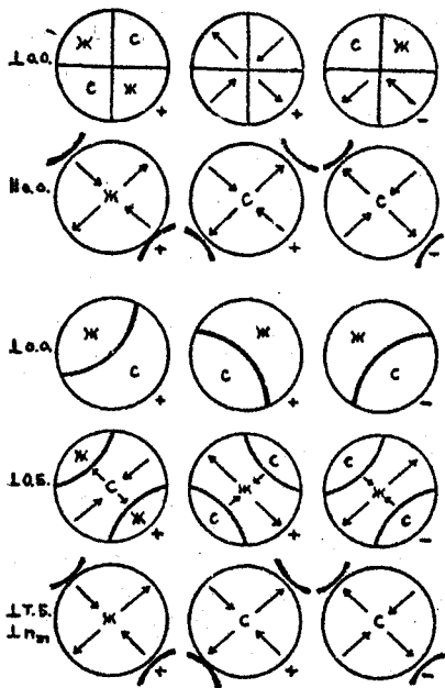
Рис. 1. Схемы определения опности и оптического знака одноосных (вверху) и двuosных (внизу) кристаллов по коноскопическим фигурам с помощью гипсовой пластинки (С - прямая параллельность, Ж - обратная) и кварцевого клина (стрелки показывают направление движения полосок при движении клина).
