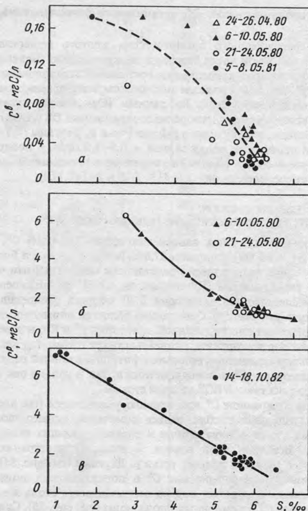
Рис. 56. Концентрация взвешенных ( a ) и растворенных ( б , в ) "окрашенных" веществ в поверхностных водах Рижского залива в зависимости от солёности (Юрковский, Ругайне, 1986)
