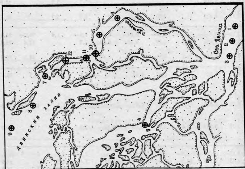
Рис. 9. Местоположение станций отбора проб в устье р. Печоры (июль 1980)
