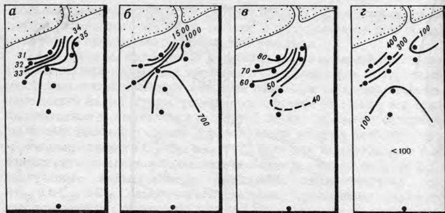
Рис. 75. Распределение солености (в ‰) (а), взвеси (в мкг/л) (б), биомассы планктона (в мг/м 3 ) (в) и C^B (в мкг/л) (г) в водах Мозамбикского пролива, прилегающих к устью р. Лимпопо (Артемьев, 1982)
