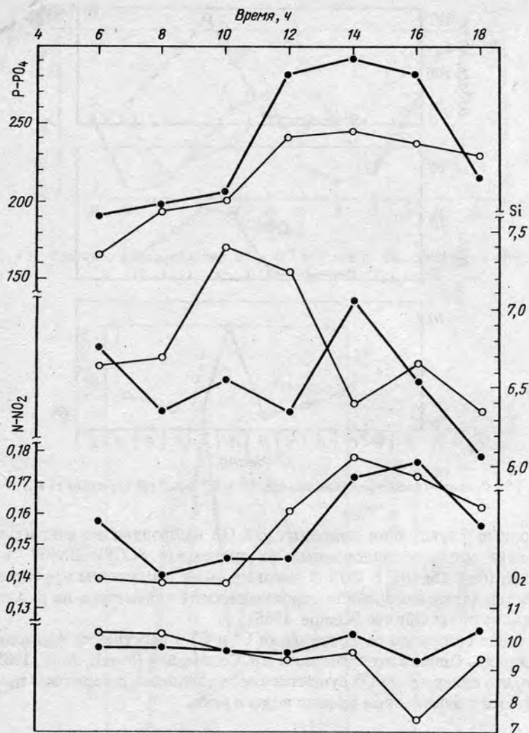
Рис. 20. Изменение концентраций биогенных элементов, взвеси, P^P , S^B и микроэлементов (в мг/л) в устье р. Дон в течение суток (октябрь 1980)
