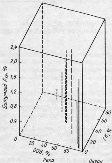
Рис. 70. Преобразование состава ОВ взвеси и донных осадков в системе река-эстуарий-океан
