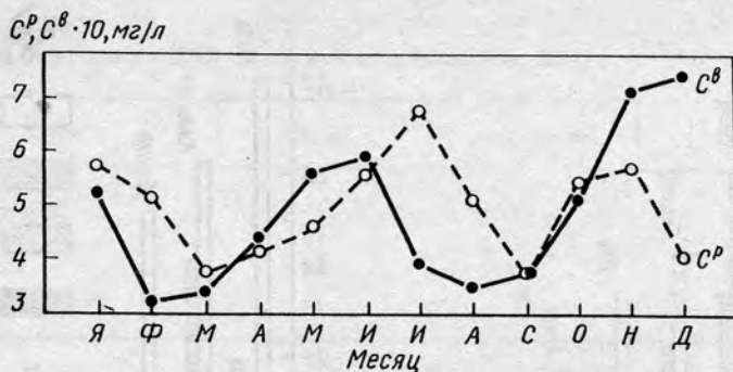
Рис. 17. Сезонное распределение C^P и C^B в устье р. Св. Лаврентия (Pocklington, 1985)
