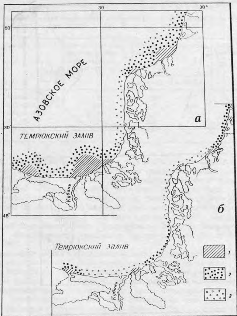
Рис. 47. Распределение речной и морской воды в системе устье р. Кубань—море при юго-восточном (а) и северо-западном (б) ветрах
