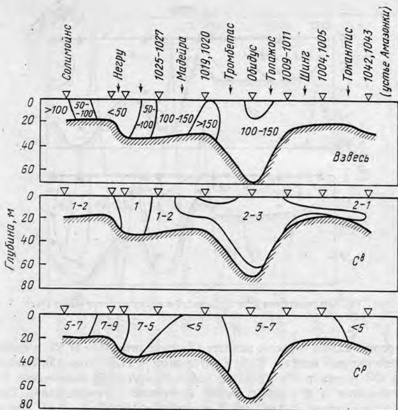
Рис. 11. Распределение взвеси, C^P и C^B (в мг/л) в бассейне р. Амазонки от устья р. Солимоинс до устья р. Амазонки (март-апрель 1983)
