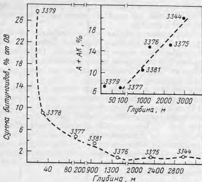
Рис. 80. Изменение битуминозности ОВ поверхностного слоя донных осадков на разрезе устья р. Замбези-океан (Данюшевская, Романкевич, 1987)
