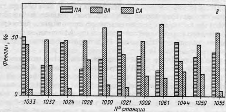
Рис. 24. Соотношение фенолов во взвеси (а) и в донных осадках (в) и содержание производных лигнина (фенолов) C_f в ВОВ (б), в донных осадках (г) и в ОВ донных осадков (д) бассейна р. Амазонки и ее эстуария
