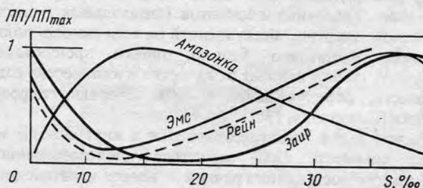
Рис. 45. Зависимость отношения \text{PP}/\text{PP}_{\text{max}} от солености в эстуариях (Eisma, 1988; Cadée, 1982)
