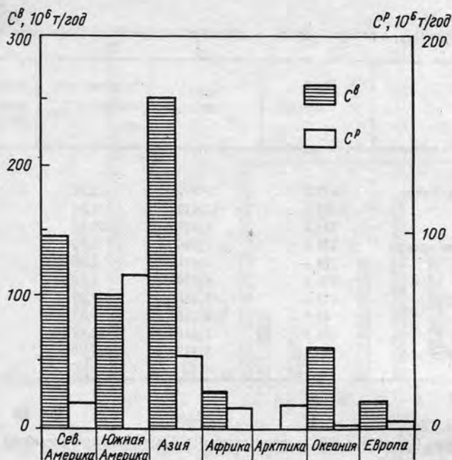
Рис. 6. Ежегодный сток речного C_{\text{орг}} с континентов в океан (Degens et al., 1984; Degens, Ittekkot, 1985)
