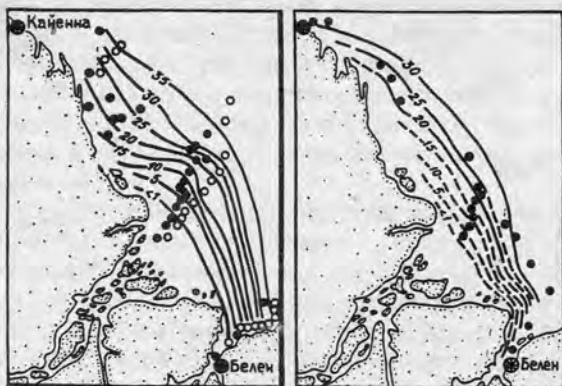
Рис. 33. Распределение солености (в ‰) на поверхности вод в эстуарии р. Амазонки в сезоны высокой (а) и низкой (б) воды (Монин и др., 1986)
