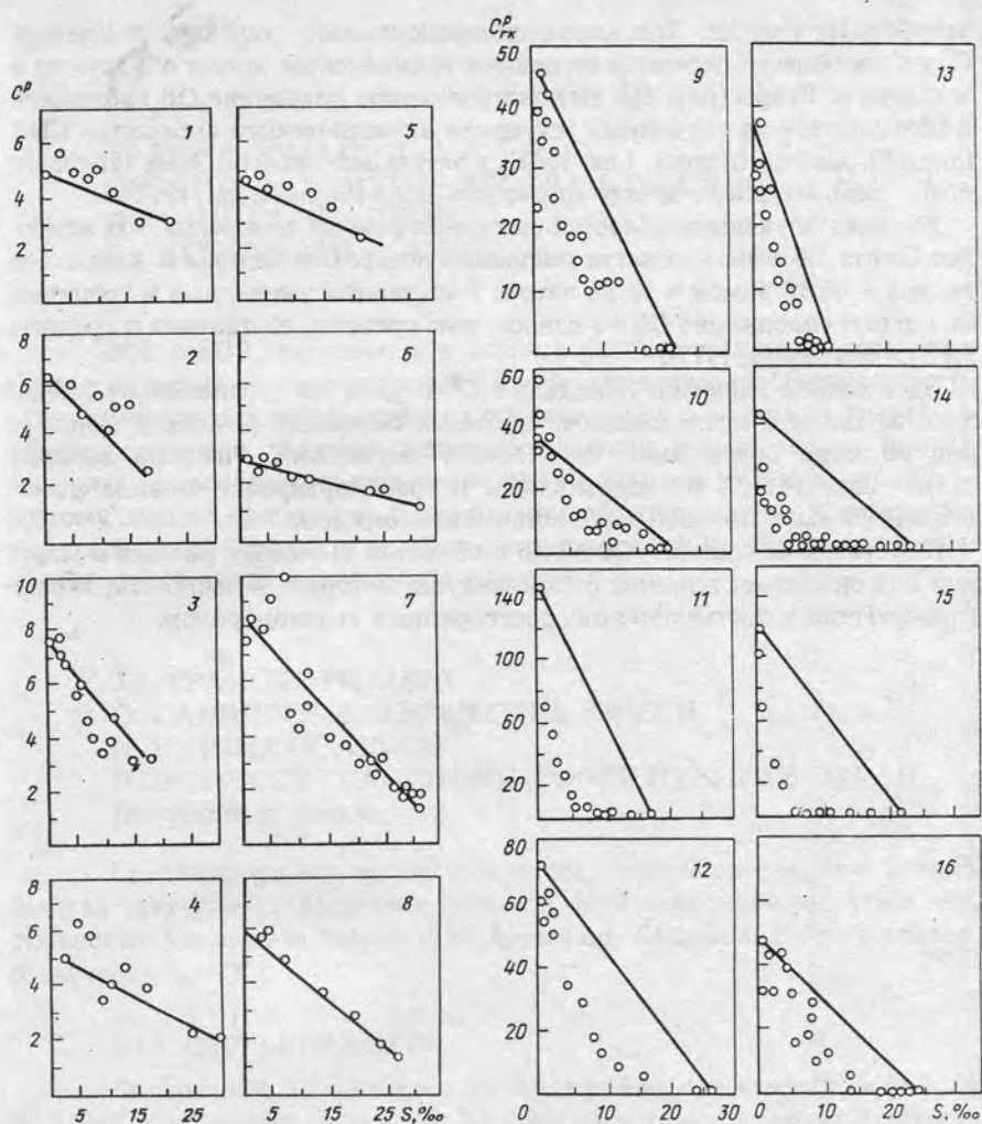
Рис. 67. Распределение C^P и C^P_K в эстуариях (Фох, 1983)
