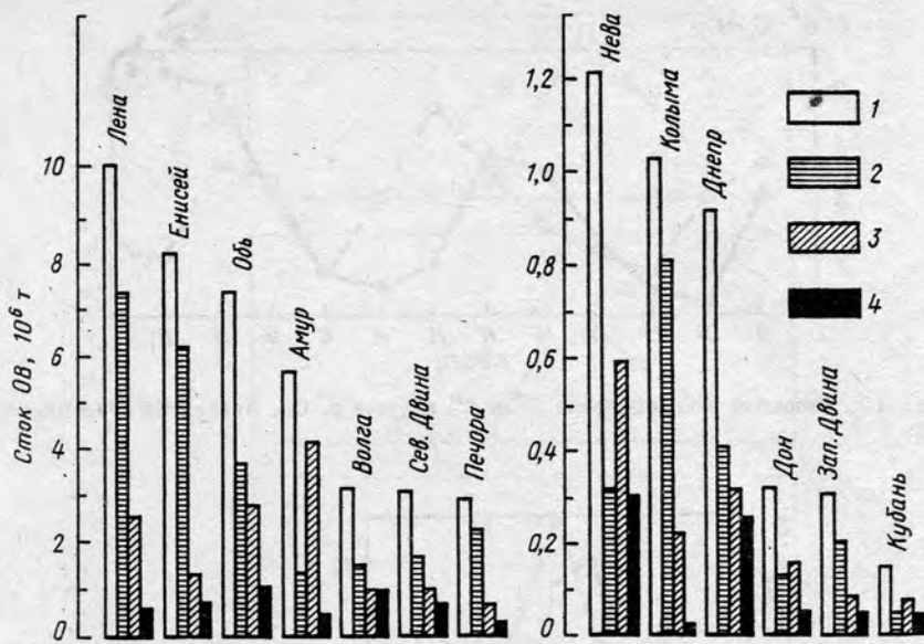
Рис. 15. Сезонное распределение стока ОБ из некоторых крупных рек бывш. СССР по сезонам года
