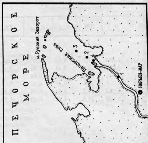
Рис. 8. Местоположение станций отбора проб в устье р. Сев. Двины и южной части Двинского залива (1980-1987)
