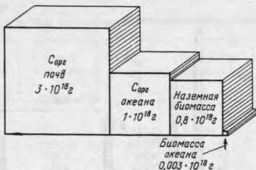
Рис. 2. Содержание C_{org} на континентах и в океане (Degens et al., 1984; Romankevich, 1990)
