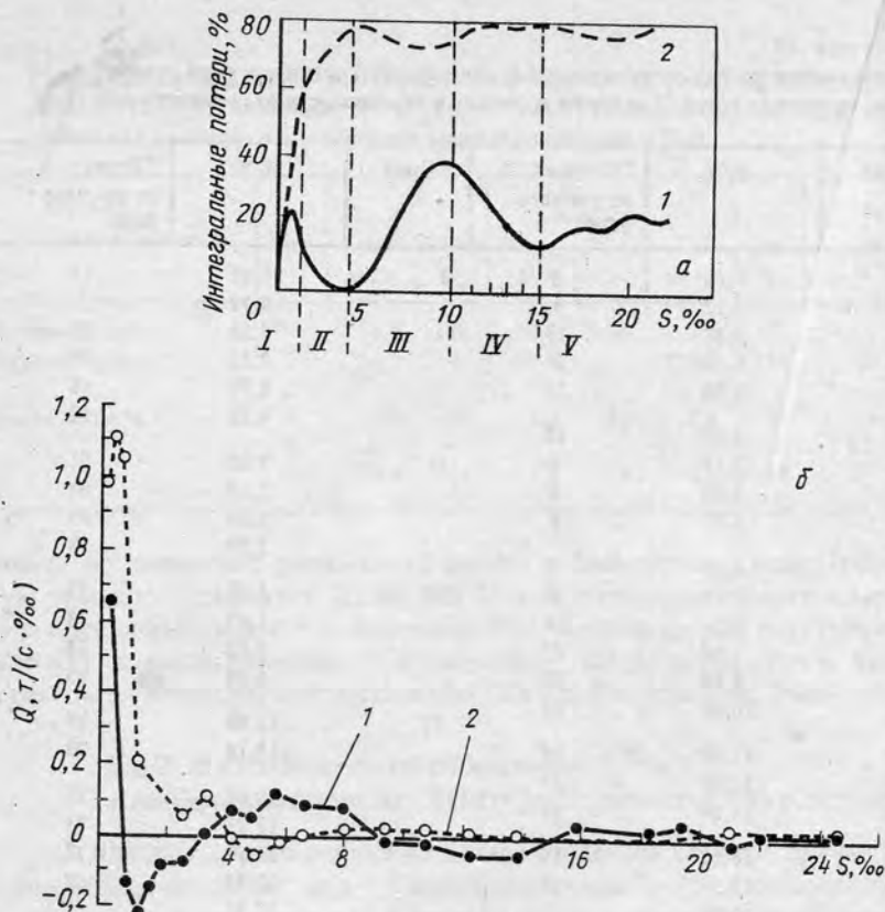
Рис. 41. Интегральные "потери" (а) и интенсивность дифференциальных "потерь" Q (б) речного РОВ (1) и ВОВ (2) в процессе перемешивания вод р. Амазонки и океана (Артемьев, Шапиро, 1987)
