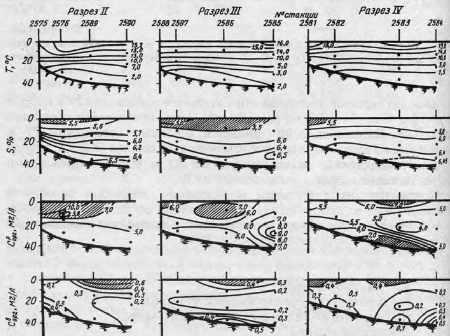
Рис. 54. Вертикальное распределение температуры, солёности, C^P и C^B на разрезах река-море в южной части Рижского залива в июле 1978 г. (Артемьев и др., 1981) См. рис. 53.
