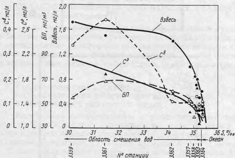
Рис. 76. Зависимость концентрации взвеси, биомассы планктона (БП), C^P и C^B от солености на периферии области смешения вод р. Лимпопо—океан (Артемьев, 1982)
