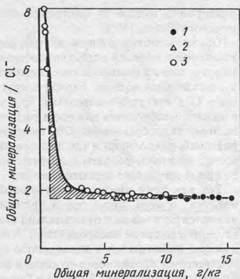
Рис. 27. Соотношение между общей минерализацией и отношением ее к хлору в Азовском море (Цурикова, Шульгина, 1964)
