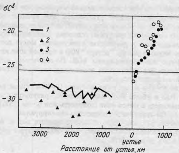
Рис. 44. Изменение \delta^{13}\text{C} в водах бассейна р. Амазонки и ее эстуария (Cai et al., 1988)
