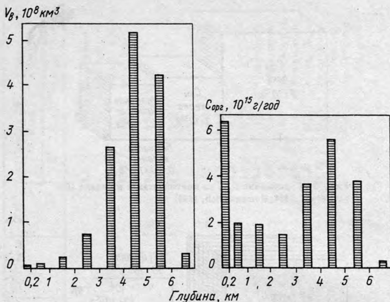
Рис. 4. Объемы воды и количество C_{орг} , образующегося в водах над различными глубинами дна океана (Degens, Ittekkot, 1983)
