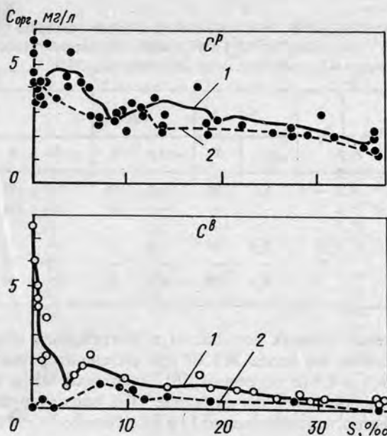
Рис. 40. Зависимость концентраций C^P и C^B от солёности в эстуарии р. Амазонки (Артемьев, Шапиро, 1987)
