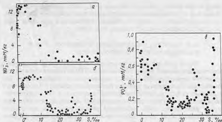
Рис. 39. Зависимость содержания нитратов (а, б) и фосфатов (е) от солёности в эстуарии р. Амазонки по данным экспедиции ИО АН СССР в 1983 г. (а) и по данным Edmond et al., 1981 (б, е)
