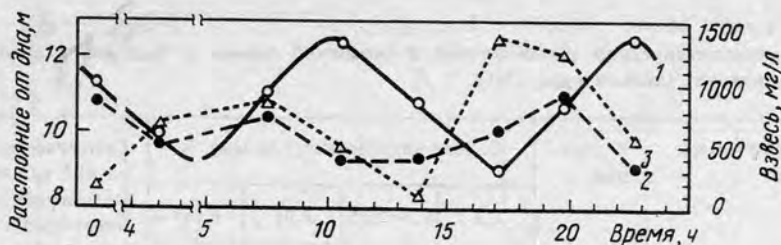
Рис. 37. Суточные изменения концентраций взвеси в эстуарии р. Амазонки (Гордеев и др., 1988)
