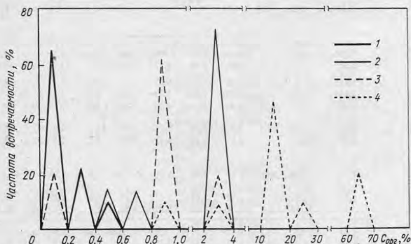
Рис. 14. Содержание C_{\text{орг}} в почвах, взвеси и донных осадках бассейна р. Амазонки (март–апрель 1983)
