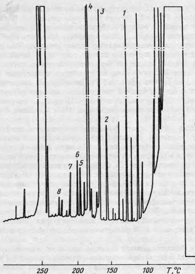
Рис. 23. Хроматограмма продуктов щелочно-нитробензольного окисления ОБ донных осадков из устья р. Сев. Двины (Пересыпкин и др., 1989) 1 — БК; 2 — ПА; 3 — ПАФ; 4 — ВА; 5 — ПК; 6 — СА; 7 — ВК; 8 — СК
