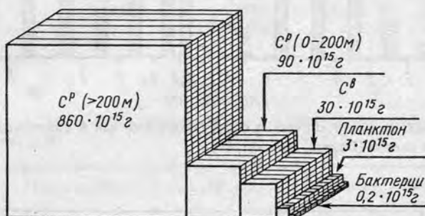
Рис. 3. Распределение C_{org} в водах океана (Degens et al., 1984)
