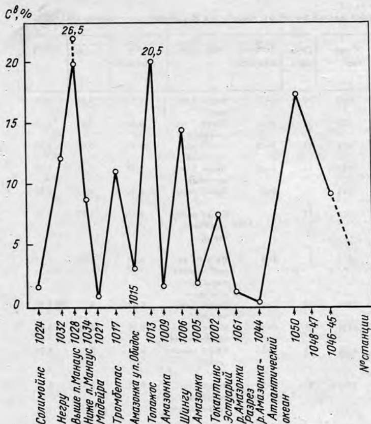
Рис. 13. Распределение C^B в бассейне и эстуарии р. Амазонки (март—апрель 1983)
