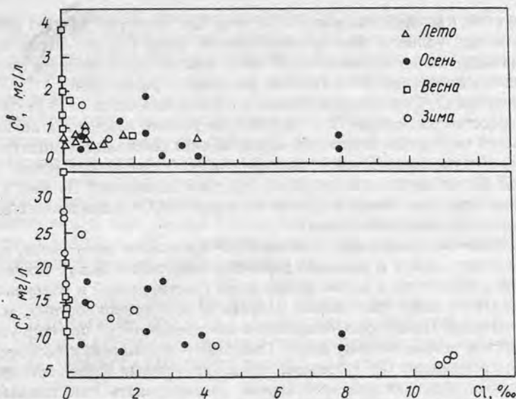
Рис. 63. Распределение C^P и C^B в области смешения вод р. Сев. Двины и моря в разные сезоны года в зависимости от хлорности (Артемьев, Лазарева, 1984; Artemyev, Romankevich, 1988)
