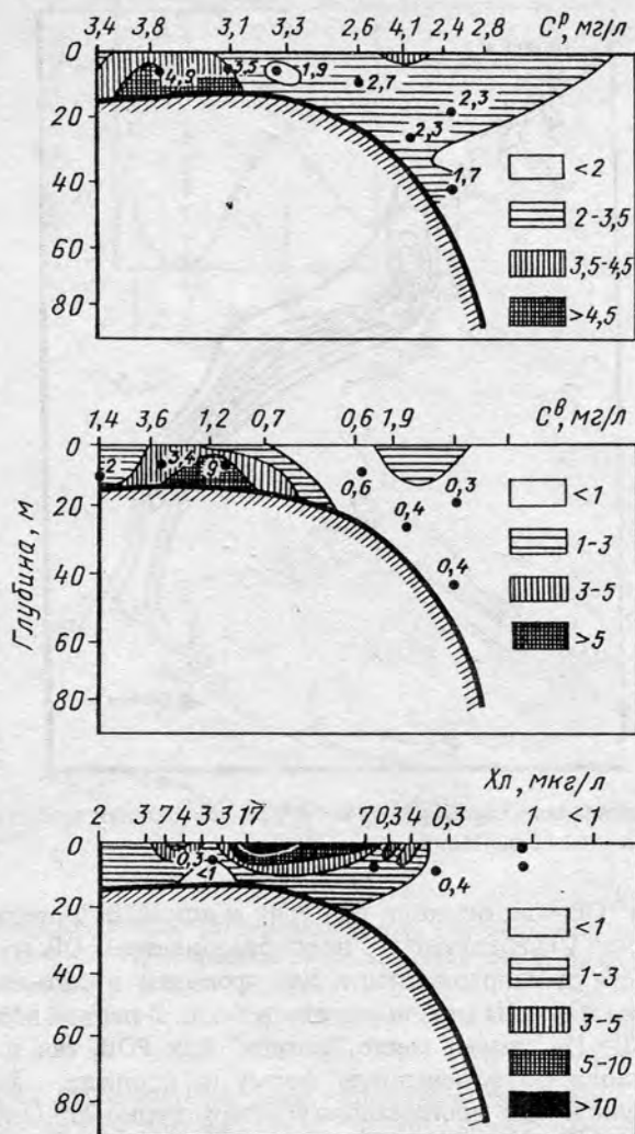
Рис. 43. Вертикальное распределение C^P , C^B и хлорофилла ( Xл ) на разрезе устья р. Амазонки—океан (Монин и др., 1986)
