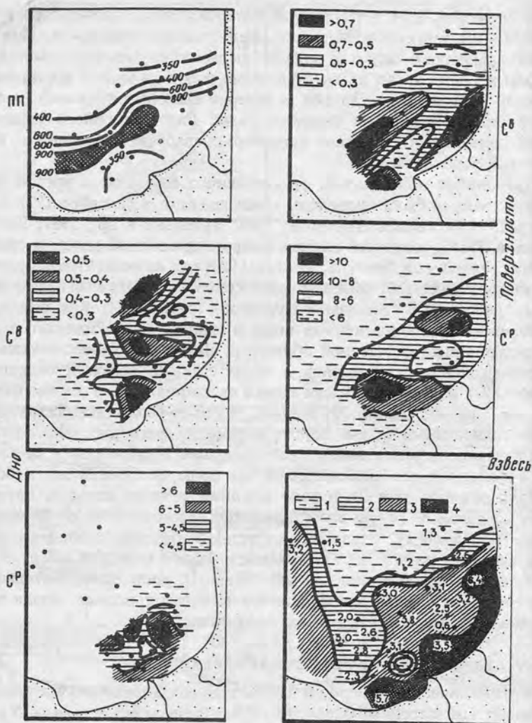
Рис. 55. Концентрация первичной продукции (в \text{мг С} / (\text{м}^3 \cdot \text{сут}) , \text{С}^{\text{В}} , \text{С}^{\text{Р}} и взвеси (в \text{мг/л} ) в поверхностном и придонном слоях вод южной части Рижского залива (Артемьев и др., 1981; Демина, Артемьев, 1984)
