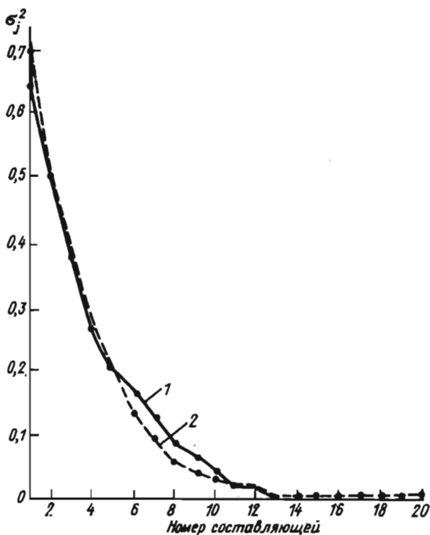
Рис. 4.1. Распределение относительных погрешностей аппроксимации пористости (1) и содержания \text{CaCO}_3 (2) в отложениях осинского горизонта (Марково).
