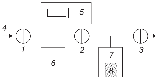
Рисунок 1 — Принципиальная схема двухкамерного порозиметра
