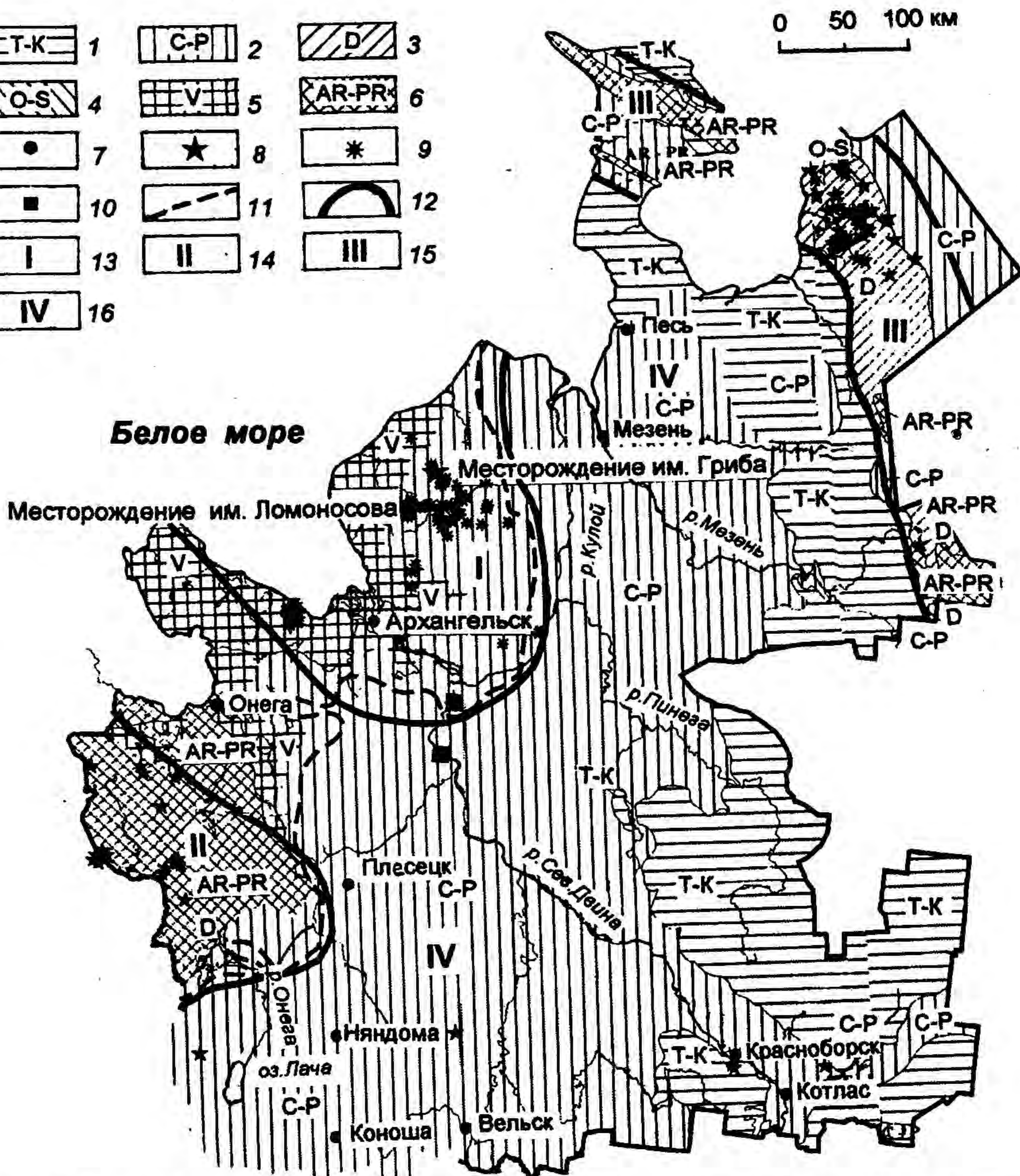
Рис. 1. Схема районирования Архангельской алмазонасной провинции: 1—6 — структурно-металлогенетические комплексы: 1 — триасово-меловой, 2 — каменноугольно-пермский, 3 — девонский, 4 — ордовикско-силурийский, 5 — вендский; 6 — архейско-протерозойский; 7 — трубки взрыва; 8 — месторождения алмазов; 9 — находки алмазов в четвертичных образованиях; 10 — находки обломков кимберлитов; 11 — изопакита палеозойского перекрывающего комплекса 150 м; 12 — границы районов; 13—16 — алмазонасные районы: 13 — Зимнебережный, 14 — Онежский, 15 — Канино-Тиманский, 16 — Двинской
