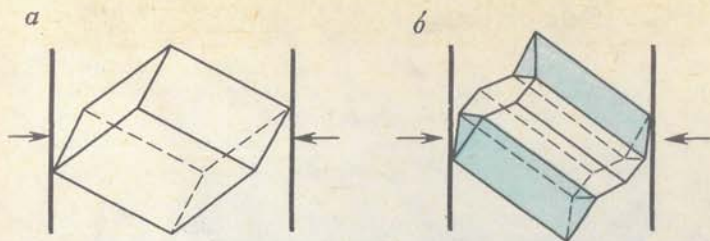
Рис. 42. Механическое двойникование кальцита. а — кристалл до двойникования; б — кристалл после двойникования
