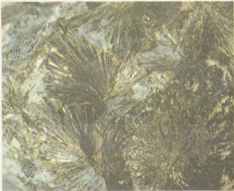
Рис. 52. Радиально-лучистые агрегаты астрофиллита. Хибинны
