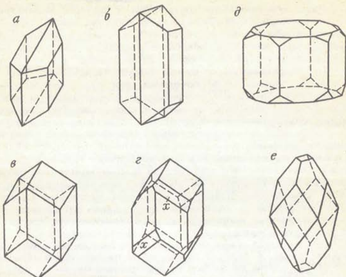
Рис. 5. Примеры кристаллов различных классов симметрии: а — гипс L_2PC ; б — арагонит 3L_23PC , в, г — диоптаз L_3C ; д — берилл L_6L_27PC ; е — апофиллит L_4L_25PC
