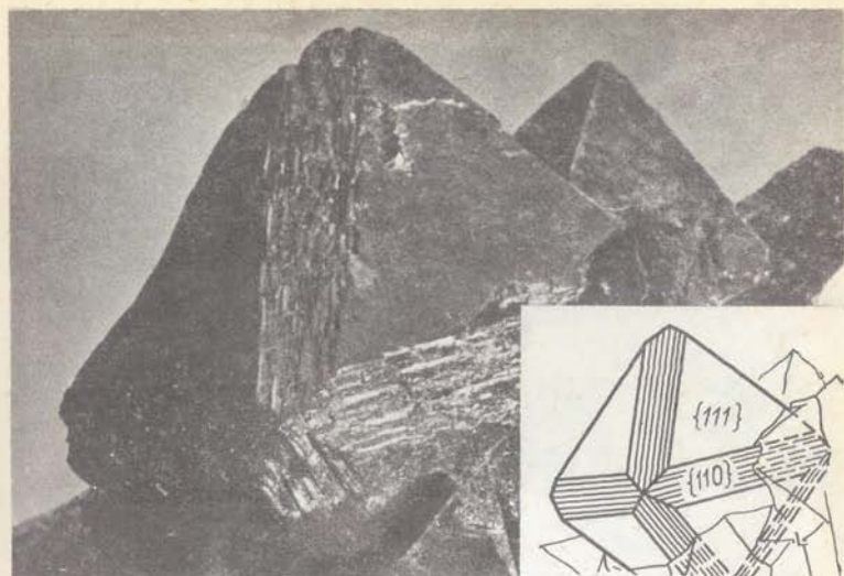
Рис. 24. Магнетит. Дашкесан, Азербайджан
