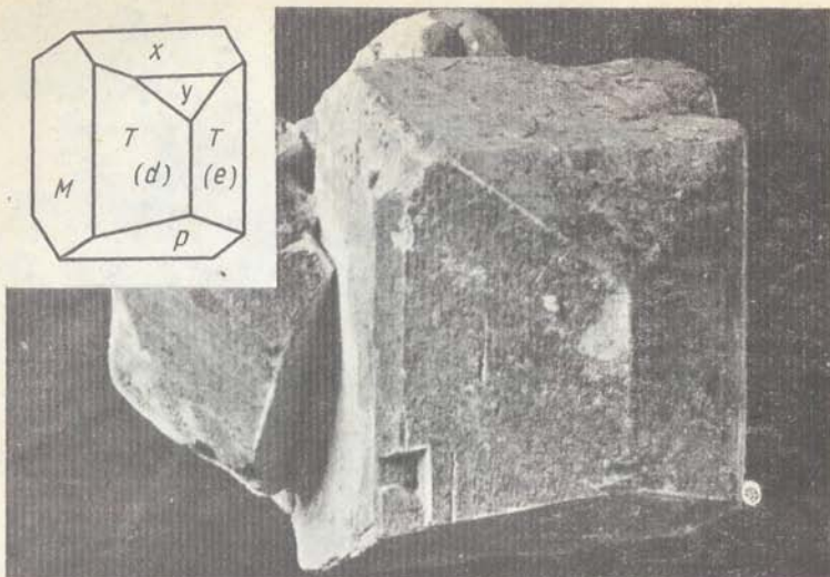
Рис. 14. Ортоклаз. Украина
