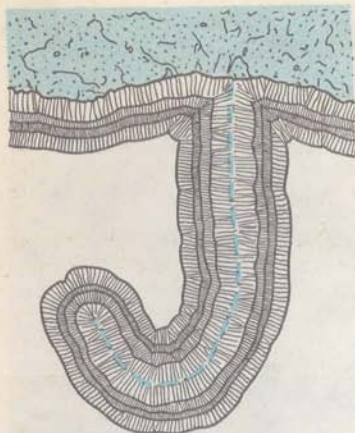
Рис. 59. Строение псевдосталактита
