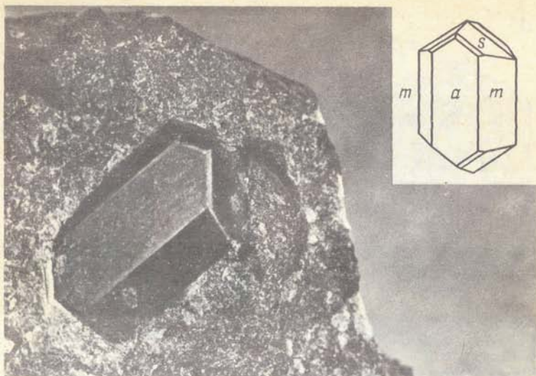
Рис. 12. Кристалл рамзаита. Хибины
