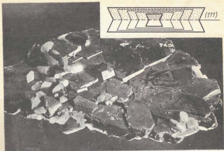
Рис. 41. Таблитчатый двойник галенита по шпинелевому закону. Сихотэ-Алинь
