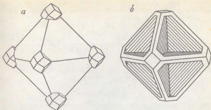
Рис. 28. Скелетные кристаллы:
