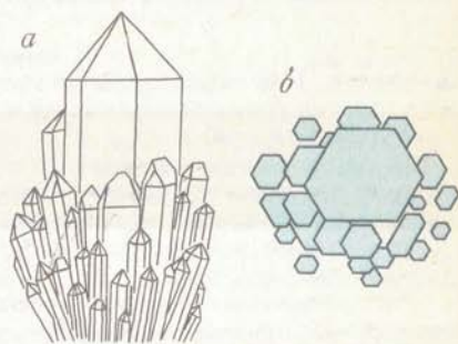
Рис. 48. Расщепленный кристалл кварца: субиндивиды разориентированы относительно направления наибольшего роста (а), но сохраняют параллельную ориентировку в поперечном направлении (б)
