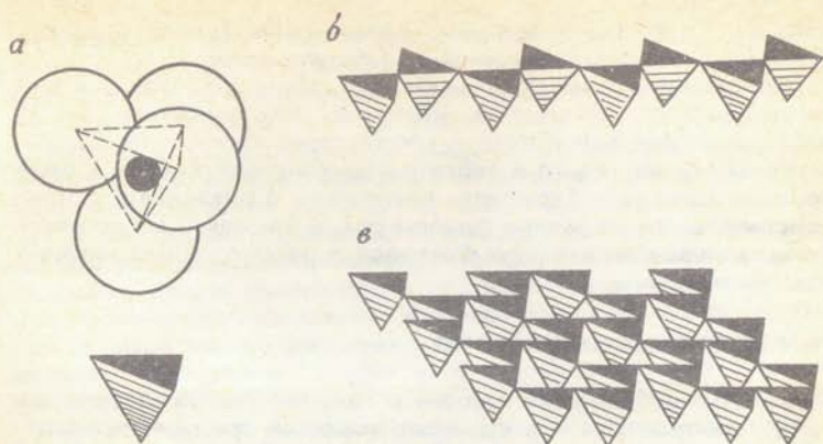
Рис. 18. Кристаллические структуры силикатов: а — кремнекислородный тетраэдр; б — цепочечный структурный мотив пироксена; в — листовая (слоистый) структурный мотив слюды
