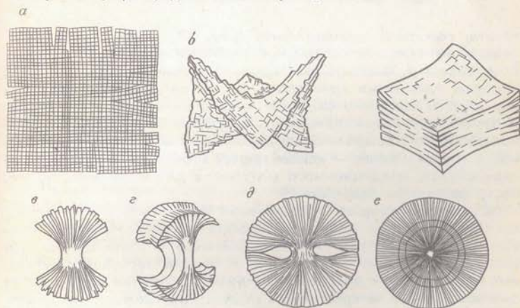
Рис. 44. Блочное строение [а] и формы расщепления кристаллов: седло (б), сноповидный сросток (в), двулистник (д), сферокристалл (е), сферолит (е)
