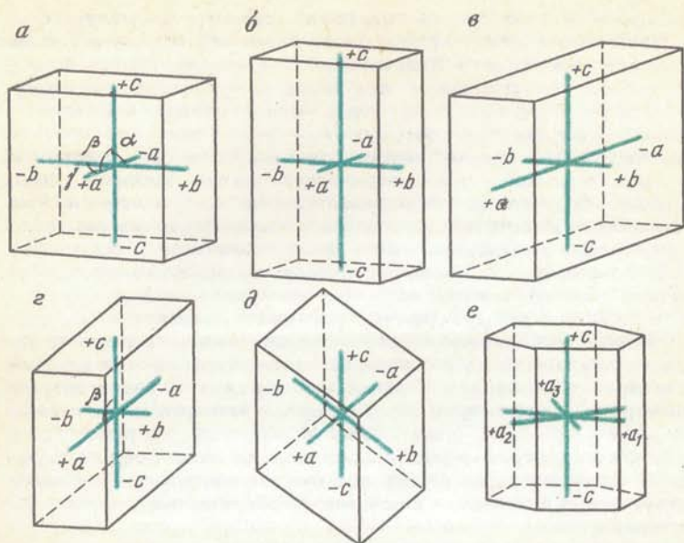
Рис. 6. Осевые кресты в кубической [а], тетрагональной [б], ромбической [в], моноклинной [г], триклинной [д], тригональной и гексагональной [е] сингониях
