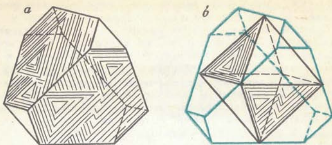
Рис. 10. Кристалл сфалерита:
