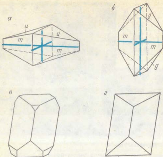
Рис. 13. Минералы моноклинной сингонии:
