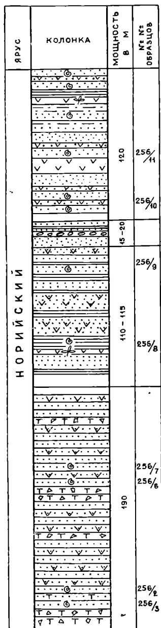
Рис. 7. Стратиграфическая колонка верхнетриасовых отложений бассейна р. Малая Кутинская (по Г. П. Тереховой, 1938 г.).
