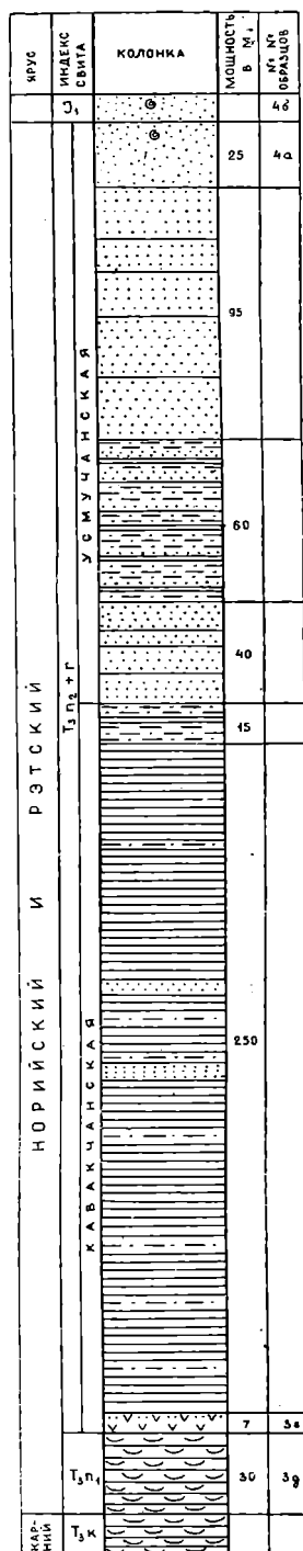
Рис. 5. Стратиграфическая колонка норийско-рэтских отложений низовьев р. Асибеган (по Р. Б. Умитбаеву, 1963 г.).
