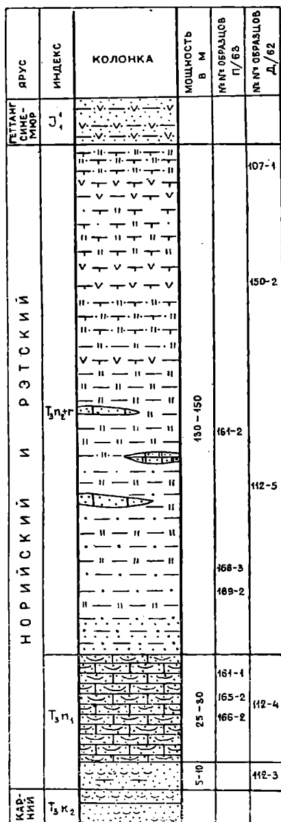
Рис. 12. Стратиграфическая колонка норийско-рэтских отложений среднего течения р. Булун (Рассоха) (по И. В. Полуботко, 1963 г.).
