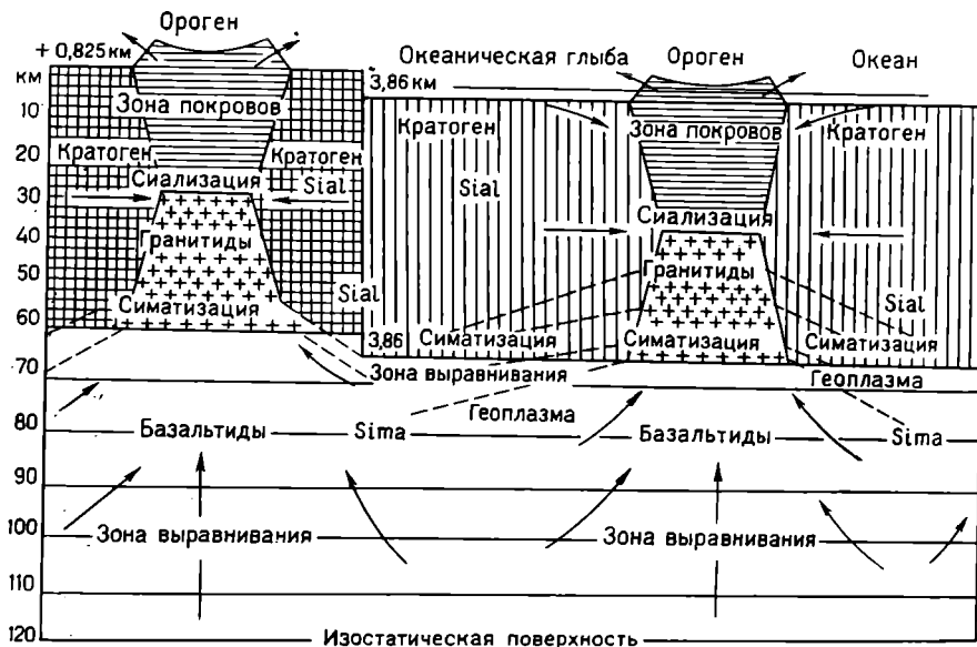
Рис. 1. Деление земной коры по орогенной теории Л. Кобера [Моисеев, 1939].
