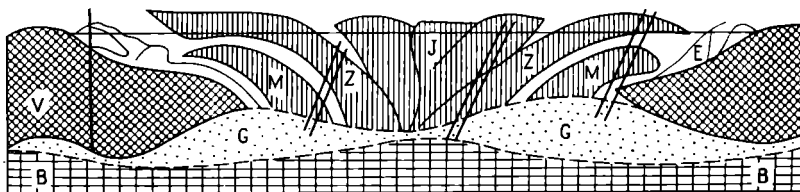
Рис. 2. Схематический разрез орогена по Л. Коберу [Бубнов, 1960]: V — форланд, E — экстерниды, M — метаморфиды, Z — централиды, J — интерниды, G — гранитовая зона, B — базальтовая зона
