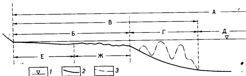
Рис. 13. Схема элементов рельефа дна подводной окраины материков [Николаев, 1975]
