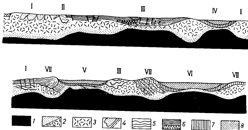
Рис. 7. Гипотетические разрезы земной коры, изображающие элементы расчленения [Милановский, 1929]
