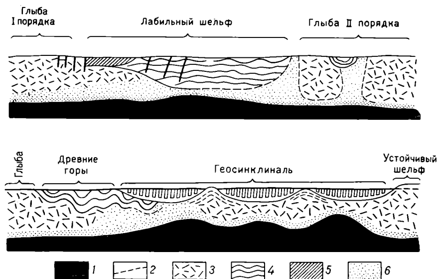
Рис. 4. Гипотетические профили, иллюстрирующие расчленение земной коры на основные структурные элементы по С. П. Бубнову [Милаповский, 1929] 1 — базальтовый субстрат; 2 — переходная зона основных пород в основании гнейсового фундамента; 3 — гнейсовый фундамент; 4 — осадочный покров; 5 — море; 6 — переход базальтового субстрата в гнейсовый фундамент
