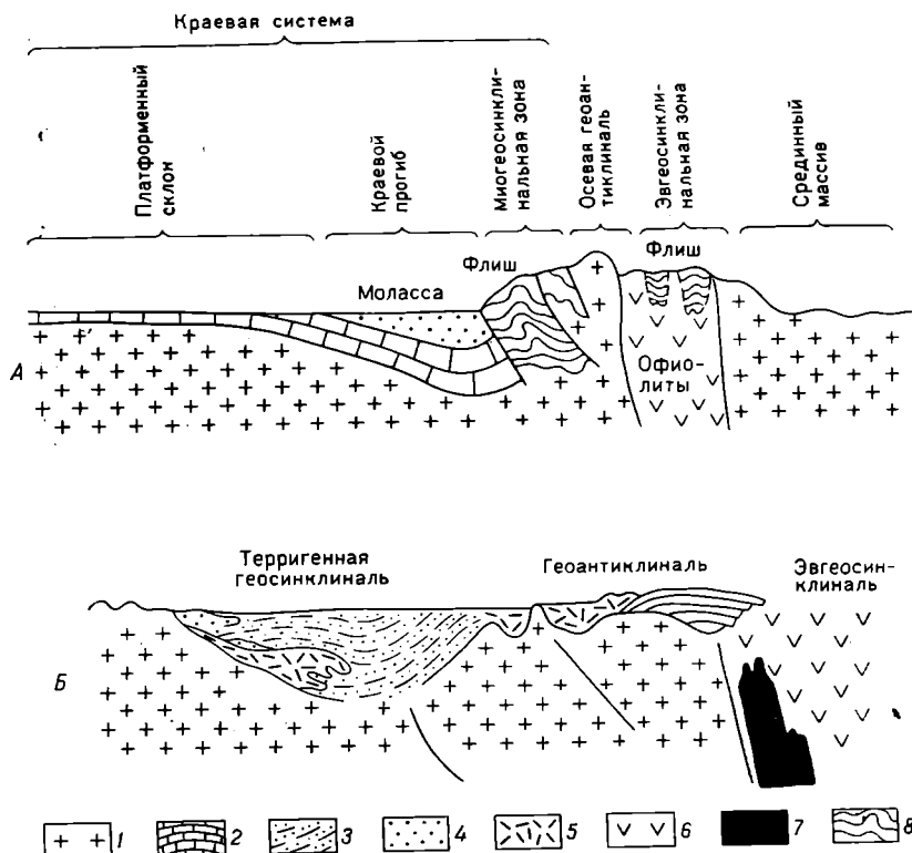
Рис. 12. Строение геосинклинальных областей: альпийского типа (А) и цент- рально-азиатского типа (Б) [Зоненшайн, 1972]
