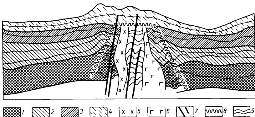
Рис. 14. Модель строения Срединно-Атлантического хребта [Пейве, 1975, 1976] 1 — юра; 2 — мел; 3 — палеоген; 4 — неоген; 5 — интрузия габбро; 6 — протрузия серпентинизированных ультрабазитов; 7 — дайки диабазов; 8 — границы метаморфического комплекса; 9 — деформированные комплексы центральной части хребта
