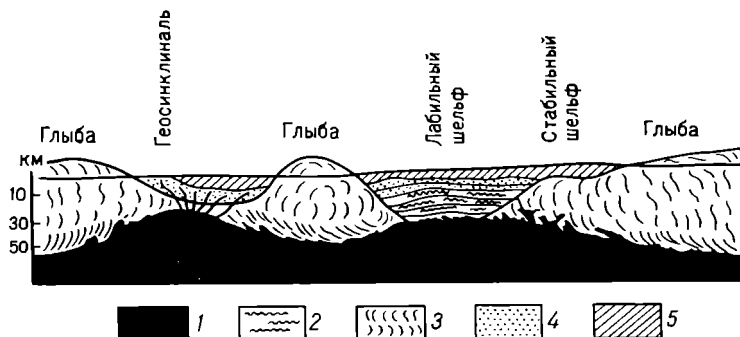
Рис. 5. Части геосинклинальной области по С. П. Бубнову [Моисеев, 1939] 1 — внутренняя оболочка из основных пород (сима); 2 — нижняя структура — складчатая, но не сложенная из метаморфических осадков; 3 — глубинная структура — внешняя оболочка, сложенная гнейсами; 4 — верхняя структура — нескладчатые осадки; 5 — море
