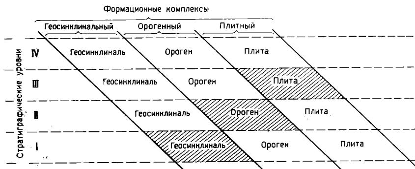
Рис. 10. Схема строения формационного комплекса [Соловьев, 1975]
