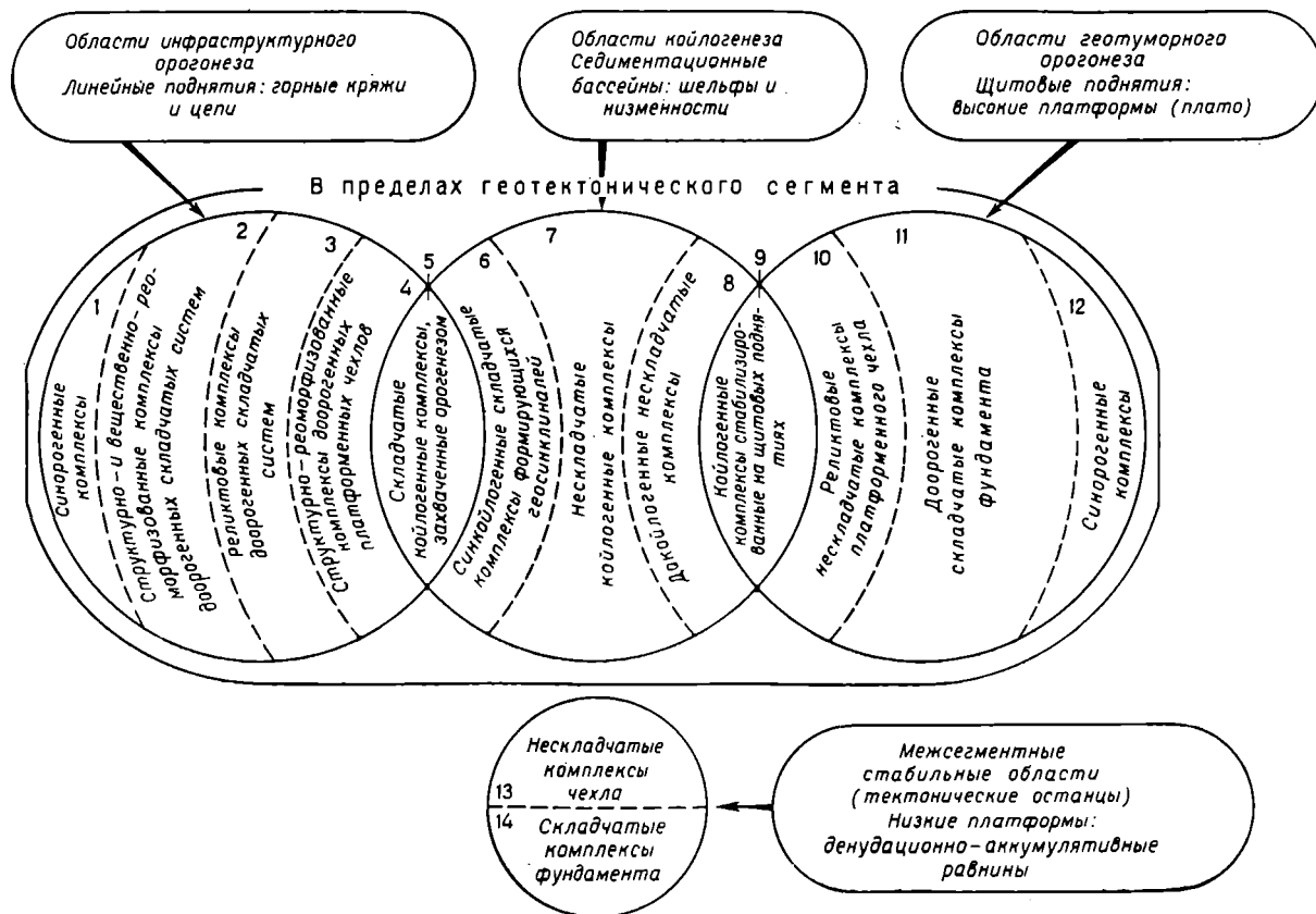
Рис. 11. Тектонические (структурно-вещественные) комплексы континентов [Погребницкий, 1975]
