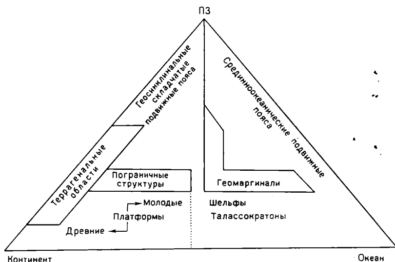
Рис. 9. Общая схема соотношения структур Земли [Красный, 1972]
