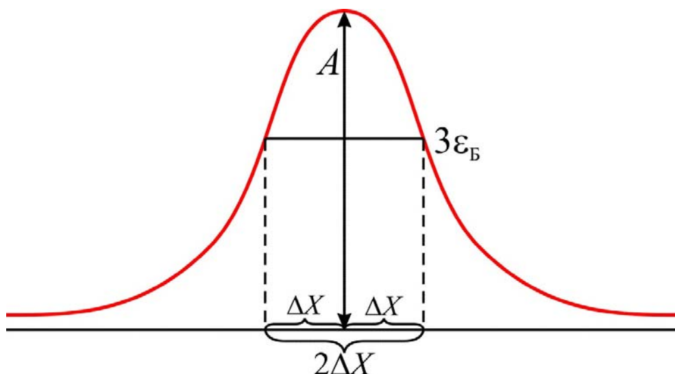
Рис. 2.1. Определение шага съемки гравиметрической съемки.
