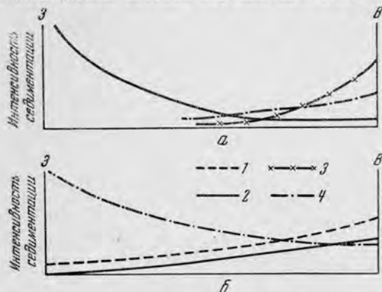
Фиг. 2. Изменение фациальных парагенезисов а — нижнемеловые карбонатные породы Южной Ферганы; б — карбонатные породы устричной свиты Южной Ферганы; 1 — глина, 2 — известняк, 3 — песчаник, 4 — доломит.
