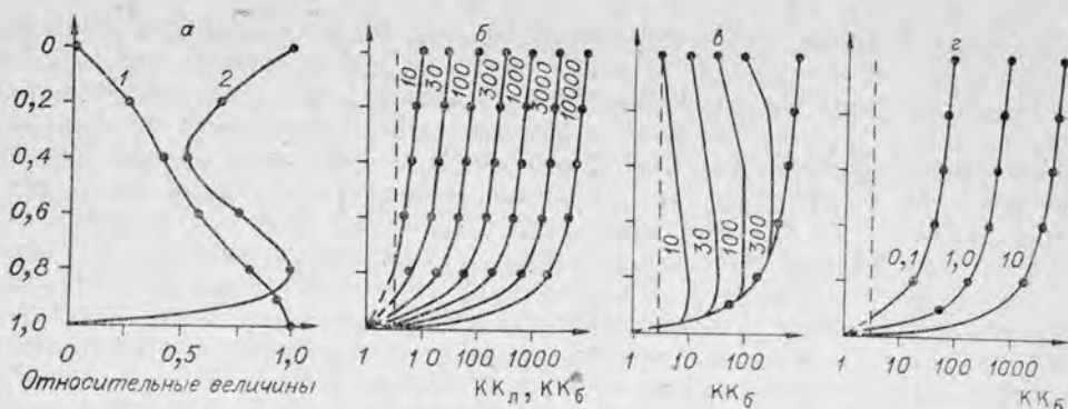
Рис. 52. Палетки зависимостей коэффициента контрастности биогеохимических аномалий ( KK_б ) при двух одинаковых максимумах корневой активности растений.
