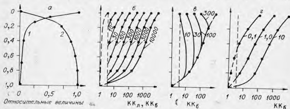
Рис. 51. Палетки зависимостей коэффициента контрастности биогеохимических аномалий ( KK_b ) при корневой активности растений, уменьшающейся с глубиной.
