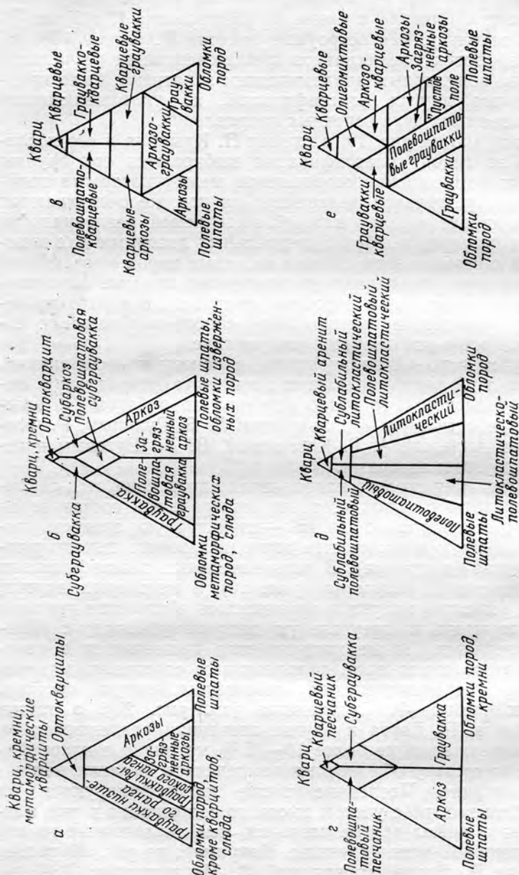
Рис. 19. Сравнение классификаций песчаных пород по составу обломочных зерен с применением треугольной диаграммы. Диаграммы: а — по П. Крынину [Krynine P., 1948 г.]; б — по Р. Фолку [Folk R., 1954 г.]; в — по Л. Б. Рухину [1956 г.]; г — по Т. Ван Анделу [Van Andel T., 1953 г.]; д — по К. Круку [Crook K., 1960 г.]; е — по А. Г. Коссовской [1962 г.].
