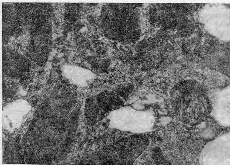
Рис. 35. К-аркозовый кварцито-песчаник зоны глубокого метаморфизма, сложенный обломками кварца, микроклина, ортоклаза, единичными зернами альбита.
