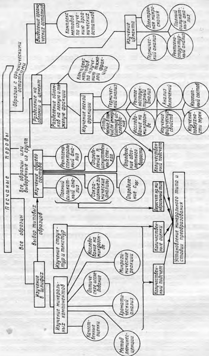
Рис. 3. Схема полного лабораторного петрографического изучения песчаных пород.
