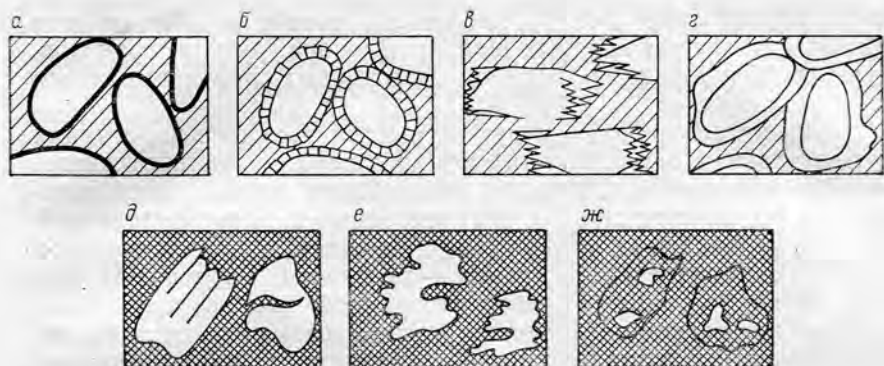
Рис. 13. Типы цемента по взаимоотношению с обломочными зернами. а — пленочный; б — кристификационный; в — неравномерного нарастания; г — регенера- ционный; д — проникновения; е — коррозионный; ж — замещения.
