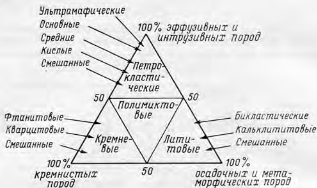
Рис. 38. Диаграмма минеральных разновидностей и разновидностей песчаников семейства граувакк, выделяемых по составу обломков.
