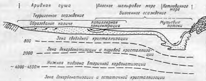
Рис. 16. Схема образования и преобразования карбонатных цементах песчаных пород.
