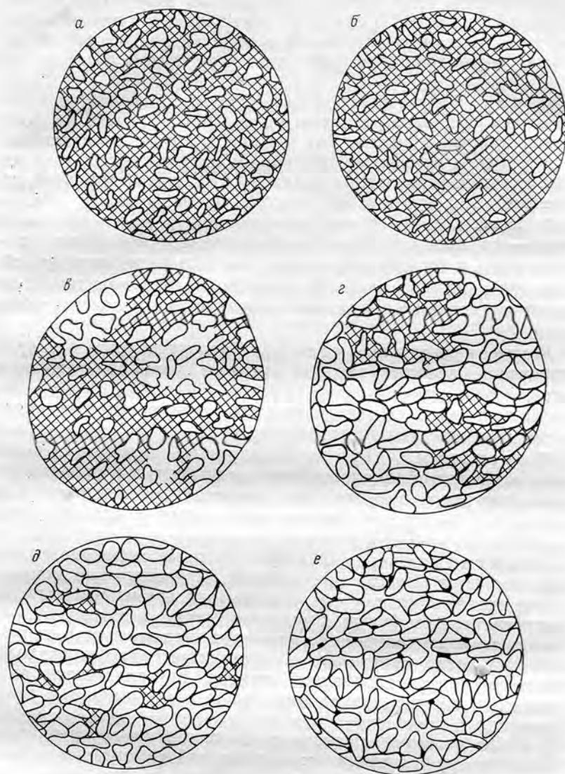
Рис. 12. Типы цемента по равномерности заполнения межзернового пространства. а — сплошной равномерный; б — сплошной неравномерный; в — преобладающий не- сплошной; г — пятнистый; д — островной; е — точечный.
