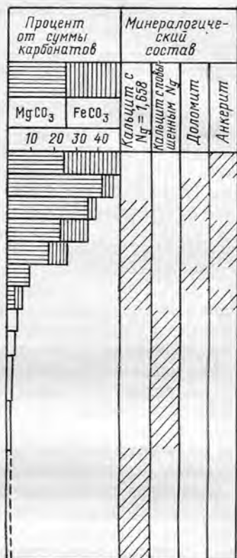
Рис. 15 Зависимость распространения карбонатных минералов в цементе песчано-алевритовых пород от содержания в нем карбонатов магния и железа (по В. И. Муравьеву [1971 г.]).
