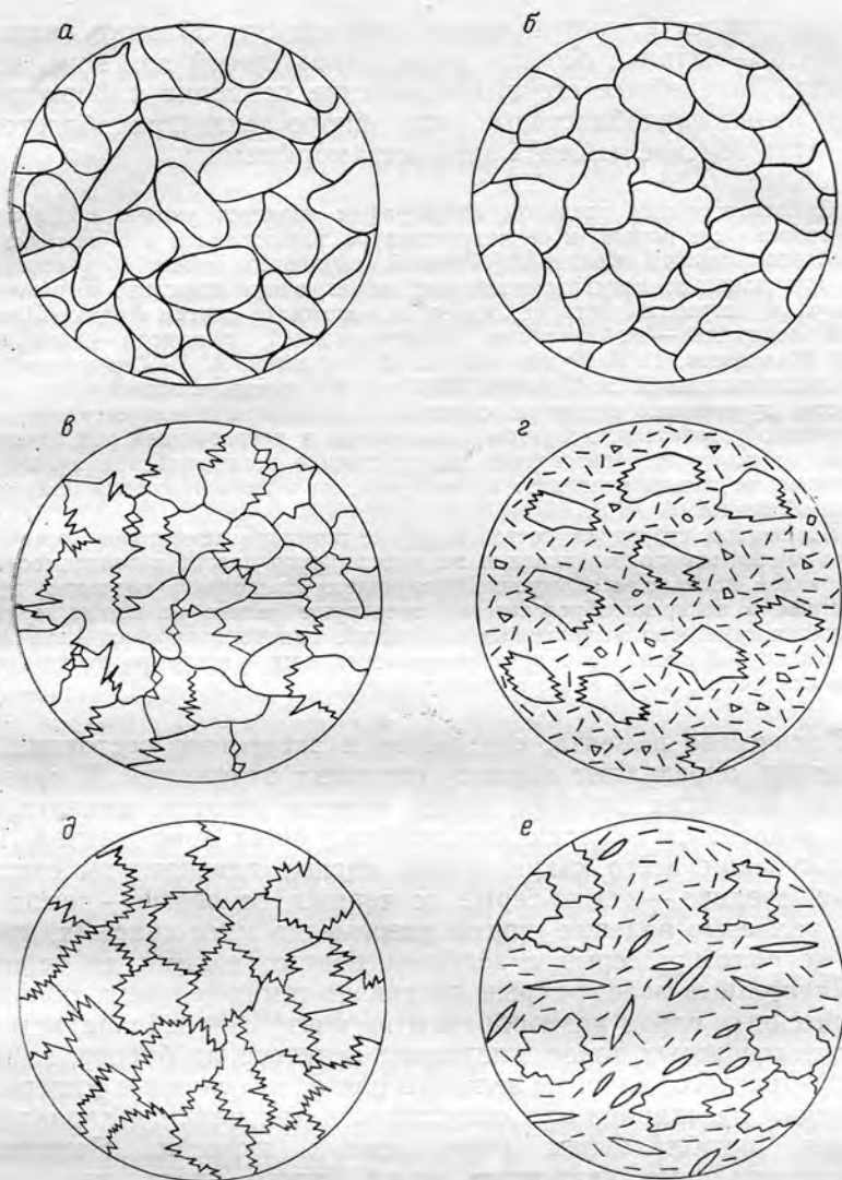
Рис. 14. Структуры бесцементных пород.
