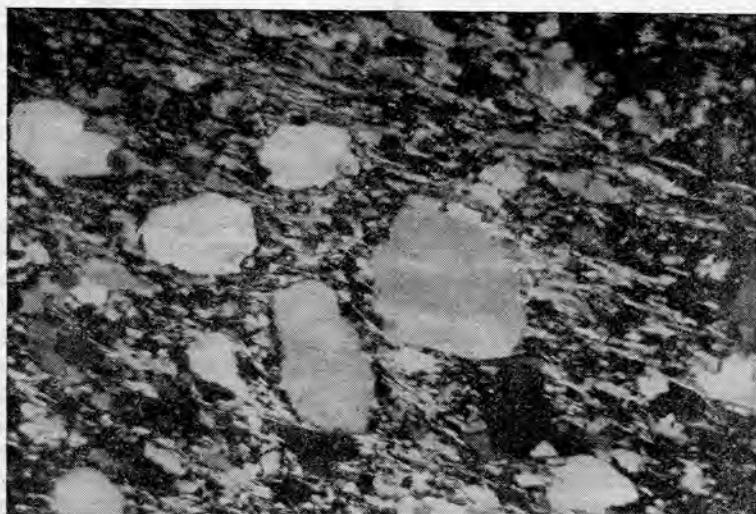
Рис. 41. Кварцево-граувакковый песчаник зоны глубокого метатенеза. Все обломочные компоненты, кроме кварца, превращены в слюдиисто-хлорит-альбит-кварцевый агрегат с гранолепидобластовой структурой и ориентированной слоистой текстурой. Реликтовые крупные обломочные зерна кварца переработаны кристаллизационным бластезом; 60\times , с анализатором. Ягнобская серия (O—S 1 ) Зеравшанского хребта.
