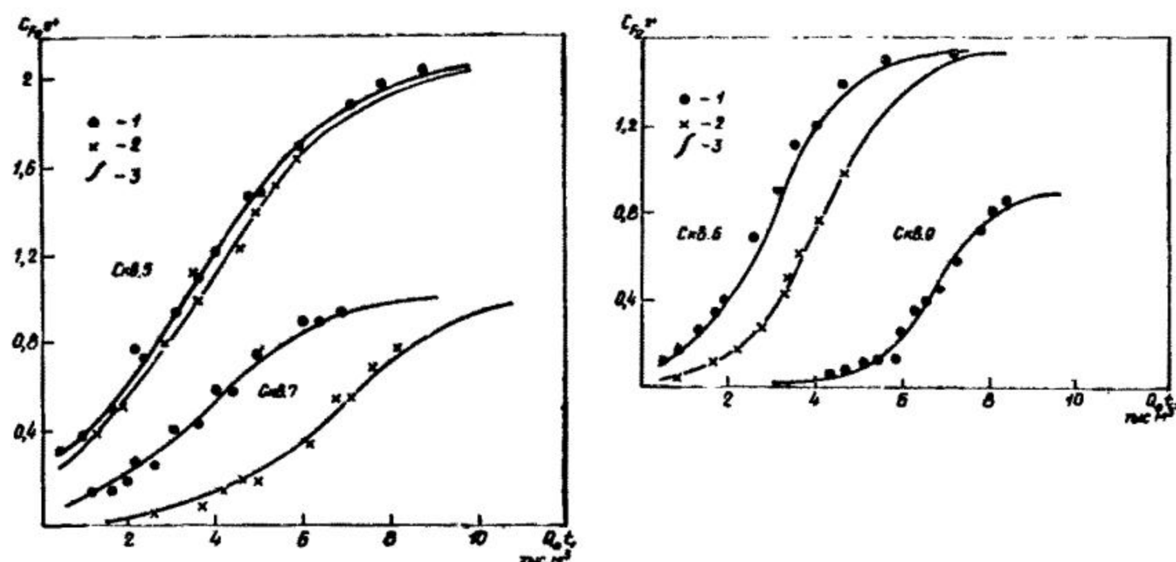
Рис. 21.9. Выходные кривые
