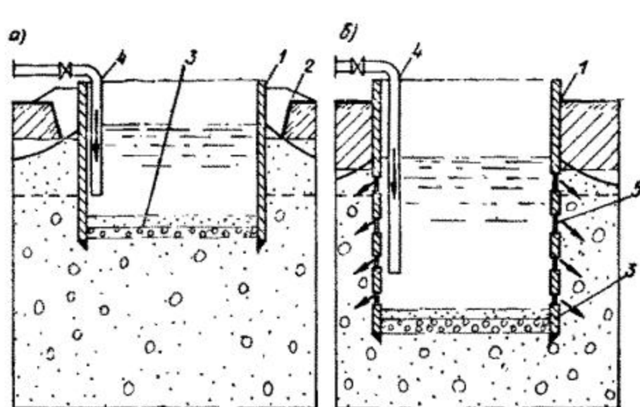
Рис. 13.7. Схемы шурфов
