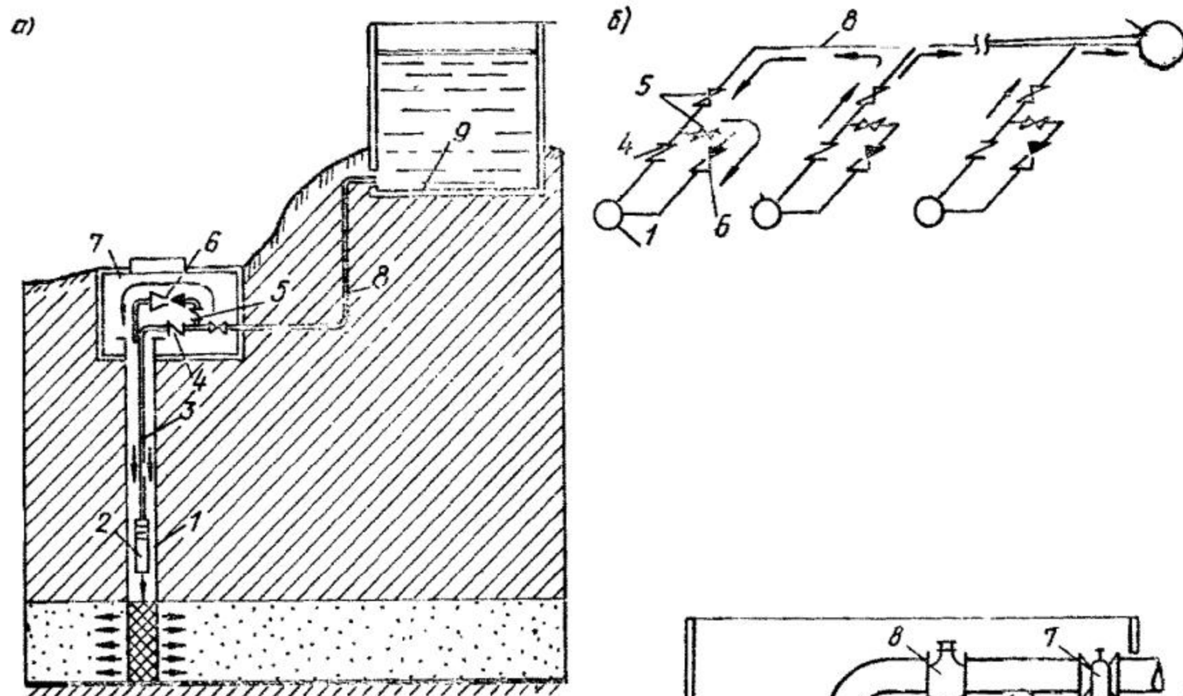
Рис. 21.3. Система водоснабжения (а, б) с установками обезжелезивания циклического типа
