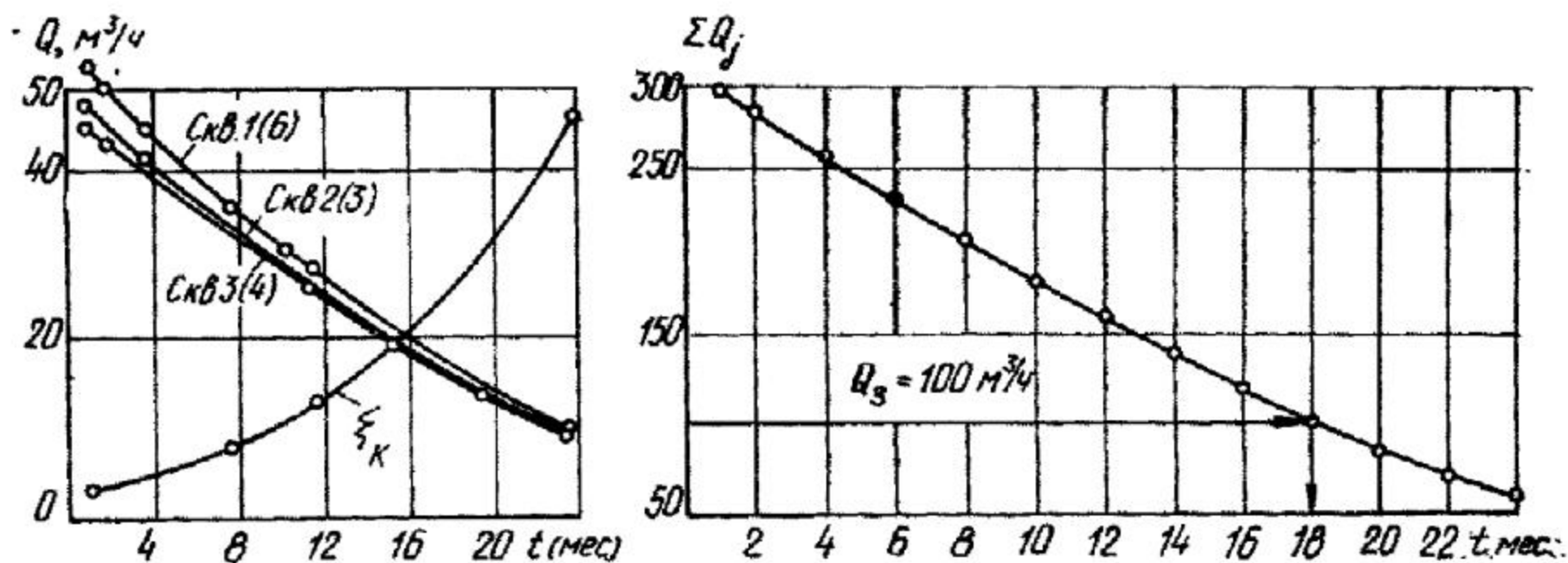
Рис. 7.7. Расчетные графики изменения во времени \xi_K(t) , Q_i(t) и \Sigma Q(t) при действии скважин в режиме S_j = \text{const}
