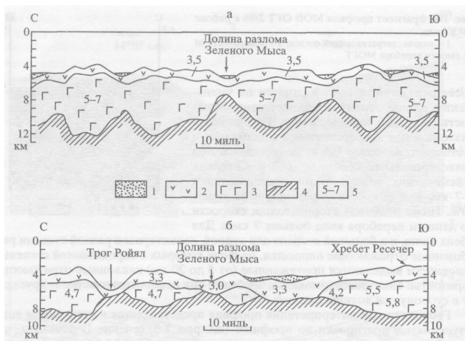
Рис. 1.9. Глубинные разрезы литосферы по профилям 2/86 (а) и 3/86 (б) 1 - осадочная толща; 2 - первая толща (геофизический слой 2А); 3 - вторая толща (слои 2В, 2С и 3); 4 - поверхность Мохоровичича; 5 - значения скоростей продольных сейсмических волн, км/с
