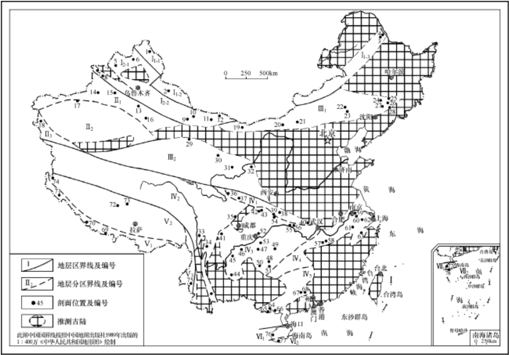
图 5-1 中国志留纪地层区划图
