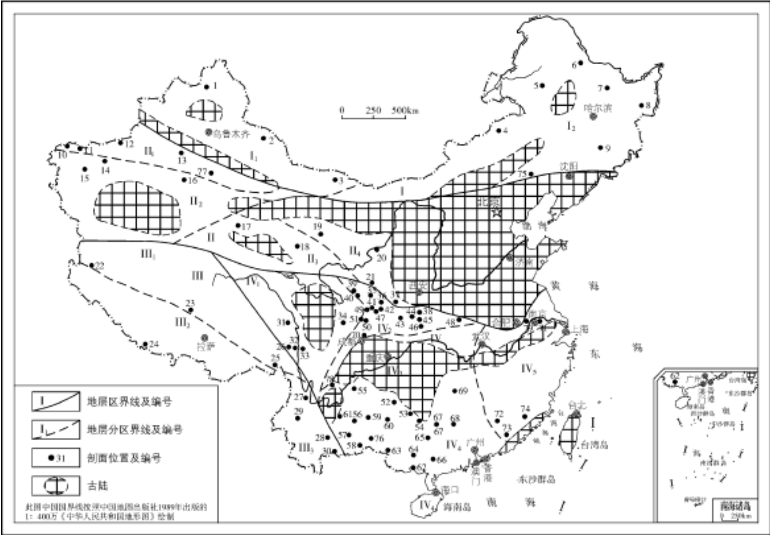
图 6-1 中国泥盆纪地层区划图
