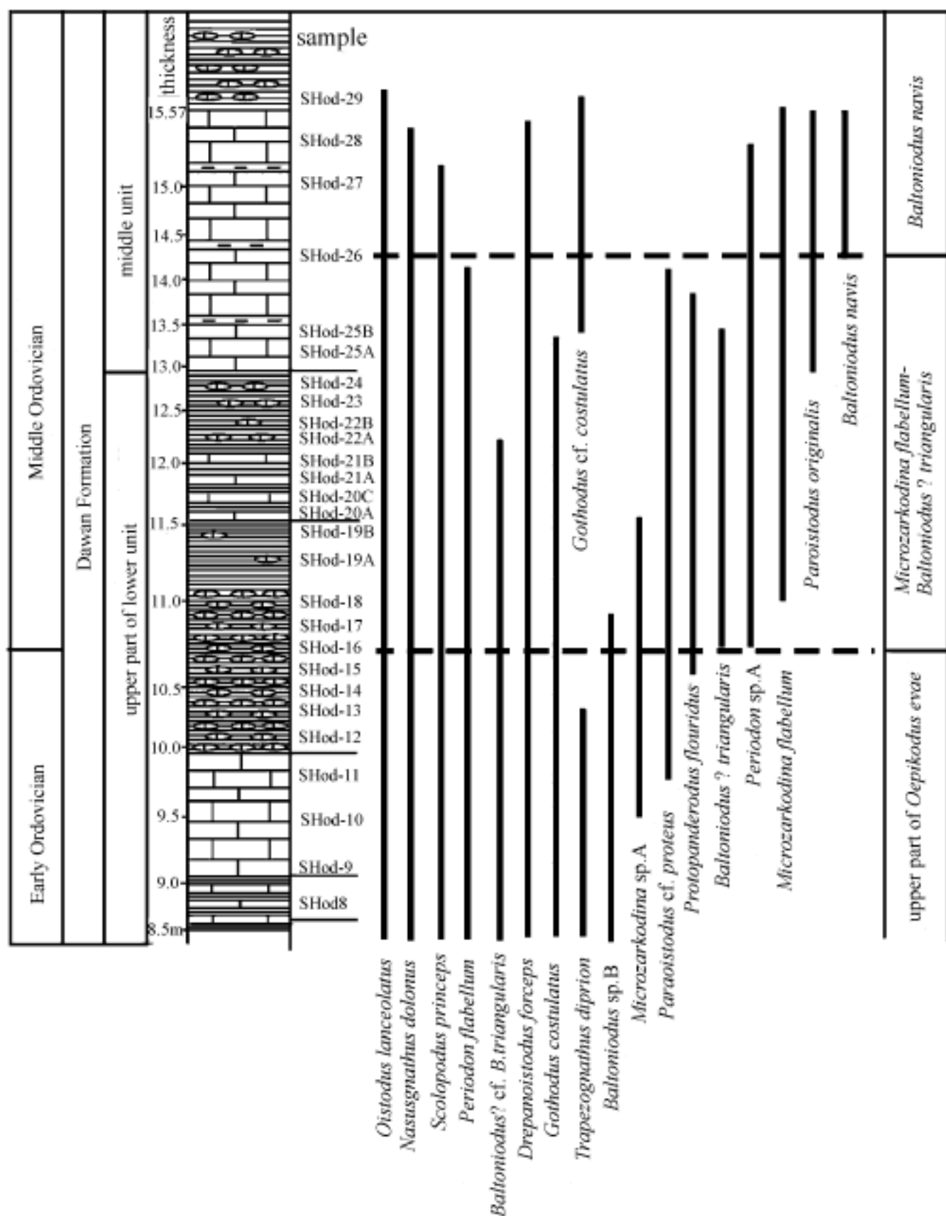
图 4-2 湖北宜昌黄花场剖面大湾阶底界附近牙形石化石分布图
