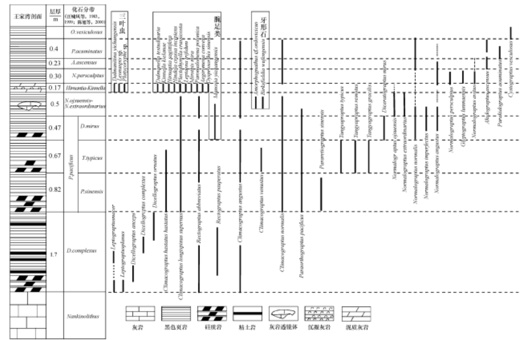
图 5-2 宜昌王家湾剖面龙马溪阶底界附近笔石、三叶虫和腕足类的分布 (据汪啸风等，1983，1987；陈旭等，2000)
