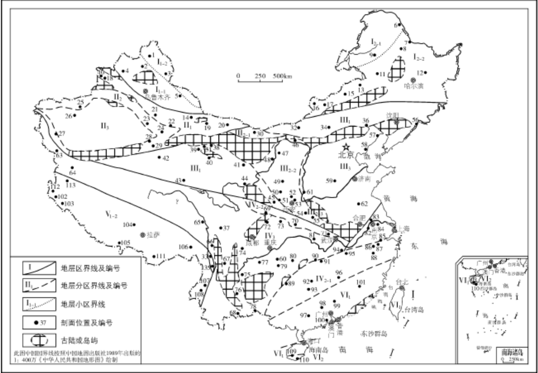
图 4-1 中国奥陶纪地层区划图
