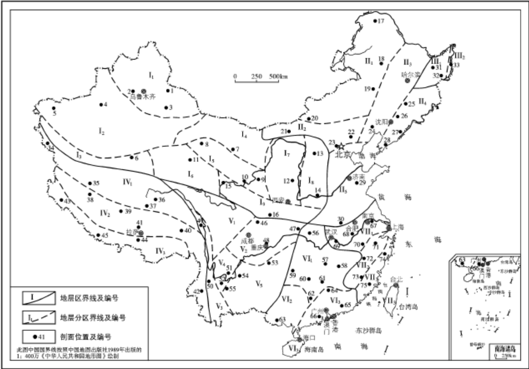
图 10-1 中国侏罗纪地层区划图
