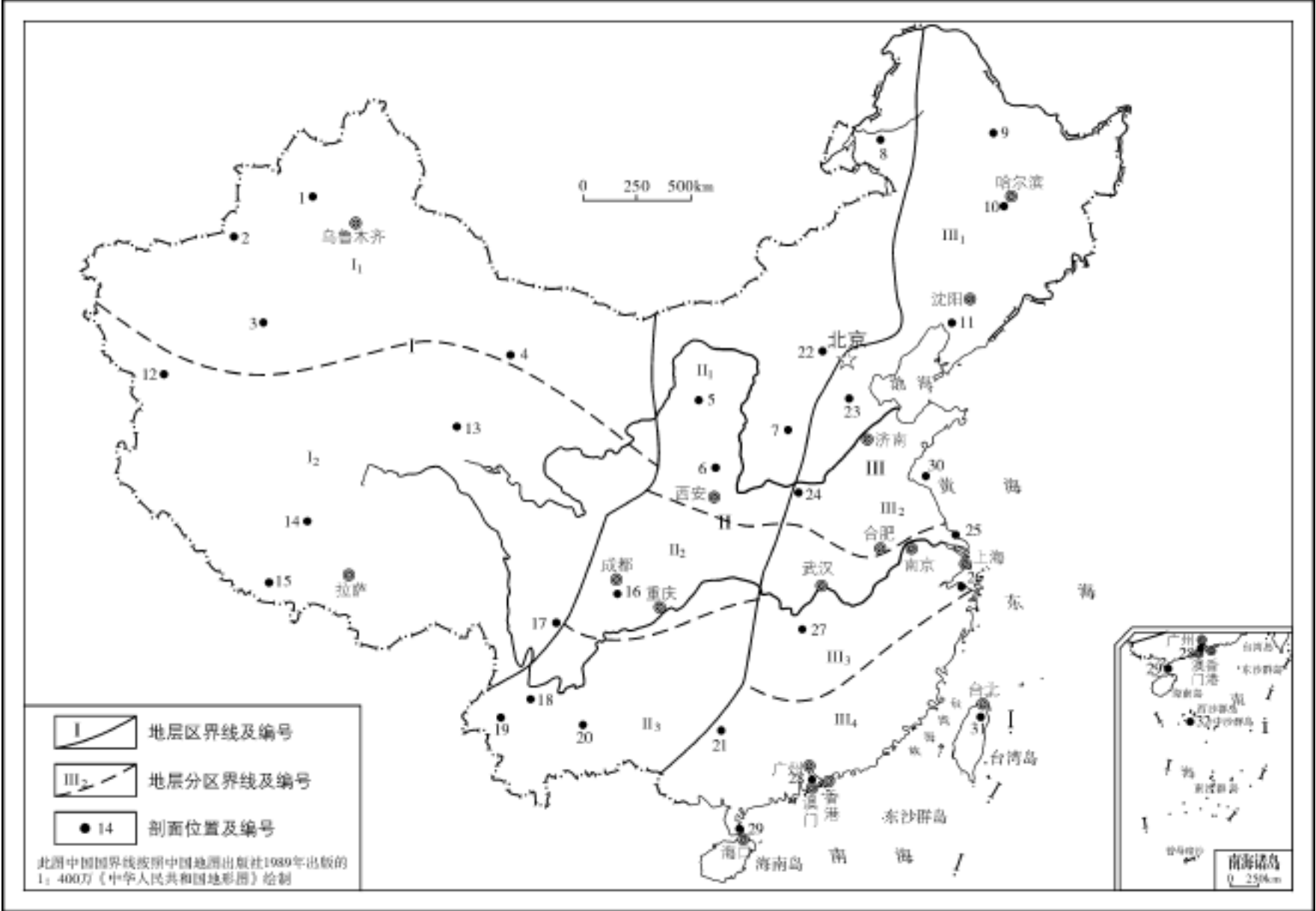
图 14-1 中国第四纪地层区划图
