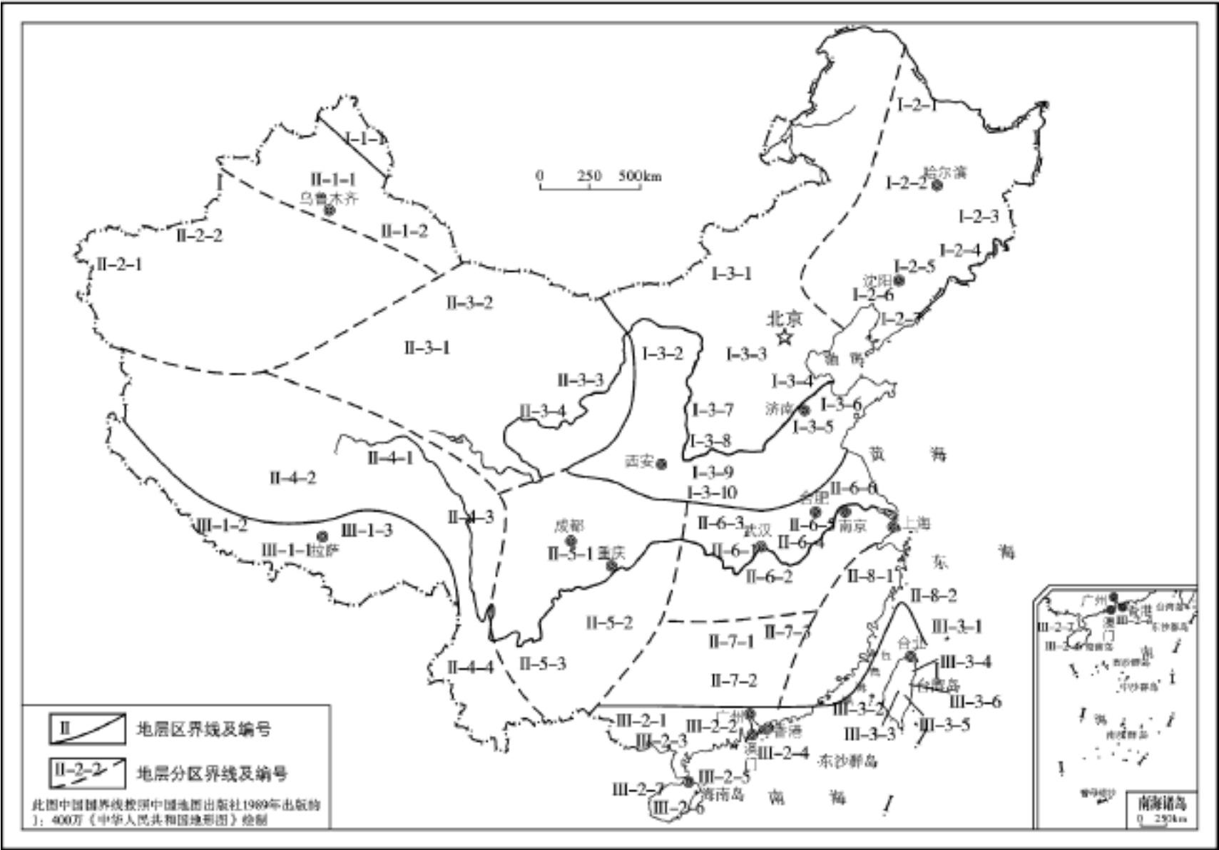
图 12-1 中国古近纪地层划分图
