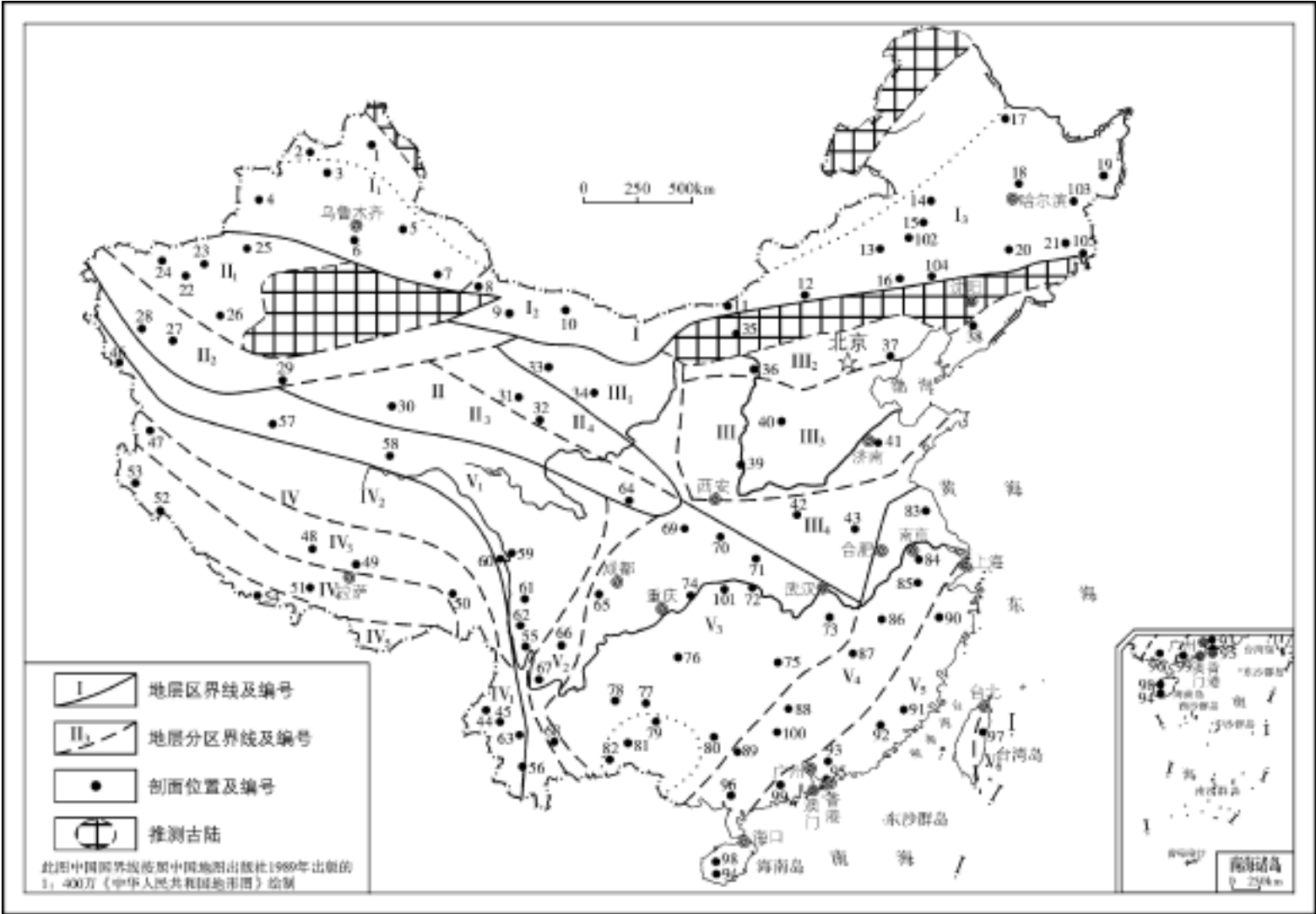
图 8-1 中国二叠纪地层区划图
