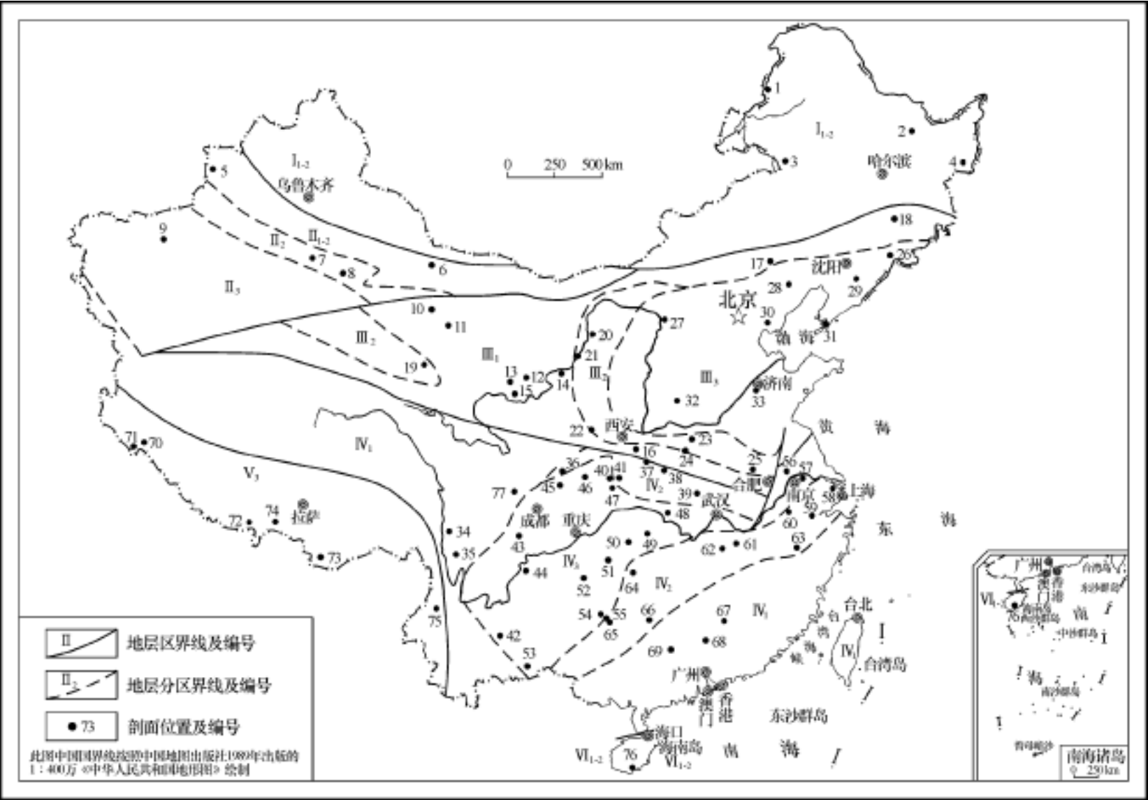
图 3-1 中国寒武纪地层区划图
