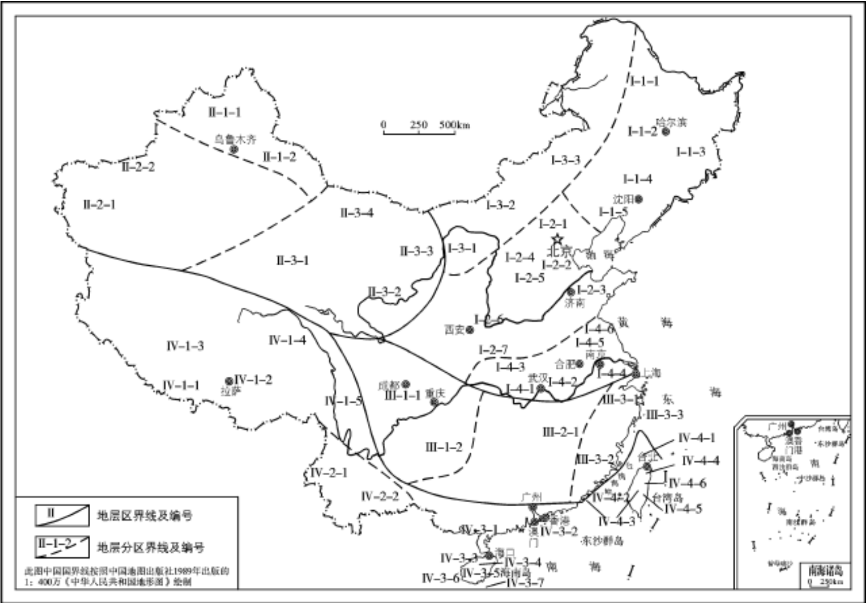
图 13-1 中国新世纪地层区划图
