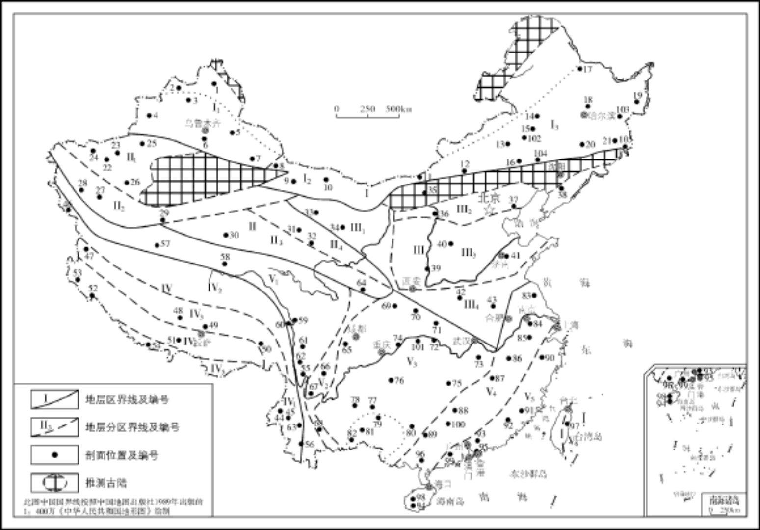
图 7-1 中国石炭纪地层区划图
