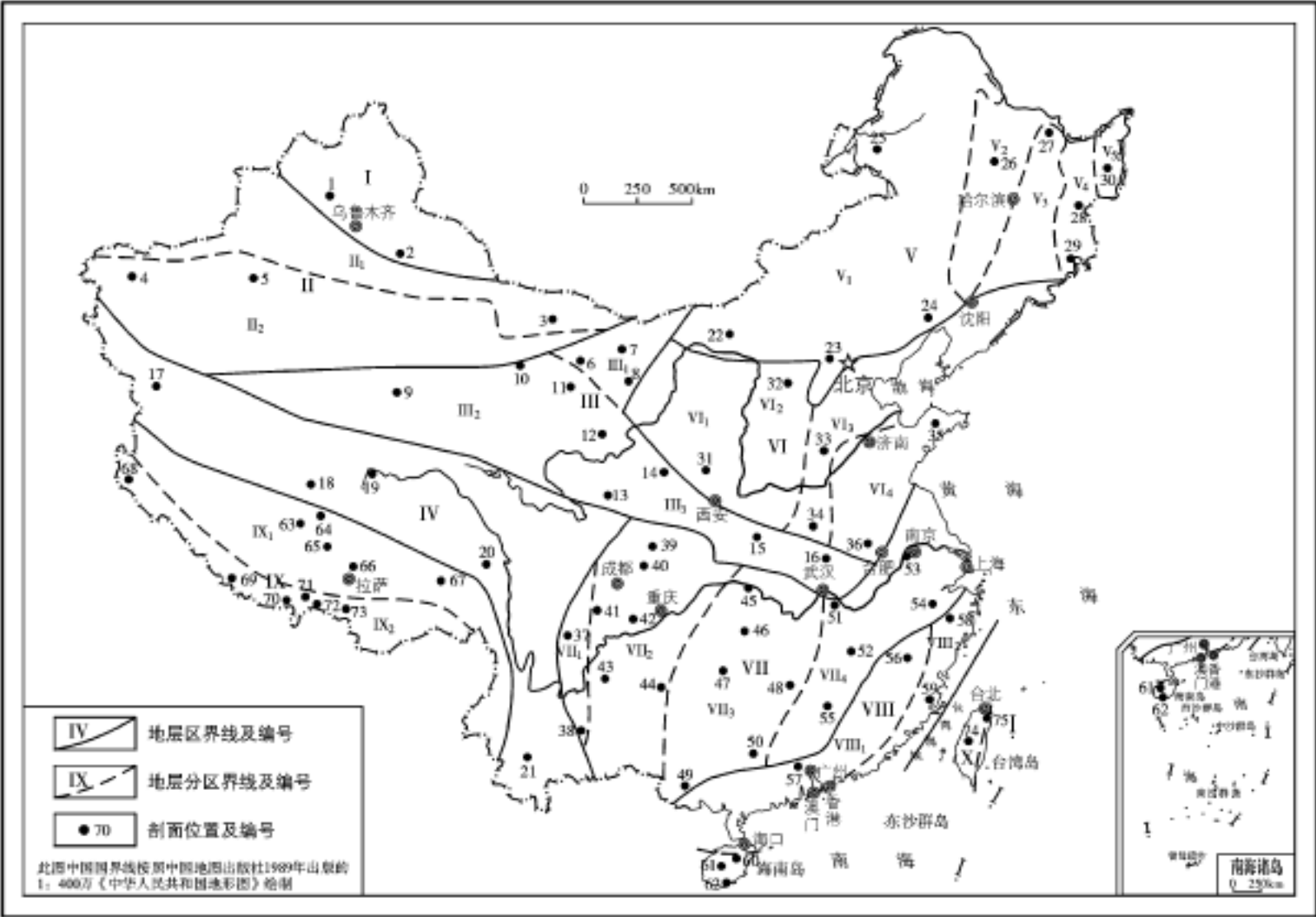
图 11-1 中国白垩纪地层区划图
