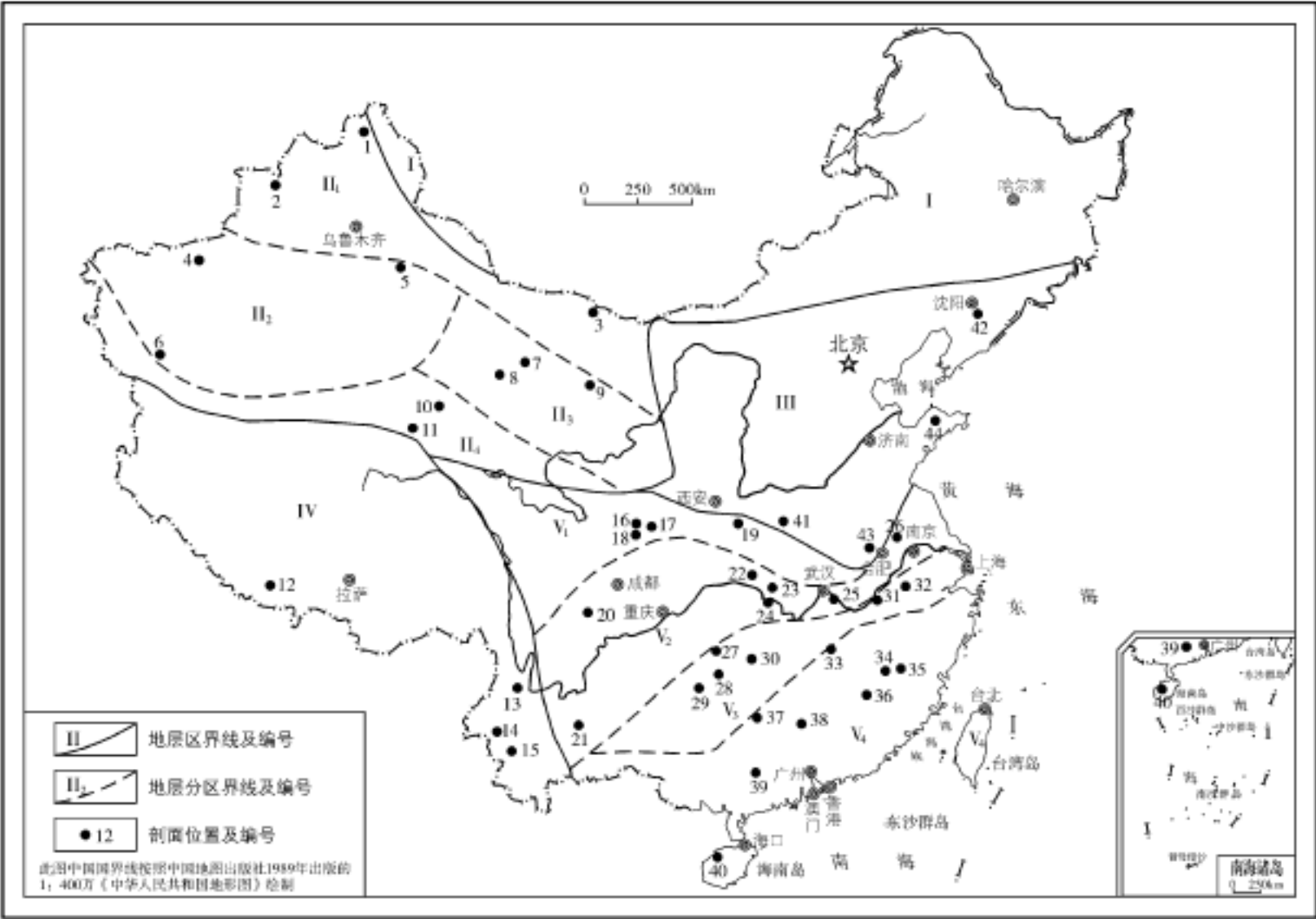
图 1-1 中国南华纪地层区划图
