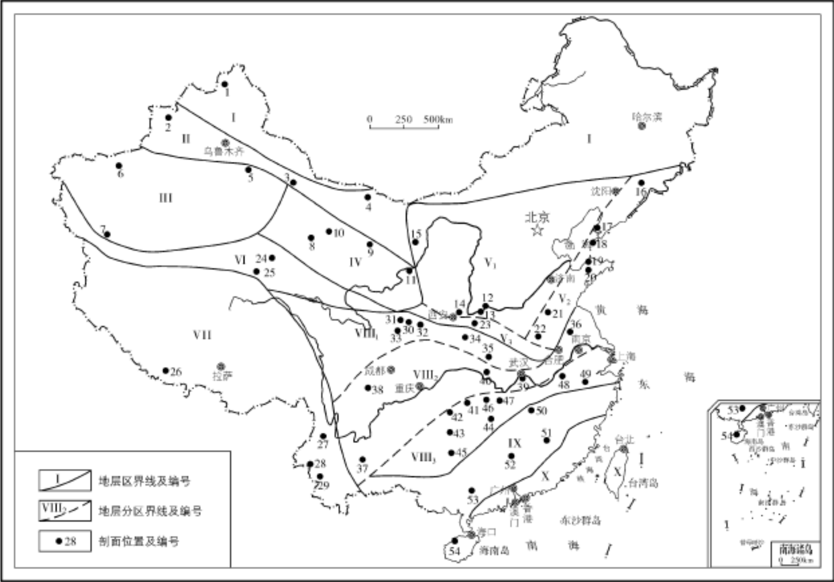
图 2-1 中国震旦纪地层区划图
