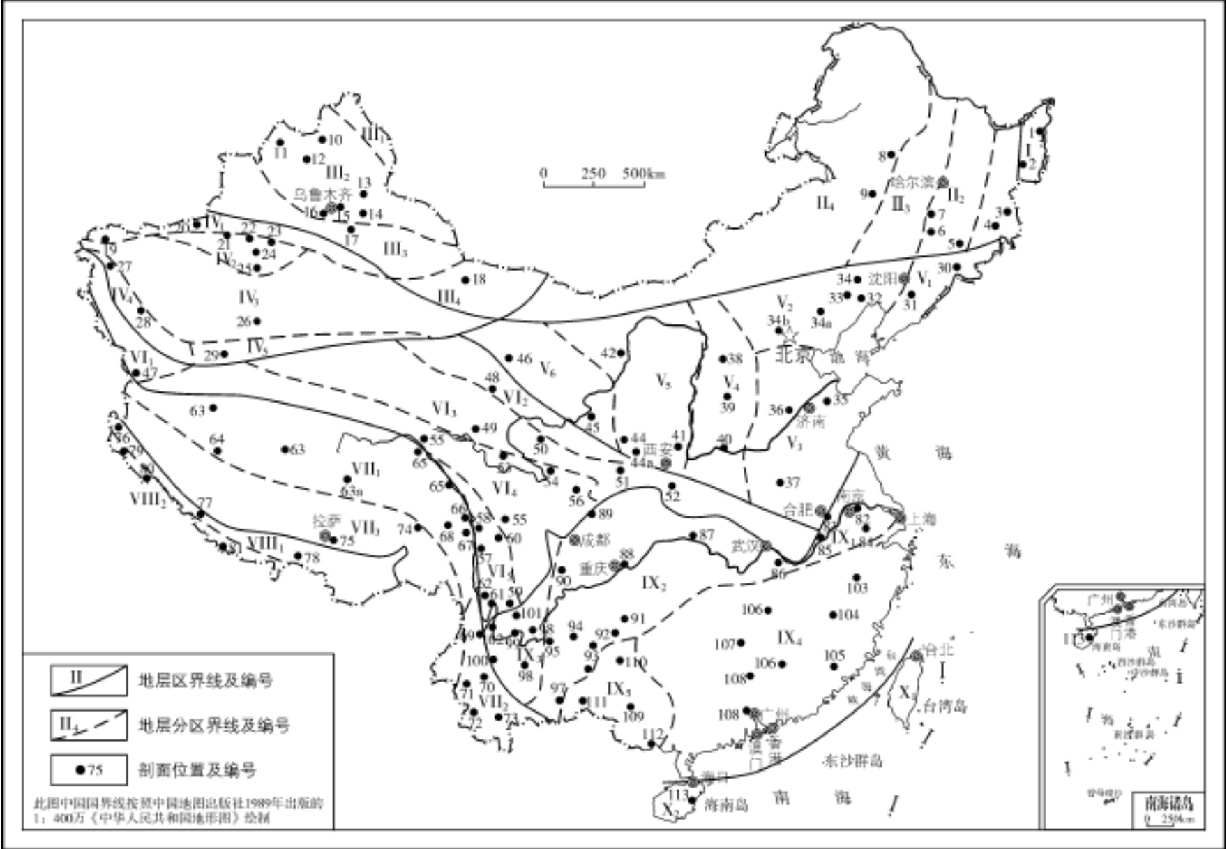
图 9-1 中国三叠纪地层区划图
