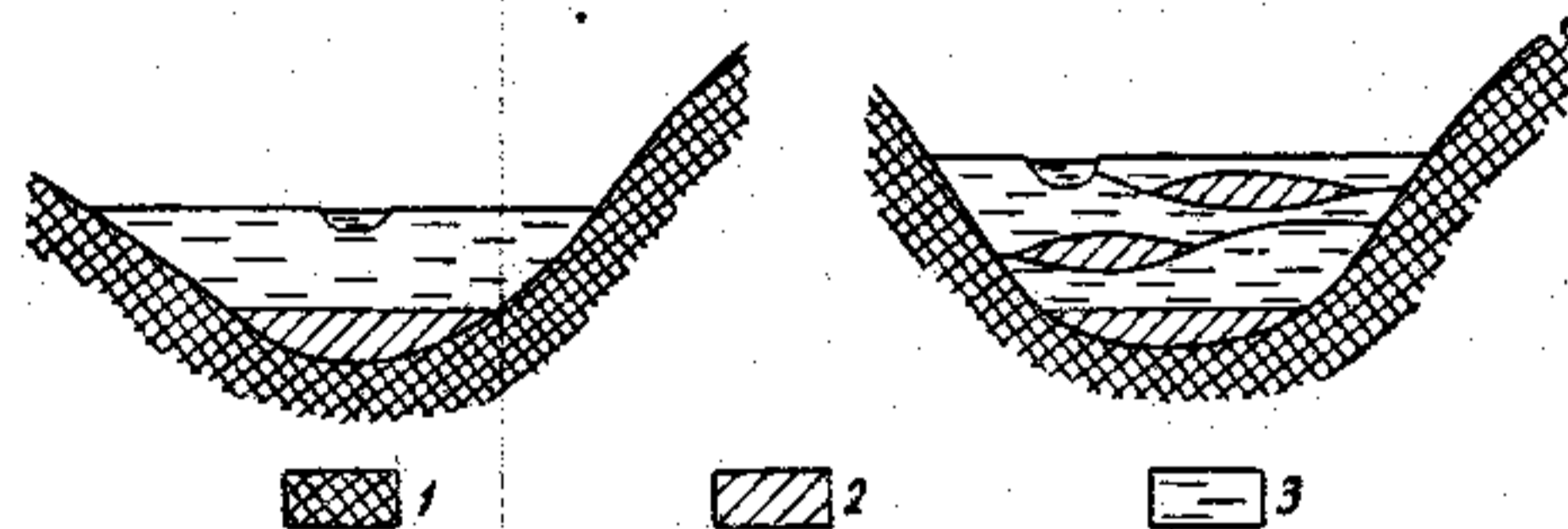
Рис. 4. Простая и сложная россыпи. 1—коренные породы; 2—пласт; 3—торфа.
