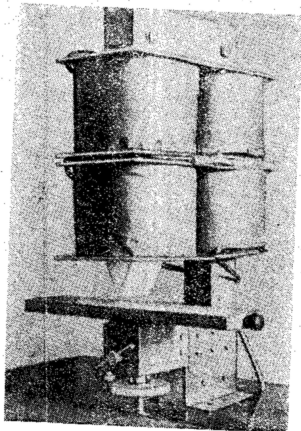
Рис. 23. Простой электромагнит.
