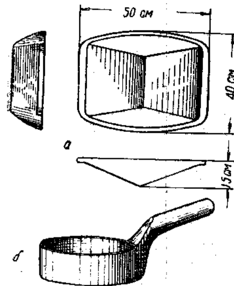
Рис. 11. а — деревянный лоток; б — азиатский ковш.
