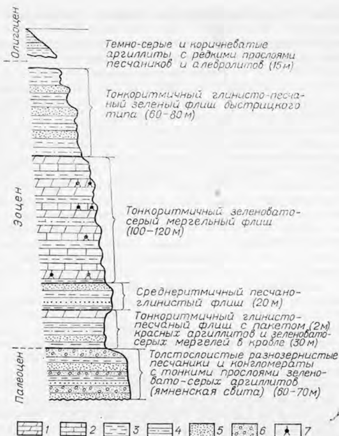
Схематический разрез палеогена в окр. с. Воля Коблянская.
