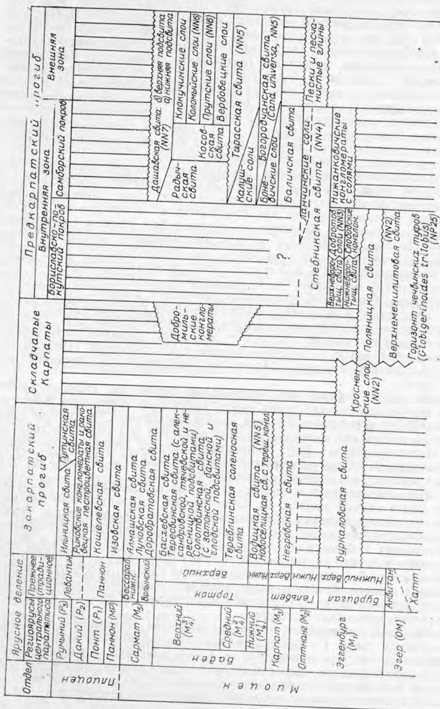
Рис. 1. Стратиграфическая схема неогена Закарпатского и Предкарпатского прогибов и Складчатых Карпат.
