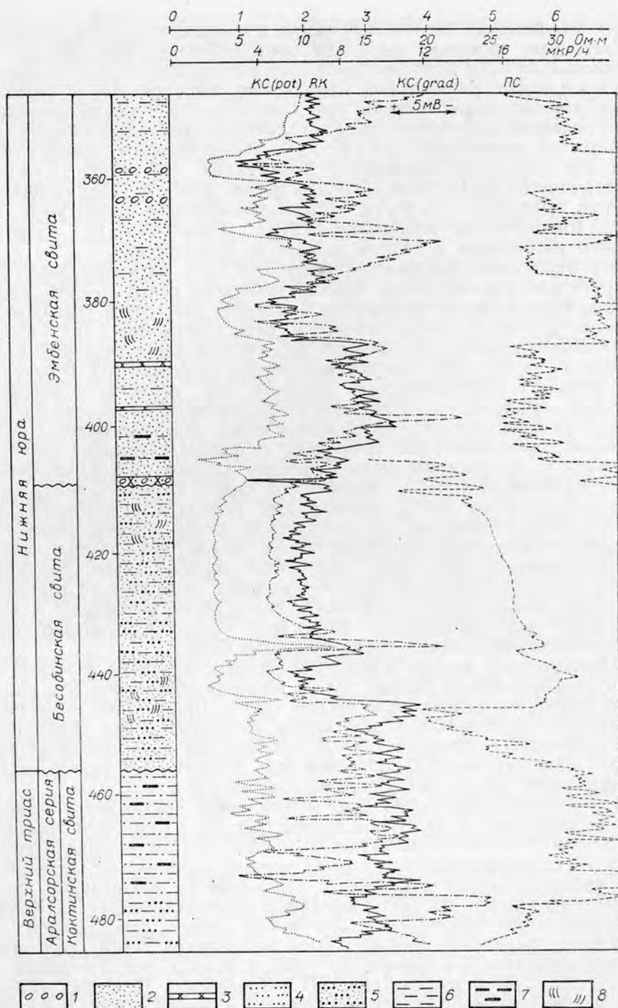
Рис. 1. Стратотипический разрез бесобинской свиты в скважине 3-Бесобе. 1 — галька; 2 — песок; 3 — песчаник; 4 — алевролит; 5 — алевролит опесчаненный; 6 — глина; 7 — углистые прослои; 8 — косая слоистость.
