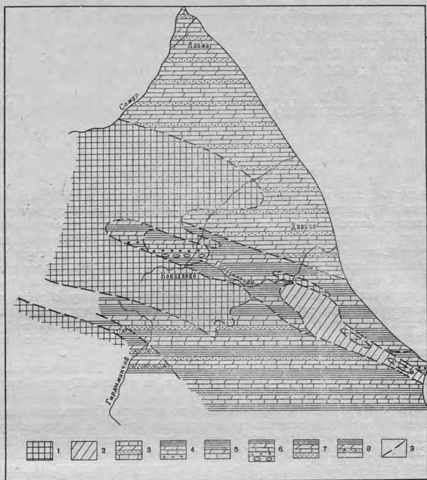
Рис. 1. Литолого-фациальная карта сantonских отложений юго-востока Большого Кавказа
