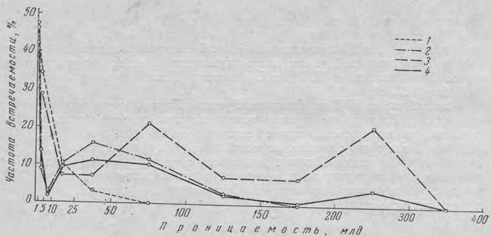
Рис. 4. Вариационные кривые распределения проницаемости песчано-алевролитовых пород:
