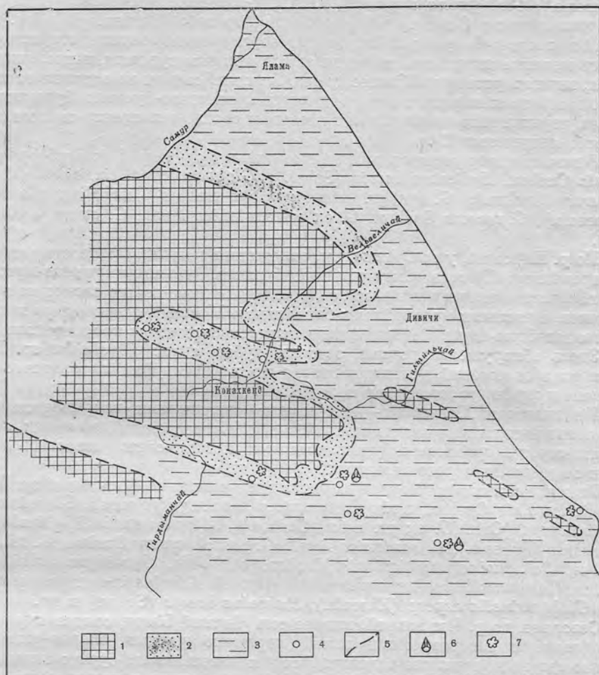
Рис. 3. Палеогеографическая схема юго-востока Большого Кавказа в сantonское время.
