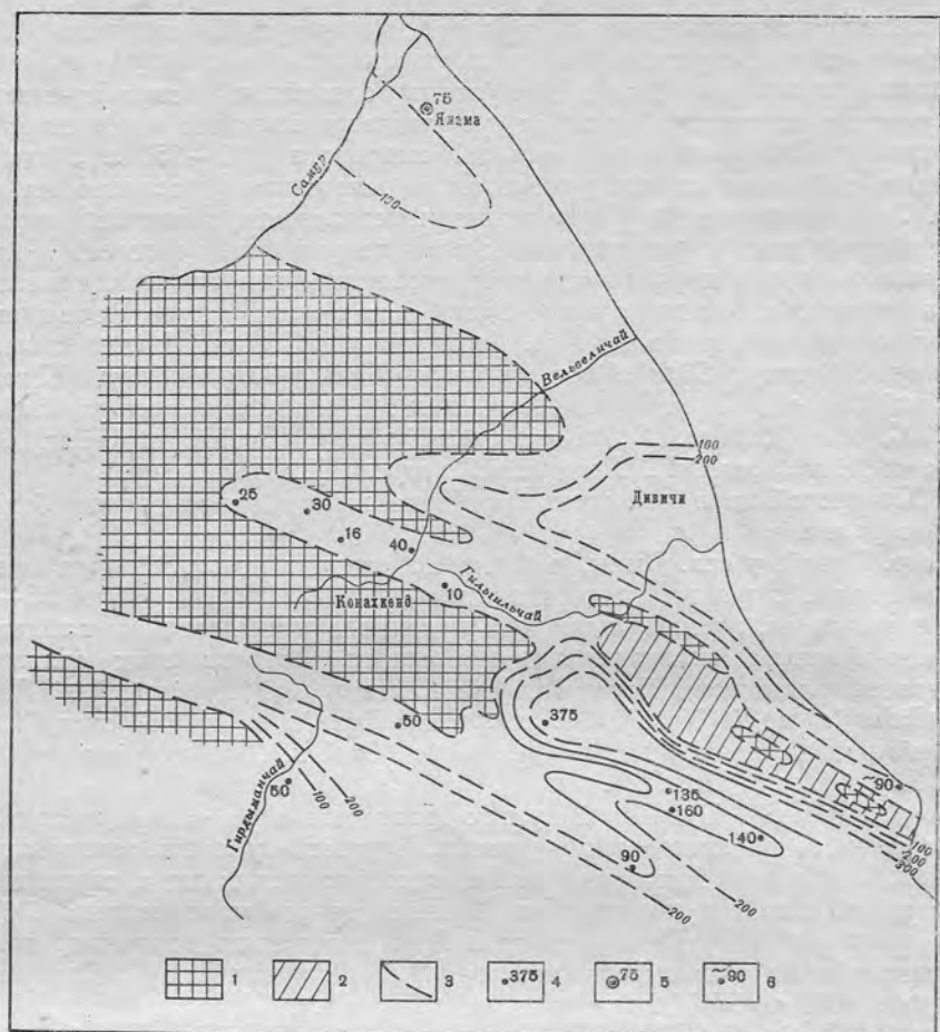
Рис. 2. Карта мощностей сантонских отложений юго-востока Большого Кавказа.
