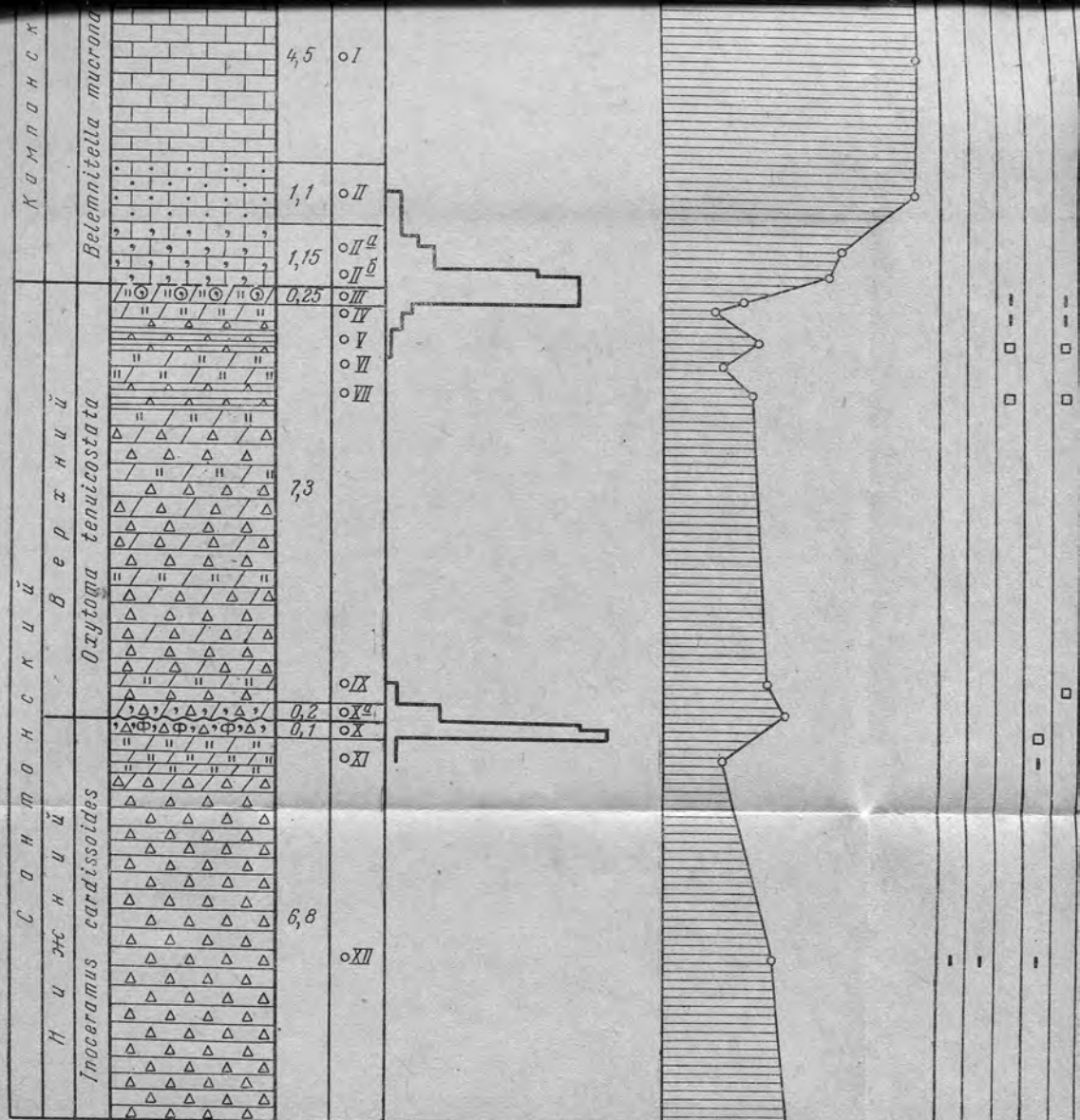
Рис. 1. Литолого-стратиграфический разрез верхнемеловых отложений.
