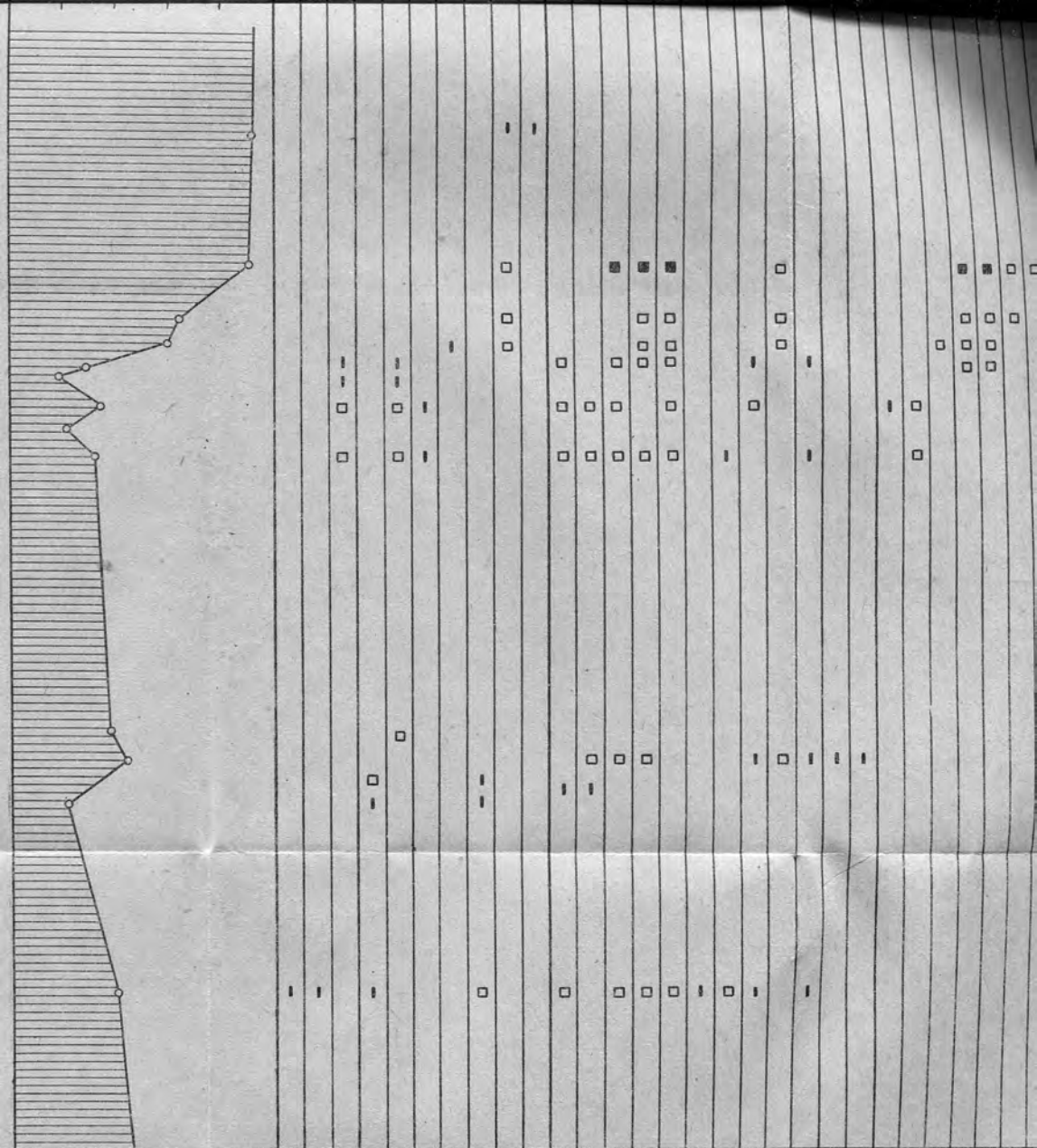
Литографический разрез верхнемеловых отложений у с. Языково (масштаб 1 : 100).
