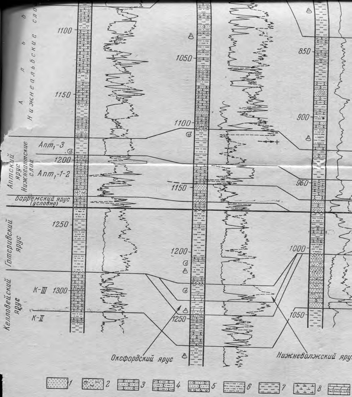
Рис. 1. Сопоставление разрезов нижнемеловых отложений северной части Астраханского 1 — пески; 2 — пески глинистые; 3 — песчаники, алевролиты; 4 — песчаники, алевролиты глинистые; 5 — глины; 6 — глины известковистые; 7 — карбонатные породы; 8 — макрофауна; 9 — фораминиферы; 10 — фораминиферы; 11 — фораминиферы
