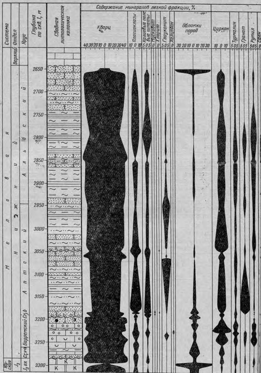
Рис. 2. Диаграмма изменений минералогического состава нерастворимого остатка Условные обозначения см. на рис. 1
