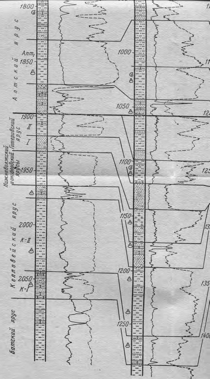
Рис. 2. Сопоставление разрезов нижнемеловых отложений Астраханского Условные обозначения см. на рис. 1
