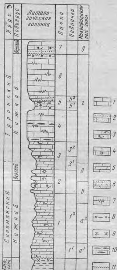
Рис. 1. Сводный разрез сеноман-нижнетуронских отложений Дагестана.
