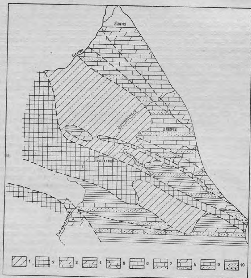
Рис. 2. Литолого-фациальная карта верхнемаастрихтских отложений юго-востока Большого Кавказа.
