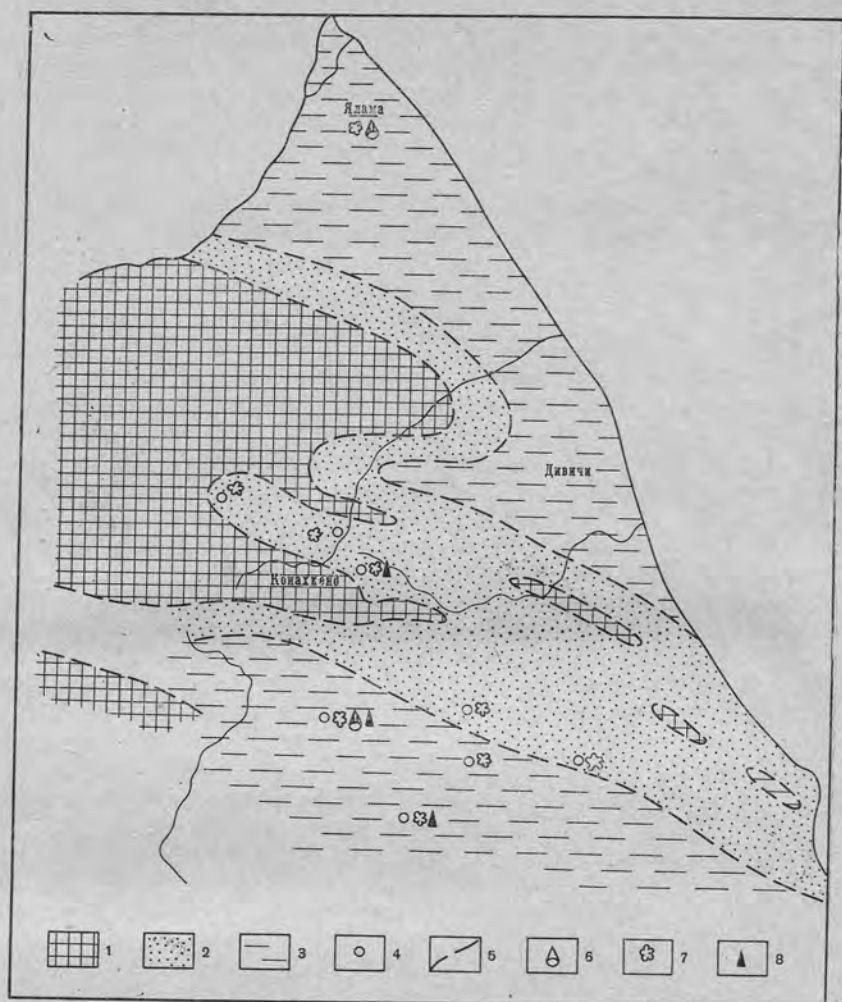
Рис. 3. Палеогеографическая схема юго-востока Большого Кавказа в верхнетуронское — коньякское время.
