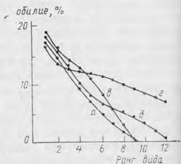
Рис. 25. Кривые доминирования для выборок разного размера а — 1 см², б — 16 см², в — 0,25 м², г — 12,5 м²
