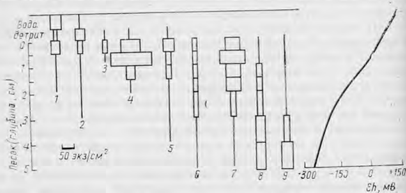
Рис. 32. Вертикальное распределение инфузорий в толще грунта. Виды: 1 — Strombidium sulcatum , 2 — Pleuronema coronata , 3 — Diophris scutum , 4 — Remanella margaritifera , 5 — Trachelostyla pediculiformis , 6 — Cardiostomatella vermiforme , 7 — Tracheloraphis incaudatus , 8 — Kentrophorus fasciolatus , 9 — Urostrongylus caudatus
