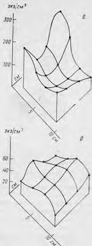
Рис. 22. Размещение диатомовых водорослей (а) и фитомастигин (б) на площади 100 см²
