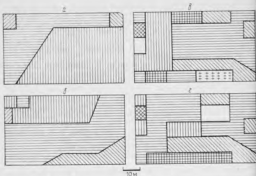
Рис. 17. Структурное разнообразие сообщества на уровнях микро-, мейо- и макро-бентоса (схема). Тип штриховки соответствует определенной структуре доминирования в микро-, мейо- и макро-бентосе, выявленной кластерным анализом: а — макро-бентос, б — мейо-бентос, в, г — микро-бентос (съемки проведены с интервалом 14 сут). Исследованная площадь — 3200 м, 25 станций (см. рис. 1, Б)
