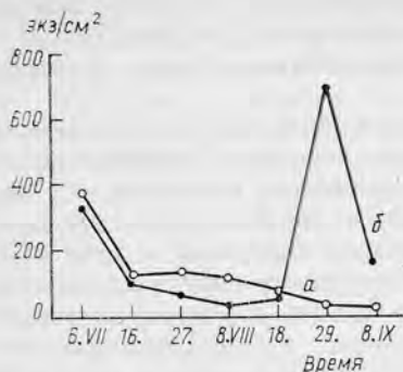
Рис. 54. Реакция морских инфузорий на понижение солености (до 4‰) и окисленности среды в отсутствие инородного биоценотического окружения.
