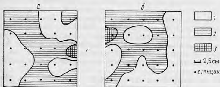
Рис. 29. Размещение инфузории Tracheloraphis incaudatus (а) и ее основного пищевого объекта диатомовой водоросли Gyrosigma recta (б) на площадке 625 м 2 (по Бурковскому, 1984).
