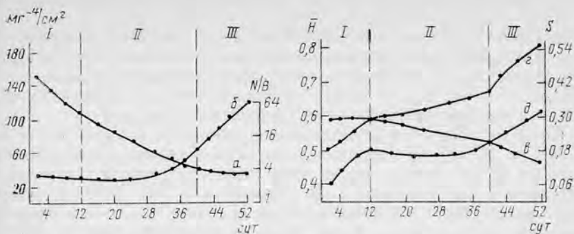
Рис. 56. Изменение некоторых структурных характеристик сообщества инфузорий в лабораторном эксперименте. а — общая биомасса инфузорий, \text{мг}^{-4}/\text{см}^2 , б — отношение численности к биомассе ( N/B ), в — трофическое разнообразие ( \bar{H} , в долях от максимально возможного), г — видовое разнообразие (то же), д — скорость сукцессии ( S , безразмерная величина). I—III комплексы видов (пояснение в тексте)
