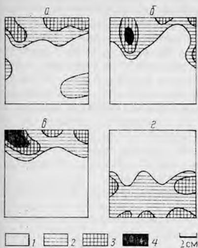
Рис. 30. Размещение организмов микробентоса на площади 100 см 2 . \bar{m} — средняя плотность, экз/см 2 , 1 — меньше \bar{m} , 2 — более \bar{m} , 3 — более 2 \bar{m} , 4 — более 3 \bar{m} . а — Tracheloraphis incaudatus , m=51 , б — Histiobalanium majus , H. marinum , m=10,1 , в — фито- и зоомастигины, m=700 , г — Uronychia transfuga , \bar{m}=116
