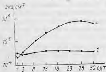
Рис. 57. Влияние нефтяных углеводов на общую плотность диатомовых водорослей.
