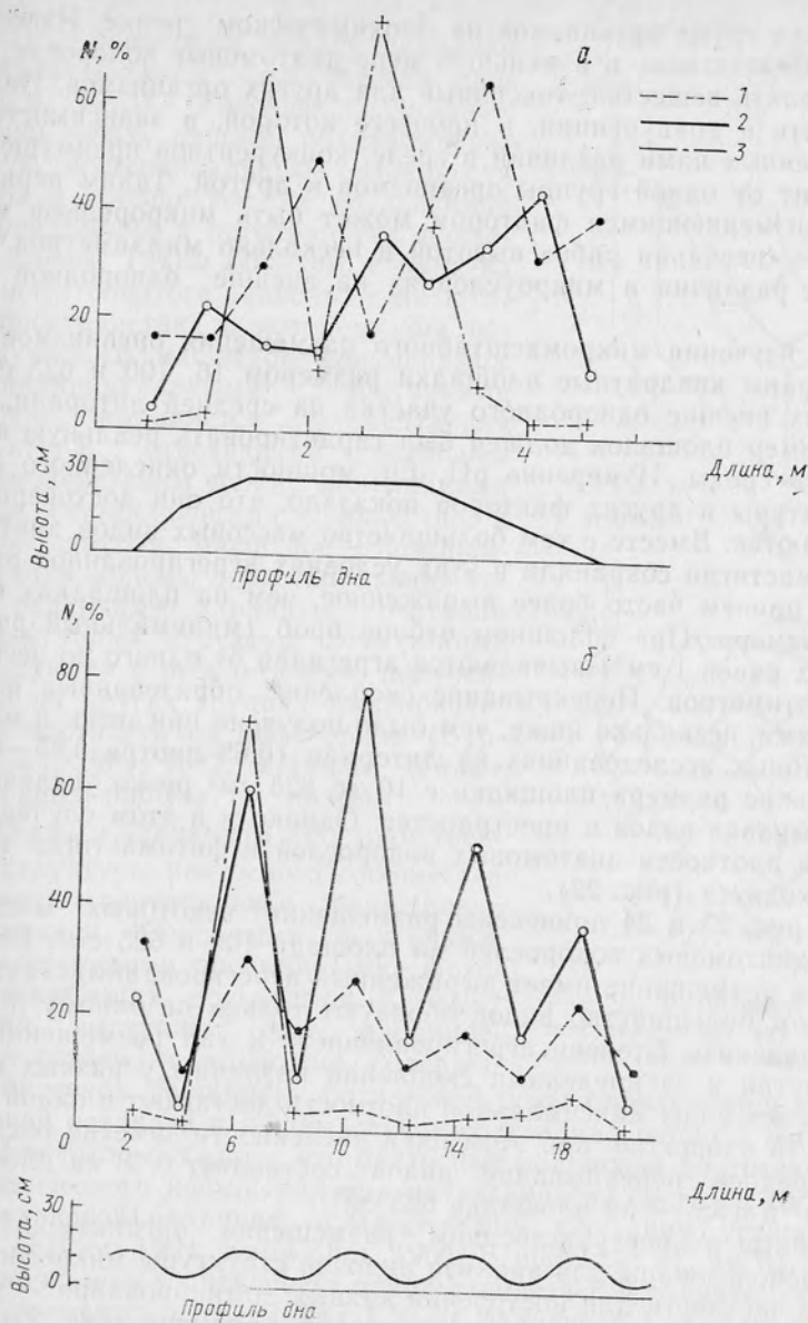
Рис. 21. Размещение микрофитобентоса на продольной (а) и поперечной (б) транsekтах. 1 — диатомовые водоросли, 2 — мелкие фитомасстигины, 3 — крупные фитомасстигины
