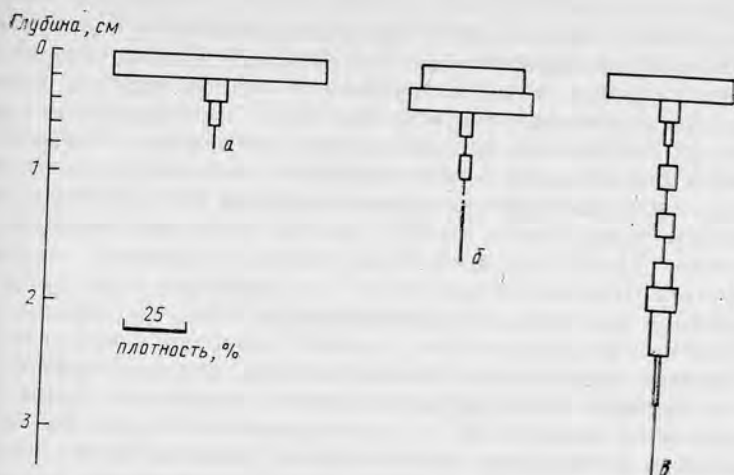
Рис. 26. Вертикальное распределение микрофитобентоса.
