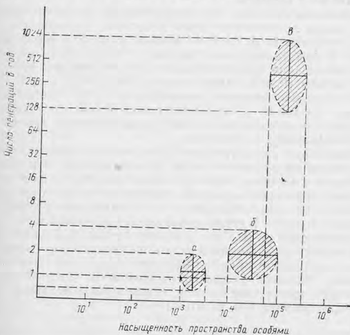
Рис. 18. Насыщенность «биологического» пространства и времени для макробентоса (а), нематод (б) и инфузорий (в). Объяснения в тексте
