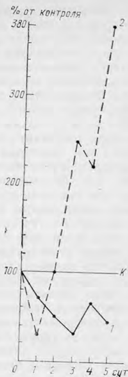
Рис. 59. Реакция Tracheilographis incaudatus (1) и Tg. phoenicopterus (2) на внесение меди (10 мг/л). К — контроль
