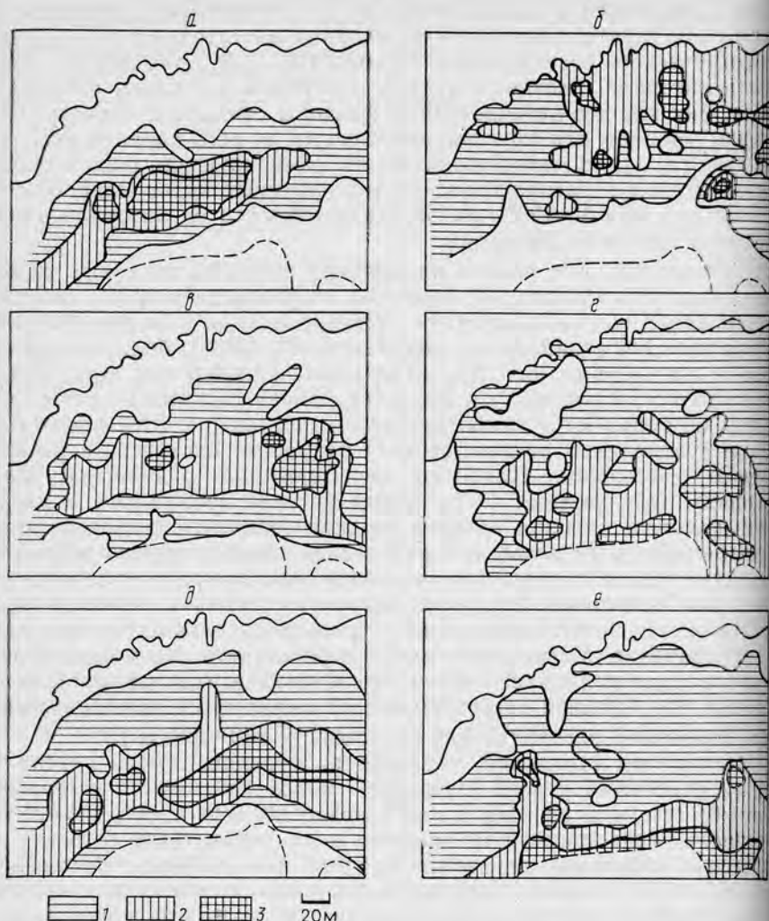
Рис. 44. Распределение массовых видов макробентоса на литорали в губе Грыбной.
