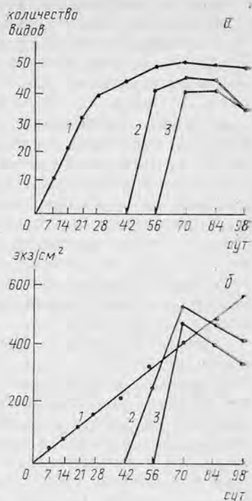
Рис. 51. Скорость колонизации у инфузорий на разных стадиях сезонной сукцессии. а — изменение видового богатства, б — изменение плотности.
