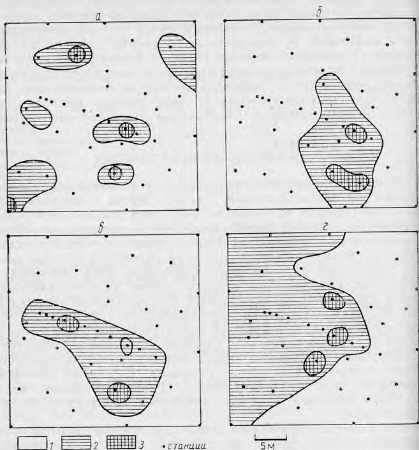
Рис. 28. Размещение инфузорий на площади 1000 м 2 (по Бурковскому, 1984). \bar{m} — средняя плотность, экз/см 2 , 1 — менее \bar{m} , 2 — более \bar{m} , 3 — более 2 \bar{m} . а — Uronema marina , \bar{m}=121,2 , б — Oxytricha discifera , \bar{m}=75,6 , в — Remanella margaritifera , \bar{m}=61,0 , г — Tracheloraphis incaudatus , \bar{m}=52,1 .
