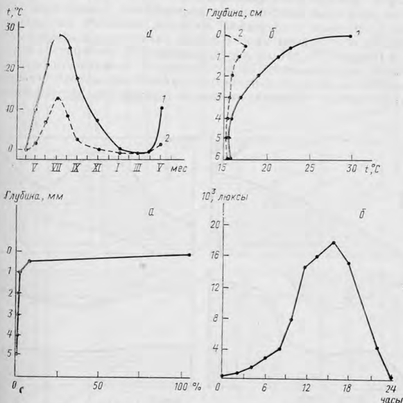
Рис. 10. Изменение температуры грунта на литорали: а — на поверхности в течение года, б — в толще грунта (в июле). 1 — максимальная, 2 — минимальная
