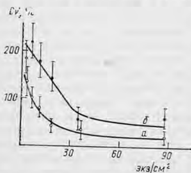
Рис. 40. Влияние плотности (экз/см 2 ) лидирующего вида Tracheloraphis incaudatus на колебания общей плотности ( CV , %) эвритопных (а) и интерстициальных (б) видов (по Бурковскому, Азовскому, 1985)
