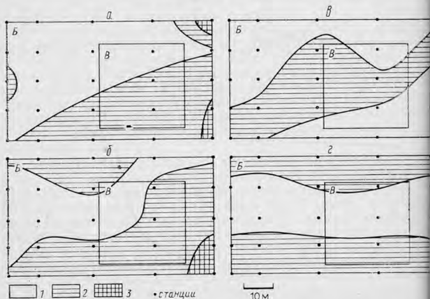
Рис. 12. Распределение пелита (а, ‰ от веса осадка), C_{орг} (б, ‰ от веса осадка), кислорода (в, ‰ от 100‰ насыщения) и редокс-потенциала (г, мВ). \bar{m} — среднее, \bar{m}_a=2,18 , \bar{m}_б=4,8 , \bar{m}_в=37,9 , \bar{m}_г=164 . Б и В — то же, что на рис. 1 1 — менее \bar{m} , 2 — более \bar{m} , 3 — более 2\bar{m} .
