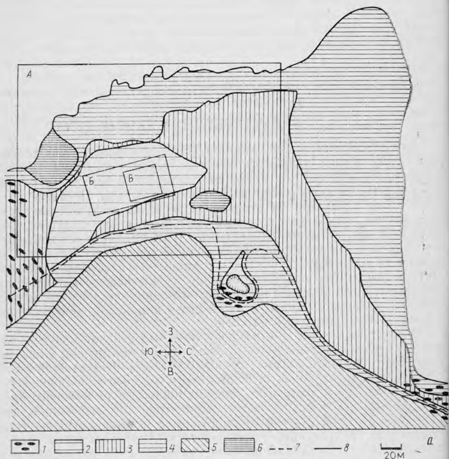
Рис. 1. Распределение грунтов (а) и макрофитов (б) в губе Грязной средним содержанием алевропелита, 4 — песок с высоким содержанием алевро- бина, 8 б: 1 — Puccinellia sp., Triglochia maritima , Glaux maritima , Aster tripolium , maritima , 4 — Zostera marina , 5 — Fucus serratus , 6 — редко: Chorda filum , Площади, ограниченные прямоугольниками А, Б, В, представляют разные мас-
