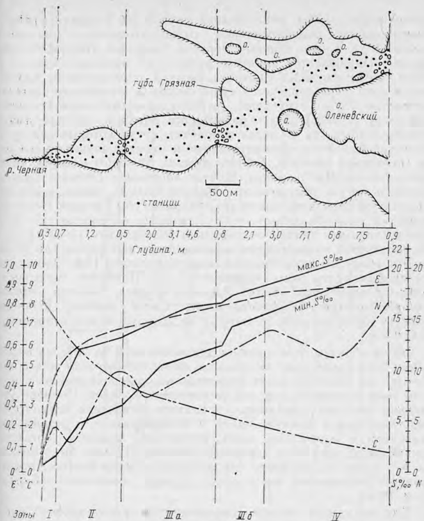
Рис. 46. Изменение видового богатства ( N ), выравненности ( \epsilon ) и доминирования ( C ) в зависимости от солености воды ( S_{\text{‰}} ) и глубины эстуария р. Черной. I—IV — зоны. Объяснение в тексте
