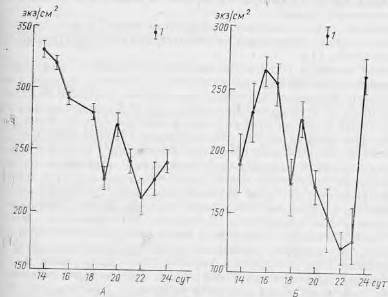
Рис. 36. Изменение плотности локальных популяций инфузорий в течение 10 сут: а — Discocephalus rotatorius , б — Aspidisca irinae , 1 — 95%-ный доверительный интервал
