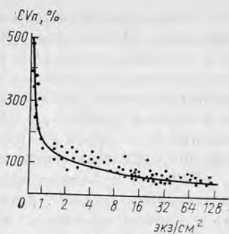
Рис. 35. Зависимость коэффициента вариации плотности ( CV_{\pi} ) инфузорий от абсолютных значений плотности, экз/см 2 (по Бурковскому, 1984). Каждая точка на графике обозначает один вид инфузорий
