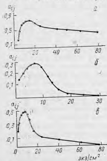
Рис. 41. Зависимость пространственного перекрытия ( a_{ij} ) потенциальных конкурентов от их суммарной плотности (по данным размещений видов в трехмерном пространстве, в объеме 30 см 3 )
