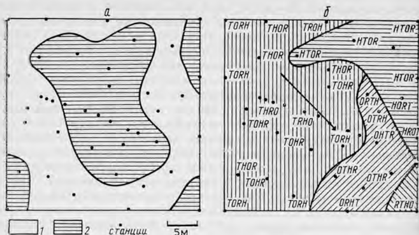
Рис. 34. Пространственная структура сообщества инфузорий (по Бурковскому, 1978):
