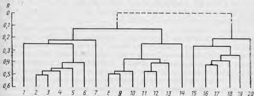
Рис. 43. Кластерный анализ распределения видов макробентоса в губе Грязной (по данным съемки 1989 г.).
