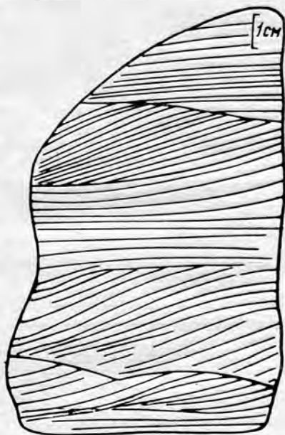
Рис. 15. Выпукло-вогнутая (S-образная) форма слоев в продольном сечении серий морского происхождения. Верхн. талаканской свиты нижнего протерозоя, левый борт кл. Клоквенного. Зарисовка по фотографии В. П. Феоктистова.
