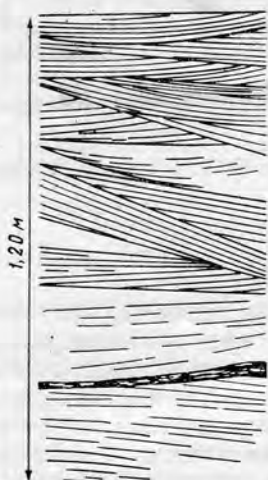
Рис. 37. Косая слоистость в отложениях подводной части дельты (по Л. Н. Ботвинкиной, 1962). Донбасс, свита S_2^3 (зарисовка А. П. Феофиловой).
