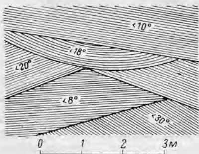
Рис. 71. Косая эоловая слоистость (по С. Н. Колову, 1952).
