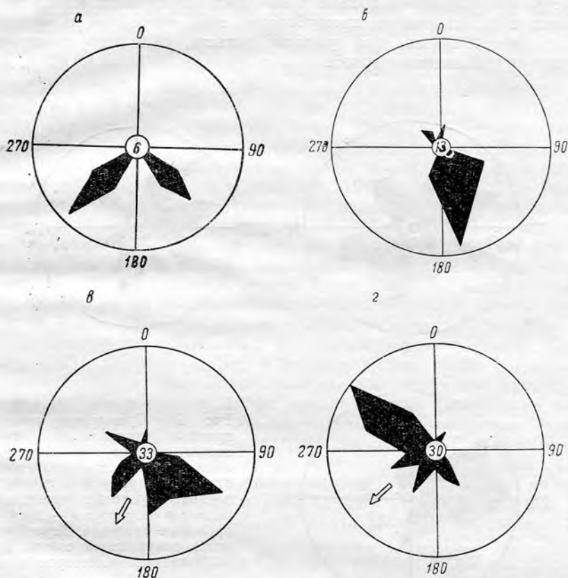
Рис. 27. Розы-диаграммы направлений наклона косых слоёв: а, б — косослоистых песчаников отелей и стрежней в турамской свите верхнего кембрия (р. Иркинеева), диаграмма а построена по замерам в одной вогнутой косослоистой серии; в — главным образом подводно-русловых отелей дельты; г — подводно-русловых протоков дельты (верхняя подсвита сакуканской свиты, район Удоканского месторождения).
