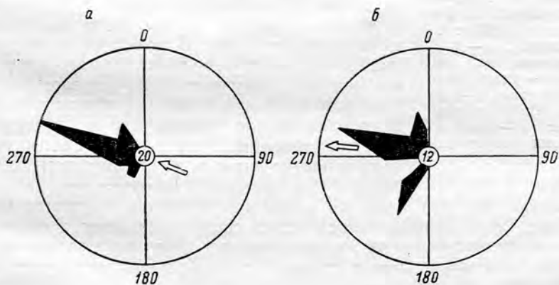
Рис. 20. Розы-диаграммы направлений наклона косых слоев известковистых песчаников подводно-русловых протоков (стрешней): a — с прямолинейными косыми слоями; б — с вогнутыми косыми слоями. Верхняя подсвита сакуканской свиты, район Удоканского месторождения. Стрелкой показано предполагаемое направление потока. Здесь и далее в кружках — количество замеров.
