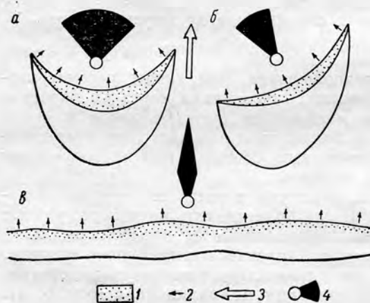
Рис. 7. Типичная форма гряд. а, б — серповидные гряды: а — симметричная, б — асимметричная; в — прямолинейная гряда, ориентированная нормально к течению, показанному стрелкой.
