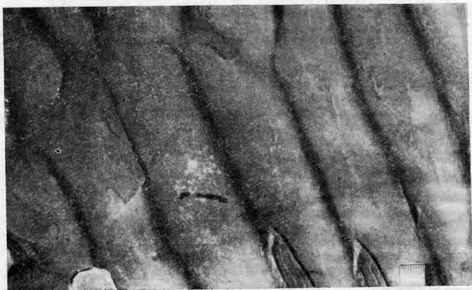
Рис. 6. Асимметричные знаки ряби течения (гряды) на поверхности напластования алевропесчаника, хорошо сохранившиеся при перекрытии их тонкозернистым материалом. Сакуканская свита, район Удоканского месторождения. Колл. Ю. В. Богданова.
