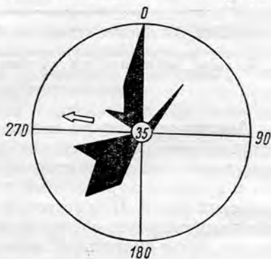
Рис. 41. Роза-диаграмма направлений наклона косых слоев песчаников прирусловых кос подводной дельты.
