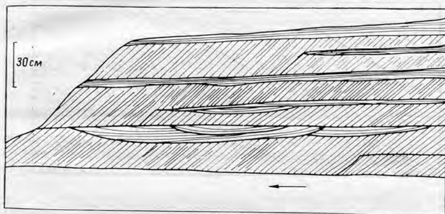
Рис. 32. Характер косой слоистости в песках конуса выноса небольшой речки, впадающей в Подкаменную Тунгуску.
