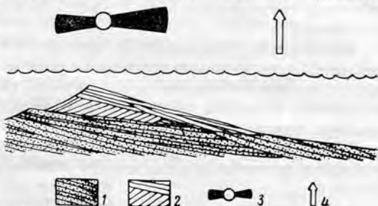
Рис. 47. Схема прируслового вала (поперечное сечение).
