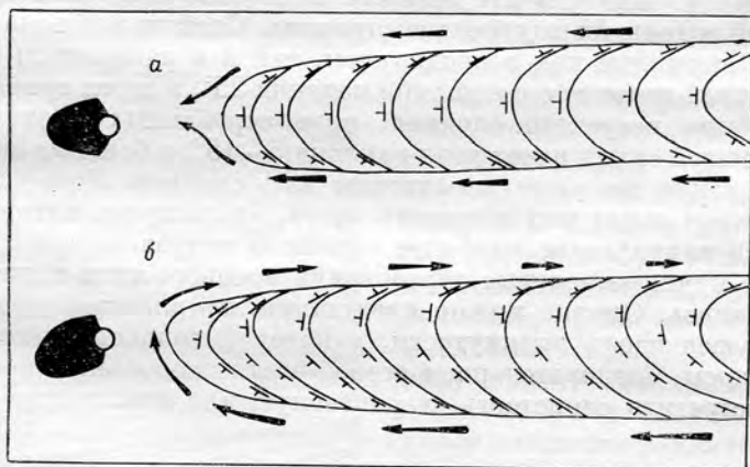
Рис. 46. Схема механизма формирования симметричных кос (стрелок). а — коса наращивается двумя потоками; б — коса наращивается одним, огибающим потоком.
