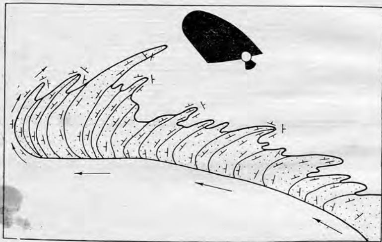
Рис. 42. Схема механизма формирования асимметричной косы.
