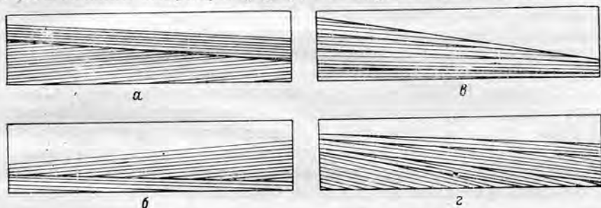
Рис. 59. Типы косой слоистости бычей.
