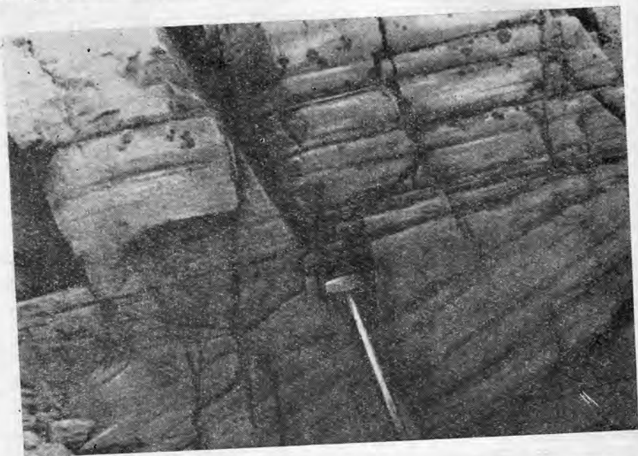
Рис. 60. Очень крупная согласная косая слоистость подводного вала. Нижняя подсвита сакуканской свиты, кл. Скользкий. Фото В. П. Феоктистова.
