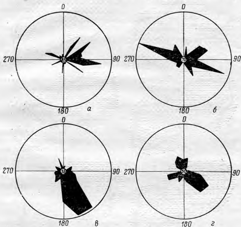
Рис. 63. Розы-диаграммы направлений наклона косых слоев: а — бары-косы, северное крыло Намингинской брахисинклинали; б — совмещенная диаграмма баровых (правая половина) и подводно-русловых (левая половина) песчаников, юго-западная часть брахисинклинали; в, г — песчаников мористой стороны бара, восточное замыкание брахисинклинали. Верхняя подсвита сакуканской свиты, район Удоканского месторождения.
