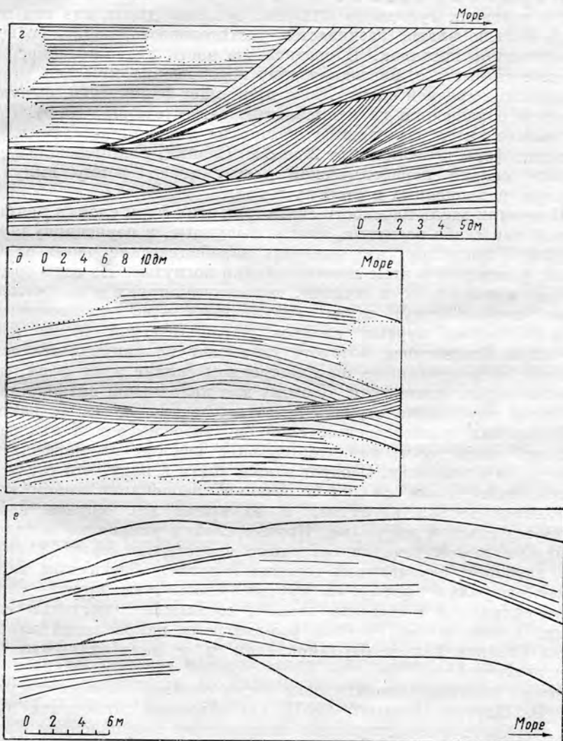
Рис. 30. Зарисовка типов косой слоистости в песках верхней части поперечной дюны высотой около 8 м. Рижский залив, г. Юрмала, Лиелупэ.
