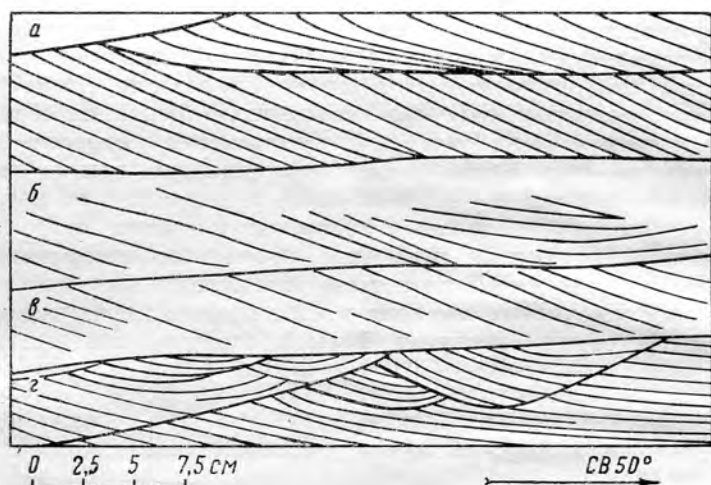
Рис. 3. Продольный разрез нормальной грядной косой слоистости (а—г) и нескольких мульдобразных косослоистых серий (г) с выполаживающимися слойками, образованных, по нашему мнению, путем выполнения подвалев гряд при падении скорости потока ниже грядообразовательной. Илгинская свита верхнего кембрия, р. Лена.
