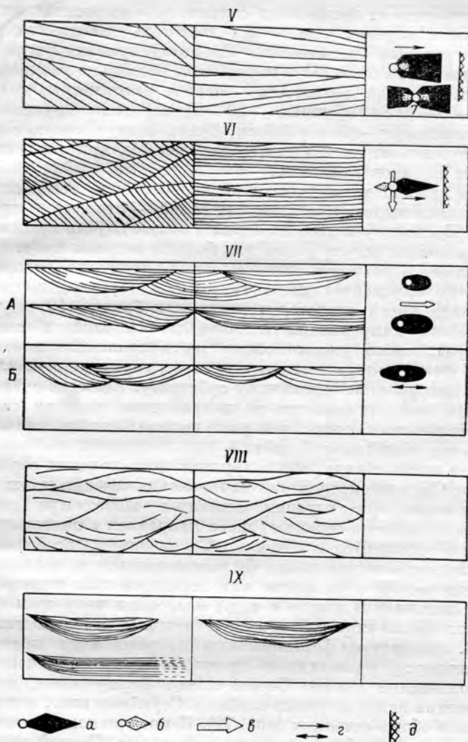
Рис. 72. Морфологические типы косой слоистости.
