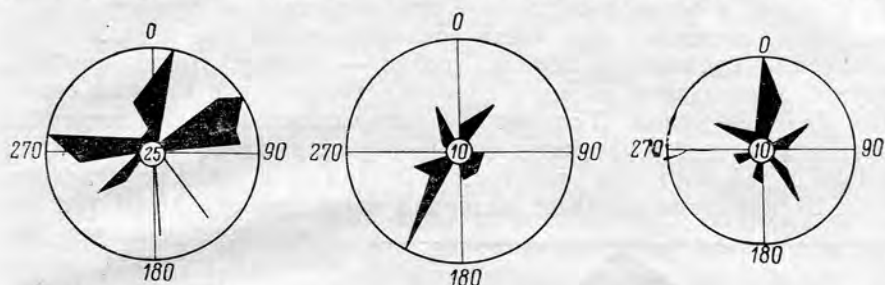
Рис. 56. Суммарные диаграммы, характеризующие недифференцированные (грядные и гривневые) отложения донных морских течений. О направлении течений по таким диаграммам ничего определенного сказать нельзя. Сакуканская свита, район Удоканского месторождения.
