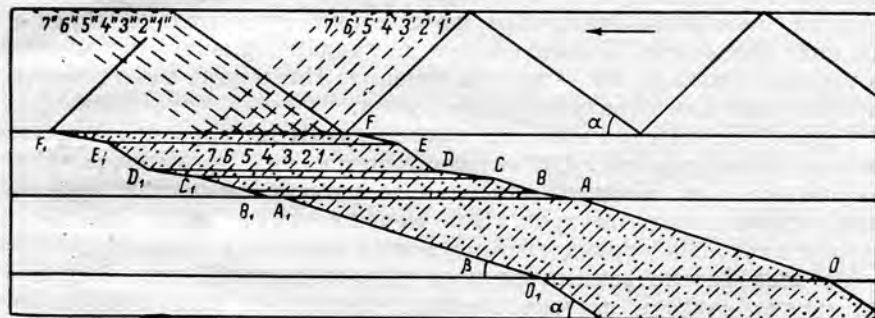
Рис. 34. Схема образования косослоистой серии (пунктир с точками) при движении гряды.
