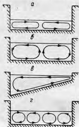
Рис. 21. Схема четырех типов поперечной циркуляции воды в русловом потоке и их зависимость от формы поперечного сечения и глубины русла (по А. И. Лосиевскому, 1934, с изменениями). а — расходящиеся по дну токи; б — сходящиеся по дну токи; в — односторонняя циркуляция; г — смешанный тип (сдвоенный тип а).
