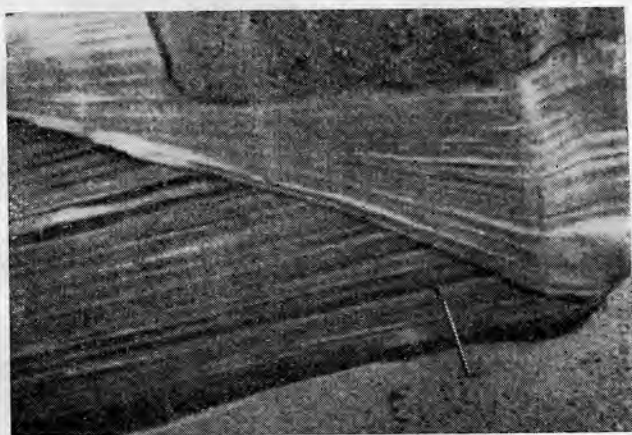
Рис. 61. Характер сочленения двух косослоистых серий подводного вала. Четвертичные отложения. Ленинград, Сосновский парк.
