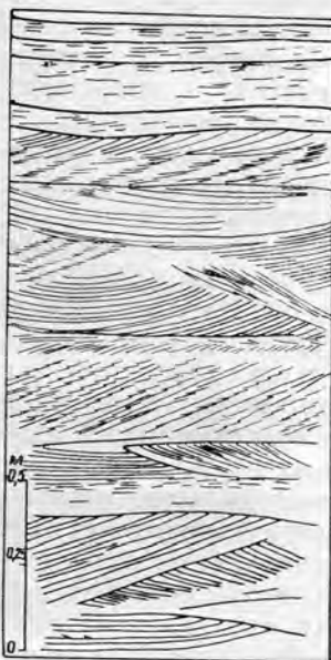
Рис. 50. Косая слоистость в верхней части русловых отложений на левом берегу р. Дона у хут. Кривского (по Л. Н. Ботвинкиной, 1962).
