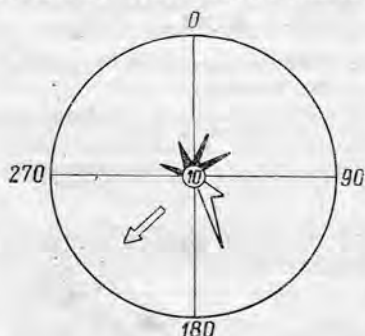
Рис. 49. Диаграмма направлений наклона косых слоев песчаников прируслового вала.
