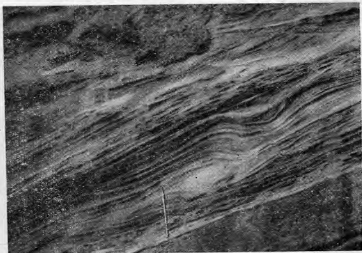
Рис. 62. Знаки оползания и усложнение однонаправленной косой слоистости подводного вала мелкими косослоистыми сериями, что совершенно нехарактерно для грядного типа косой слоистости. Четвертичные отложения. Ленинград, Сосновский парк.
