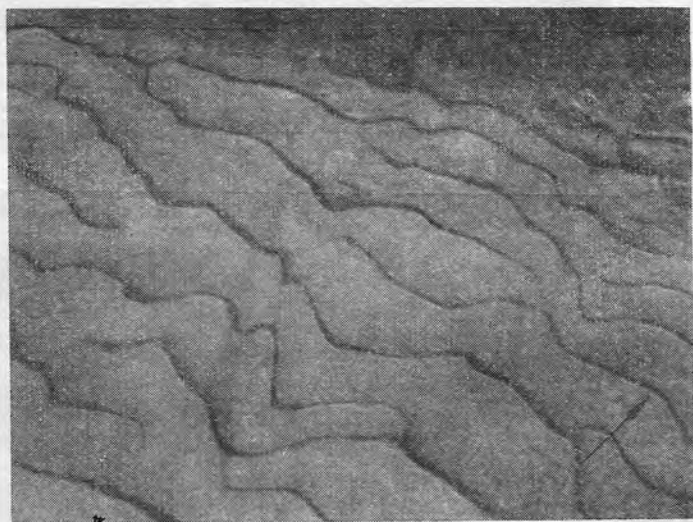
Рис. 11. Выпукло-вогнутая форма гряд в плане. Русло р. Ангары в нижнем течении.
