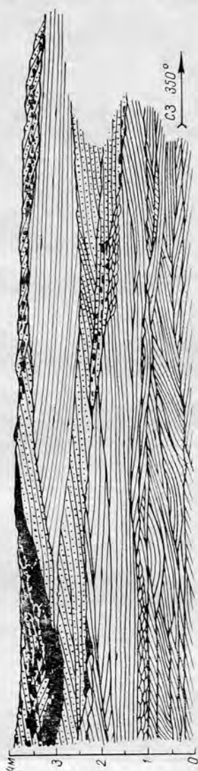
Рис. 38. Зарисовка косой слоистости песчанков приустьевых кос, переслаивающихся с известковыми песчанками подводно-руслых протоков (показано крапом). Черные — катипи аргиллита. Сечение примерно перпендикулярно к направлению палеотечения. Сакуканская свита, район Удоканского месторождения.
