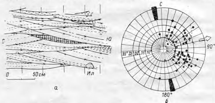
Рис. 26. Косая слоистость в третичных дельтовых отложениях Японии (по Канэко Сиро, 1958). a — зарисовка обнажения, разбитого по сетке для замеров (крестиками показаны точки замеров; заштрихована одна косослоистая серия); б — полярная диаграмма направлений и углов наклона косых слоев и серийных швов.
