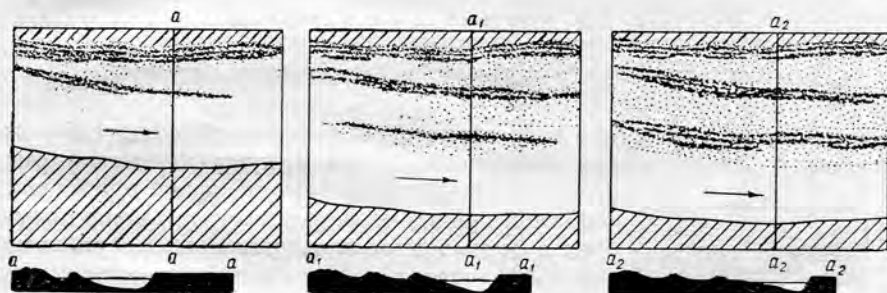
Рис. 35. Схема, иллюстрирующая «скачкообразное» нарастание прирусловых отелей и происхождение крупногрядного рельефа (по Е. В. Шанцеру, 1951).
