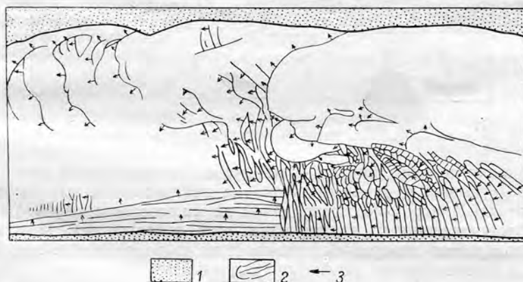
Рис. 23. Схема одного из небольших перекатов на верхней Оке. (Рисунок по аэроснимку А. К. Пронина из книги Е. В. Шанцера [1951]).
