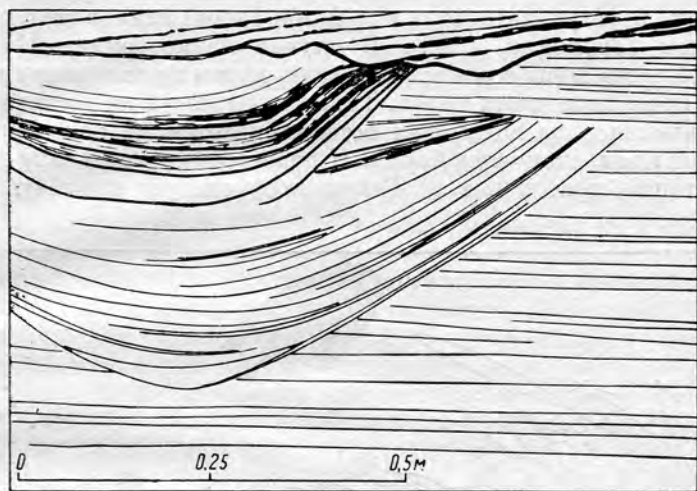
Рис. 40. Косослойный песчаник косы с промоинами, выполненными наносами, обогащенными «естественным шпихом» (толстые черные слойки). Сакуканская свита, район Удоканского месторождения.
