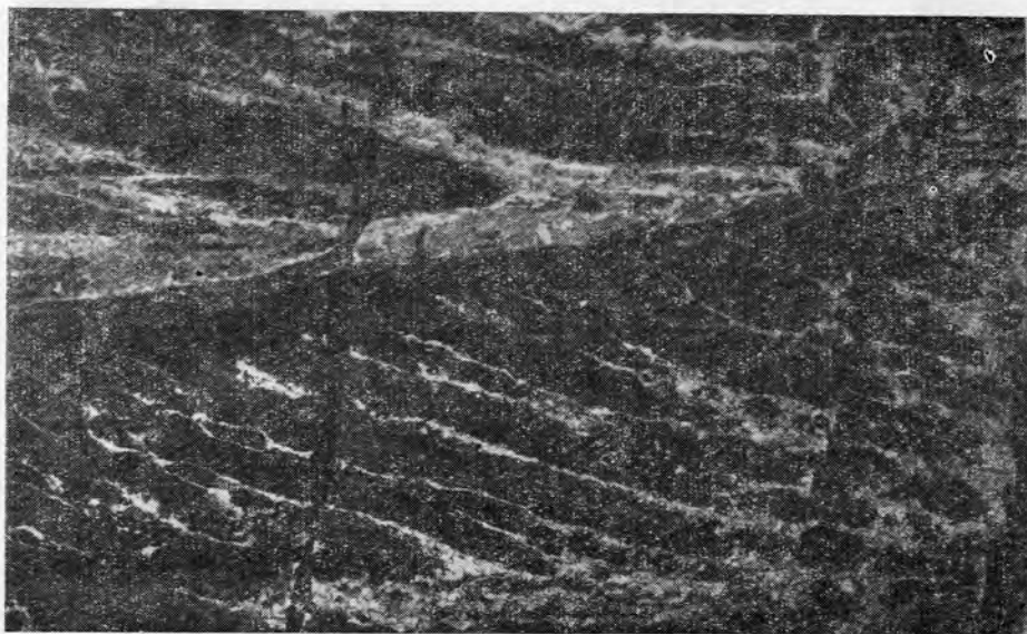
Рис. 19. Фрагмент двух косослоистых серий известковистого песчаника подводно-русловой протоки. Верхняя подсвита сакуканской свиты, район Удоканского месторождения. Фото Ю. В. Богданова.
