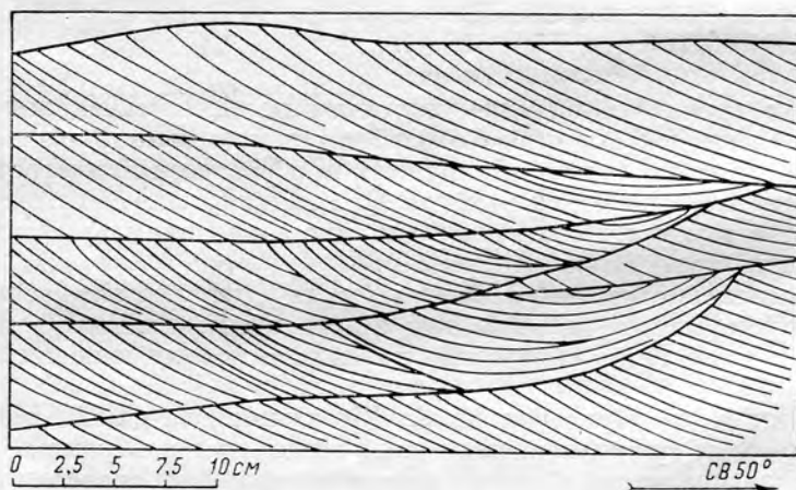
Рис. 4. Мульдобразная косая слоистость выполнения подвалев гряд, сочетающаяся с нормальной грядной косой слоистостью. Илгинская свита, р. Лена.
