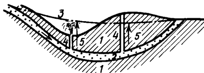
Рис. 5.3. Схема размещения артезианских вод: 1 — водоупорный пласт, 2 — артезианский водоносный горизонт, 3 — линия напора (пьезометрическая линия), 4 — скважины, 5 — высота подъема артезианских вод через скважины
