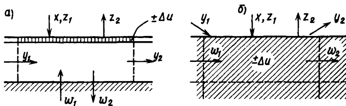
Рис. 2.1. Схема водного баланса части водного объекта a и части поверхностного слоя суши б
