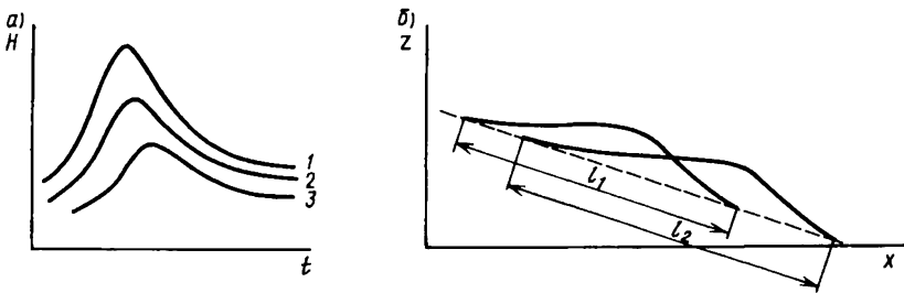
Рис. 6.17 Схема трансформации паводочной волны: а — график изменения уровня воды в трех створах, расположенных последовательно вдоль русла; б — продольные профили паводочной волны и ее длины в два последовательных момента времени
