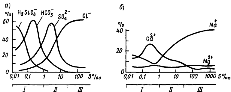
Рис. 1.2. Зависимость содержания главных анионов а и катионов б в солевом составе природных вод (в %) от минерализации (солености) воды по М. Г. Валяшко: воды: I — пресные, II — солоноватые, III — соленые
