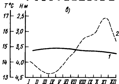
Рис. 5.7. Типичные графики колебания уровня (глубины залегания) 1 и температуры 2 грунтовых вод (по В. С. Ковалевскому): провинции: а — кратковременного питания, б — сезонного питания, в — круглогодичного питания
