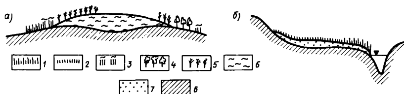
Рис. 9.1. Схема верхового (а) и низинного (б) торфяного болота: микрорельефы: 1 — осоковые, осоково-тростниковые, осоково-гипновые; 2 — сфагново-осоковые; 3 — сфагново-пушицевые; 4 — ольшаники; 5 — сосново-сфагновые; 6 — залежь сфагнового торфа, 7 — залежь тростникового и осокового торфа, 8 — минеральный грунт
