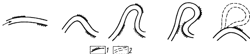
Рис. 6.22. Схема смещения и изменения формы излучины: 1 — участок размыва берега, 2 — старнца
