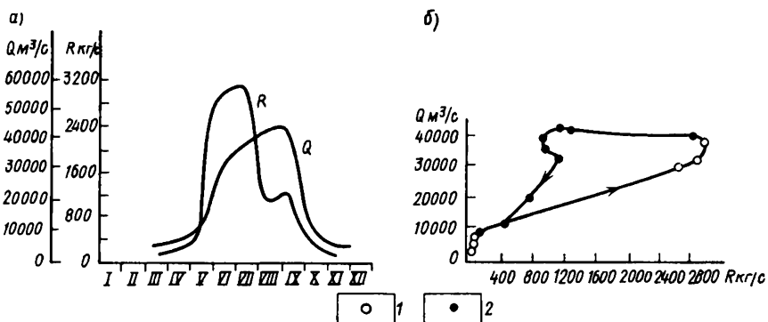
Рис. 6.20. Типичные графики изменения расхода воды и взвешенных наносов а и связи между ними б:
