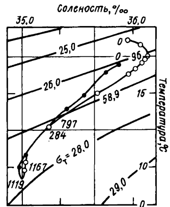
Рис. 10.23. Пример T, S -кривых для двух станций НИС «Атлантик», 1932 г. Цифрами (м) помечены некоторые горизонты
