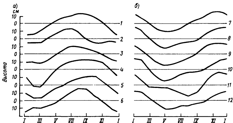
Рис. 10.22. Годовой ход уровня при муссонном (а) и зональном (б) типах циркуляции атмосферы (по Н. И. Егорову): 1 — Балтимор (Чесапикский залив), 2 — Батуми (Черное море), 3 — Шатт-эль-Араб (Персидский залив), 4 — Мергун (Бенгальский залив), 5 — Манила (Филиппинские острова), 6 — Кийру (о. Тайвань), 7 — Печенга (Баренцево море), 8 — Кабелвоч (Норвежское море), 9 — Гриннок (Ирландское море), 10 — Харлиген (Северное море), 11 — Симсон (Канада), 12 — Виктория (Канада)
