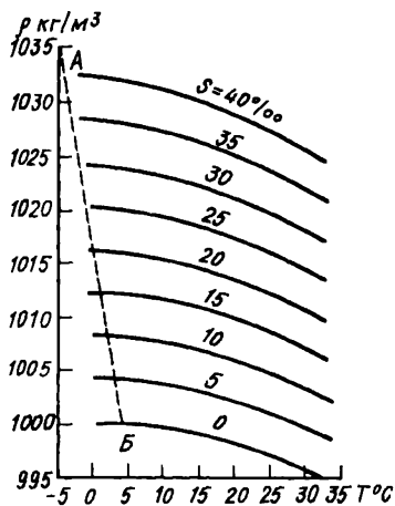
Рис. 1.5. Зависимость плотности воды при нормальном атмосферном давлении от температуры и солёности. AB — линия наибольшей плотности
