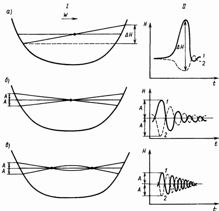
Рис. 7.7. Схема депрессии уровня озера при стонно-нагонных явлениях (а), одноузловой (б) и двухузловой (в) сейшах: I — поперечный разрез, II — колебания уровня у противоположных берегов (1,2) озера
