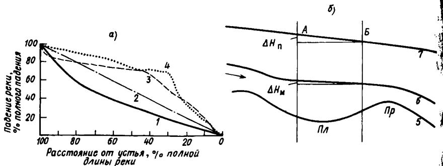
Рис. 6.5. Продольные профили реки a и ее участка б :
