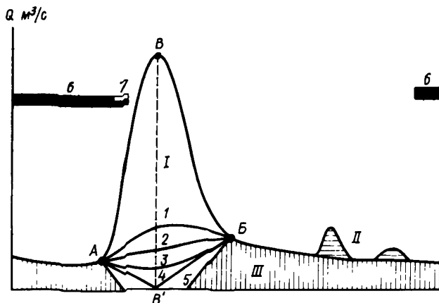
Рис. 6.10 Схема расчленения гидрографа реки по видам питания: питание: I — снеговое, II — дождевое, III — подземное; A, Б и B' — начало, конец и пик половодья; 1—5 — линии, разделяющие снеговое и подземное питание в период половодья при различном характере взаимодействия речных и грунтовых вод (пояснение см. в тексте). 6 — ледостав, 7 — ледоход
