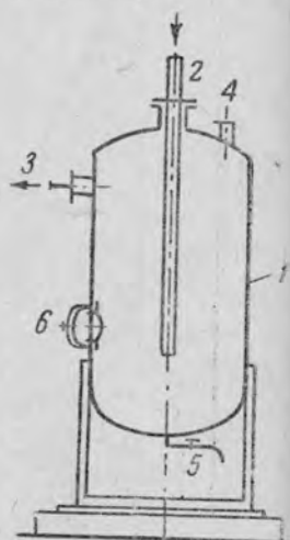
Рис. 49. Ресивер: 1 — ресивер; 2 — воздушная труба от компрессора; 3 — труба к шкатулке управления; 4 — штуцер предохранительного клапана; 5 — отверстие для спуска конденсата; 6 — люк.
